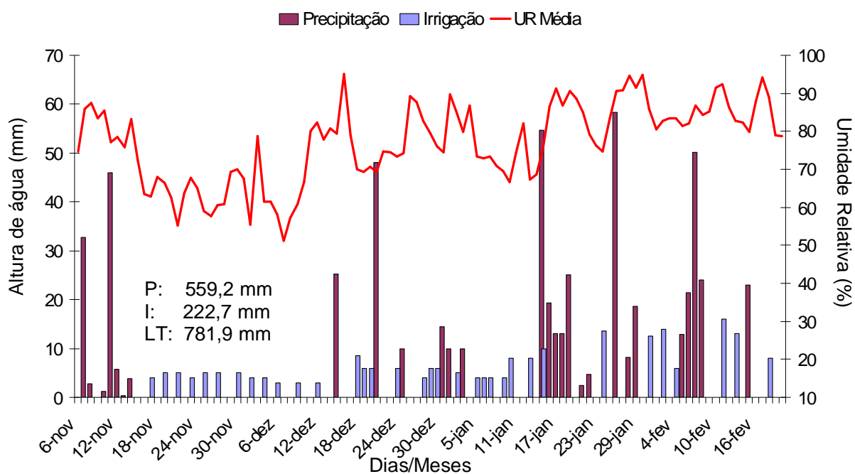
FIGURA 9. Valores diários de precipitação pluvial (mm), irrigação (mm) e umidade relativa (%), observados durante a condução do experimento, para a primeira semeadura em Selvíria – MS.
