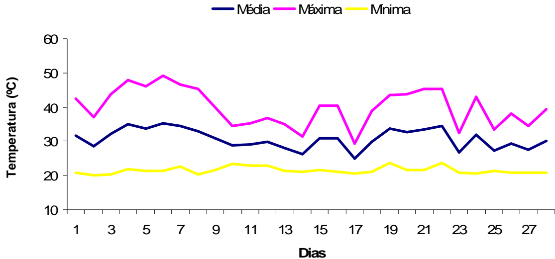
FIGURA 14. Temperatura máxima, mínima e média no mês de fevereiro de 2009. Fernandópolis - SP.
