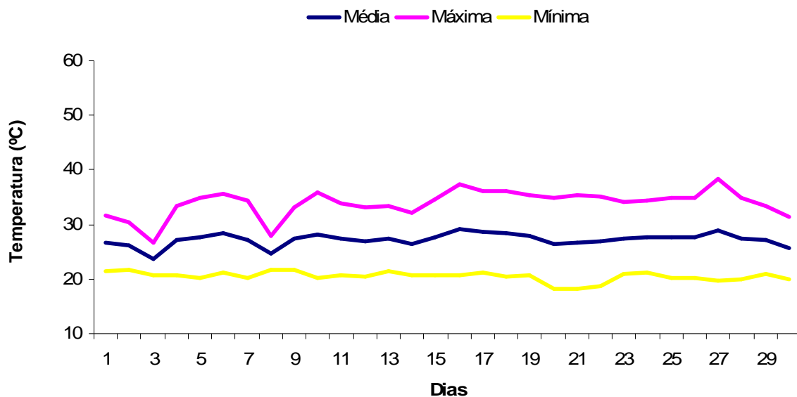
FIGURA 11. Temperatura máxima, mínima e média no mês de novembro de 2008. Fernandópolis – SP.
