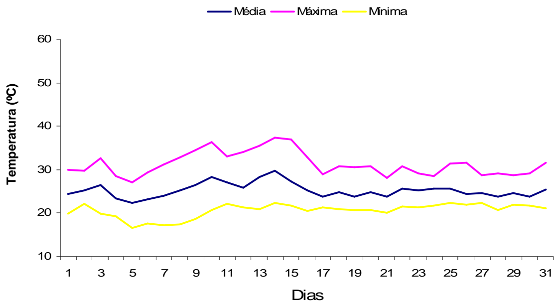
FIGURA 19. Temperatura máxima, mínima e média no mês de janeiro de 2009. Selvíria – MS. .
