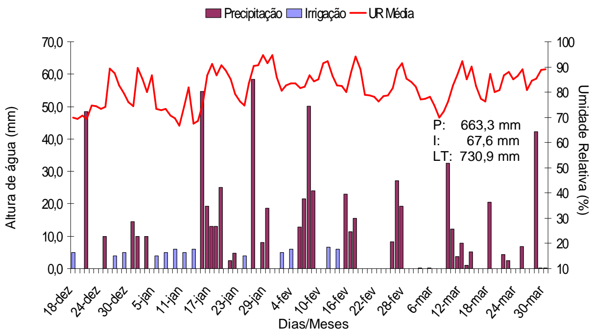
FIGURA 10. Valores diários de precipitação pluvial (mm), irrigação (mm) e umidade relativa (%), observados durante a condução do experimento, para a segunda semeadura em Selvíria – MS.
