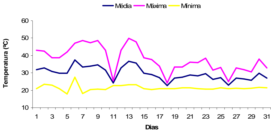
FIGURA 13. Temperatura máxima, mínima e média no mês de janeiro de 2009. Fernandópolis - SP.
