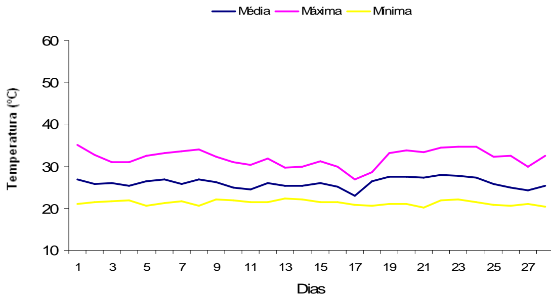
FIGURA 20. Temperatura máxima, mínima e média no mês de fevereiro de 2009. Selvíria – MS. .
