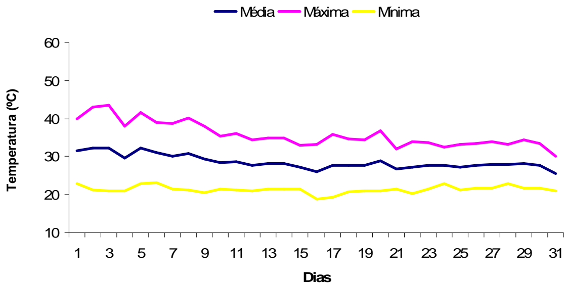
FIGURA 15. Temperatura máxima, mínima e média no mês de março de 2009. Fernandópolis – SP.
