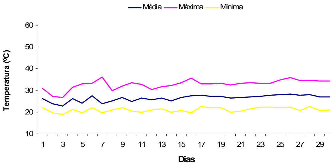
FIGURA 17. Temperatura máxima, mínima e média no mês de novembro de 2008. Selvíria – MS.
