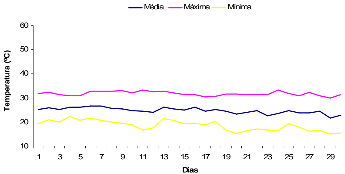
FIGURA 22. Temperatura máxima, mínima e média no mês de abril de 2009. Selvíria – MS.
