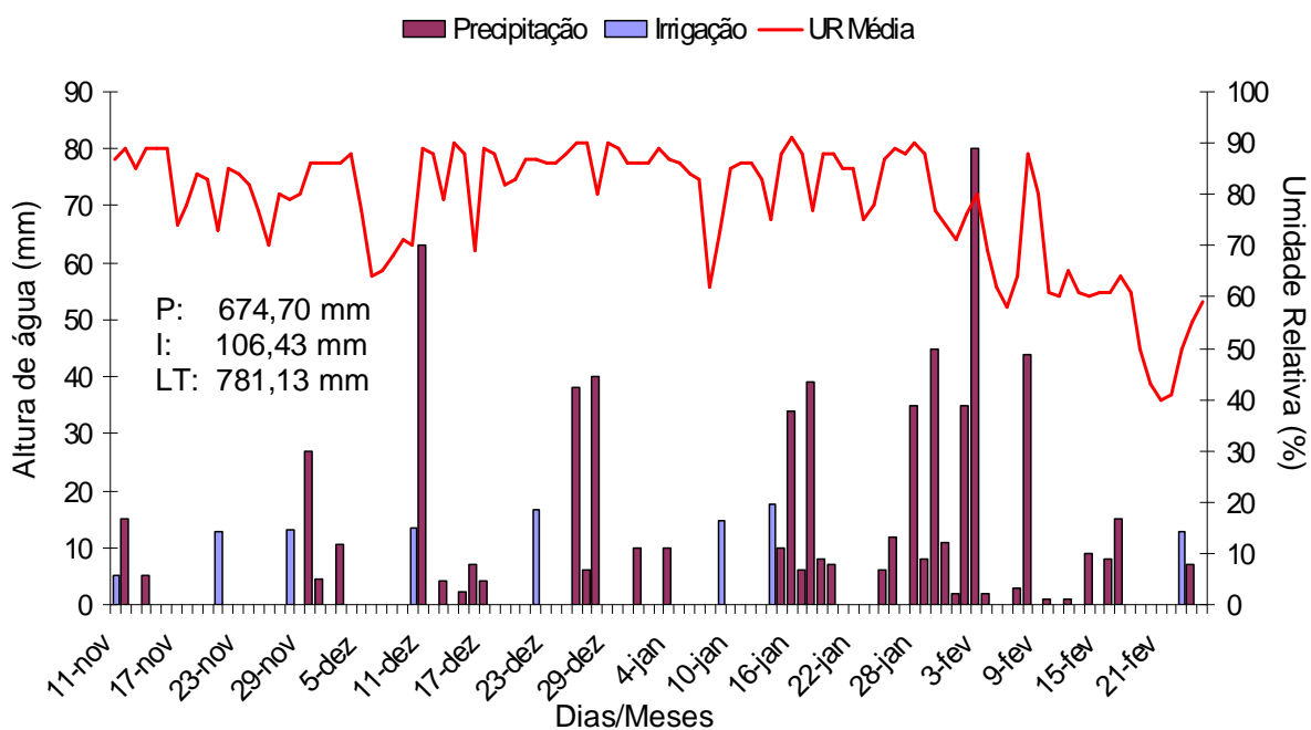
FIGURA 7. Valores diários de precipitação pluvial (mm), irrigação (mm) e umidade relativa (%), observados durante a condução do experimento, para a primeira semeadura em Fernandópolis – SP.
