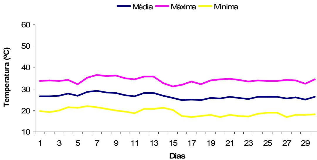
FIGURA 16. Temperatura máxima, mínima e média no mês de abril de 2009. Fernandópolis – SP.
