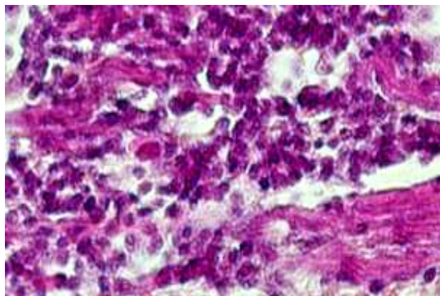
Figura 8. Histopatologia do coração de galo com integração de kDNA no seu genoma. Veja miocardite difusa, destruição de fibras cardíacas por múltiplas, confluentes unidades mínimas de rejeição. Fonte: Laboratório Multidisciplinar de Pesquisa em Doença de Chagas.
