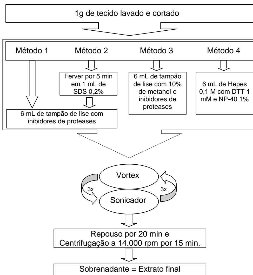
Figura 7. Fluxograma dos métodos de extração utilizados. Tampão de lise: uréia 7 M, tiouréia 2 M, Triton X-100 2%, DTT 1%. Coquetel de inibidores de proteases: EDTA 5 mM, PMSF 100 µM, TLCK 100 µM, TPCK 100 µM, pepstatina A 1 µM, leupeptina 100 µM.
