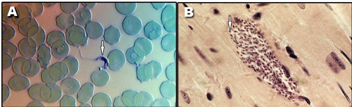
Figura 2. Estágios da forma de vida de T. cruzi . A: forma tripomastigota flagelada próxima à células sangüíneas. B: ninho do parasito na forma amastigota no tecido muscular. Fonte: www.sciencephoto.com
