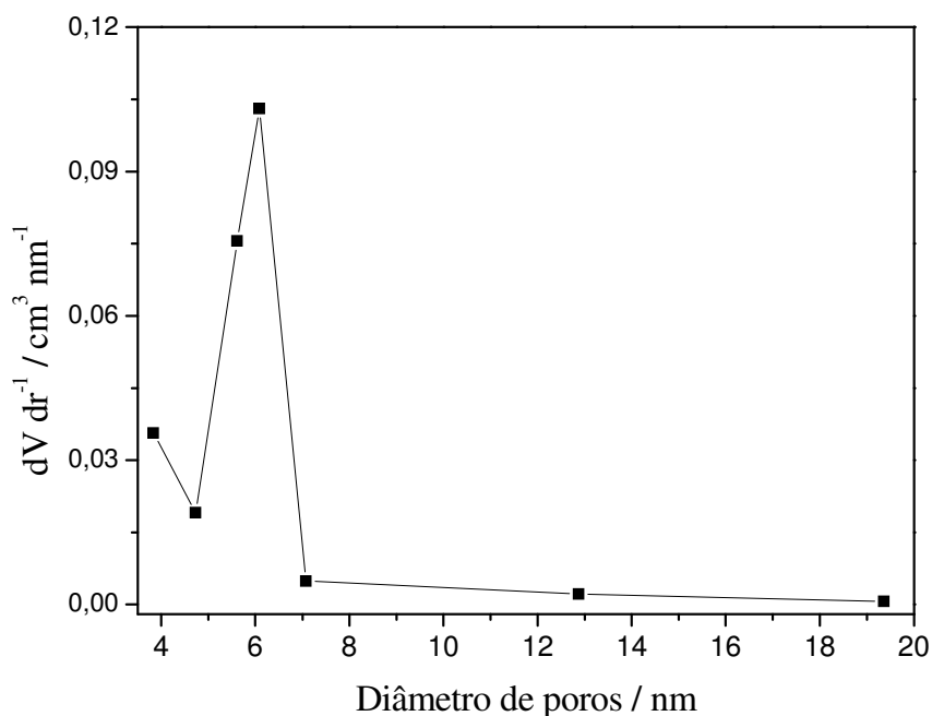
Figura 13: Distribuição de tamanho de poros da amostra S0.
