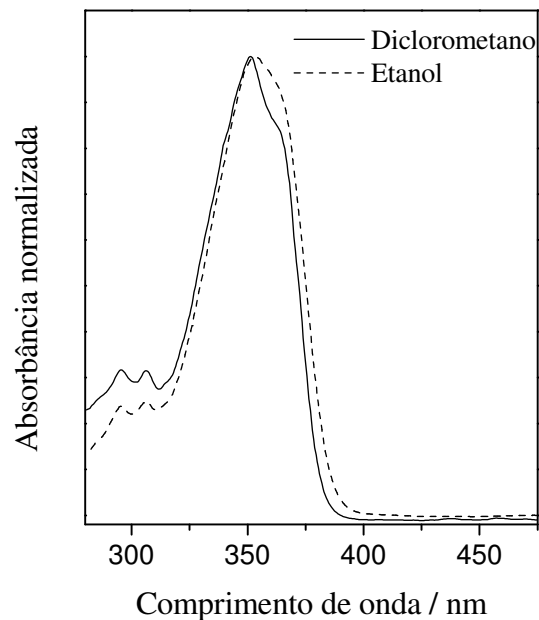
Figura 18: Espectros normalizados de absorção no UV-Vis em solução.
