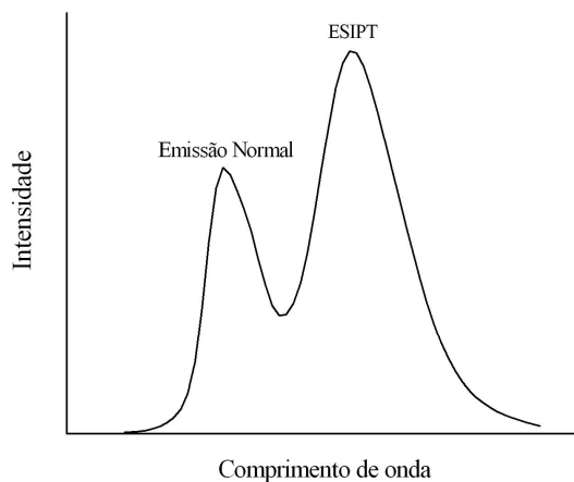
Figura 8: Representação genérica de dupla emissão de fluorescência.
