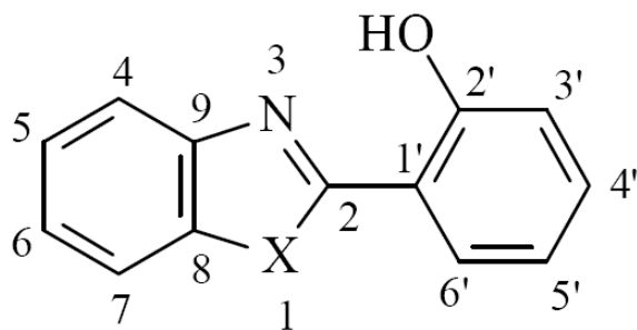
Figura 4: Representação do 2-(2'-hidroxifenil)benzazol.
