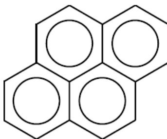
Figura 15: Fórmula estrutural do pireno.
