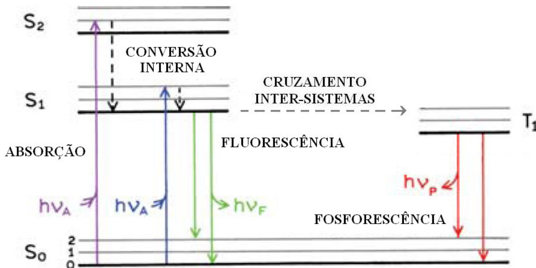
Figura 3: Diagrama de Jablonski simplificado. 57
