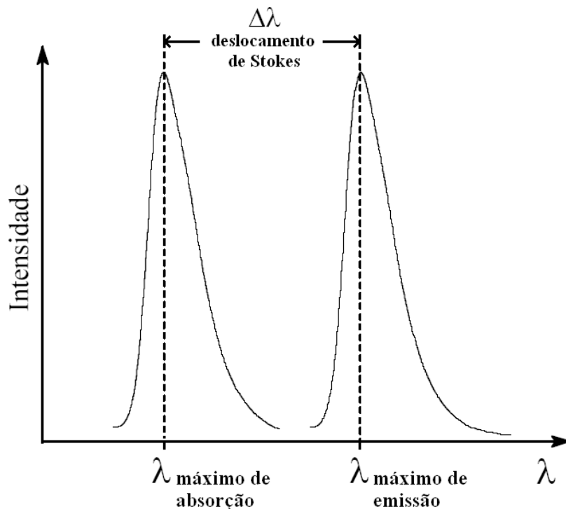
Figura 5: Deslocamento de Stokes.
