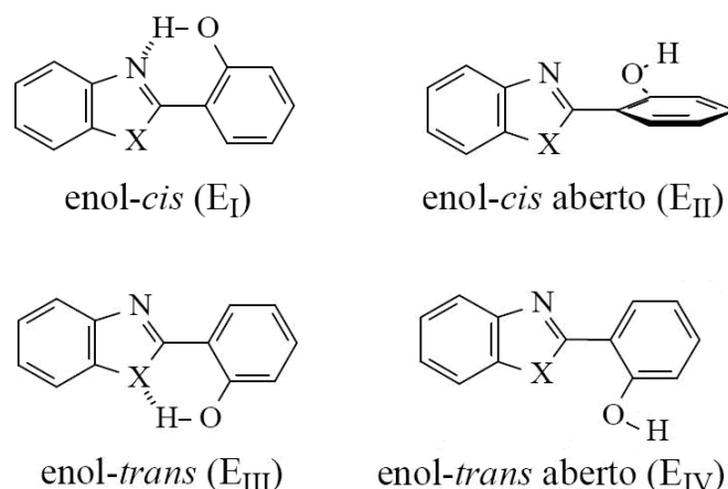
Figura 7: Geometrias dos confôrmeros dos 2-(2'-hidroxifenil)benzazóis.
