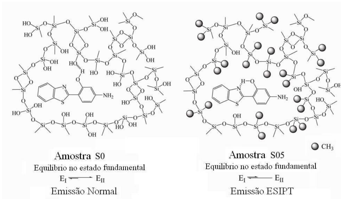
Figura 26: Representação do equilíbrio conformacional no estado fundamental para o corante 4-AHBT disperso nas amostras S0 e S05.
