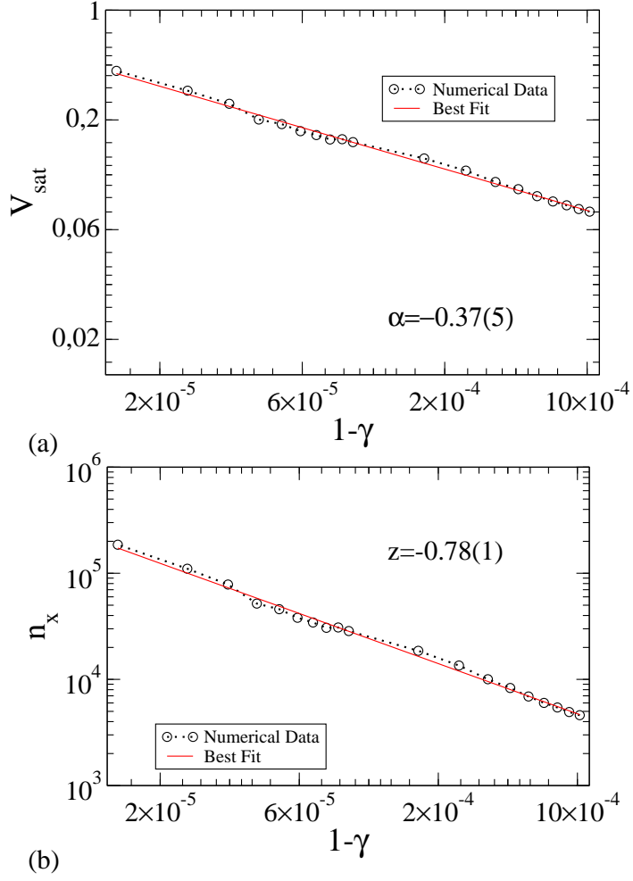
Figura 4.2: (a) Comportamento de \bar{V}_{\text{sat}} \times (1 - \gamma) . (b) Comportamento do número de crossover n_x em função de (1 - \gamma) . Um ajuste por lei de potência em (a) nos fornece \alpha = -0.37(5) e em (b) z = -0.78(1) .
