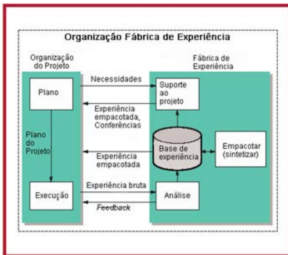
FIGURA 10: Organização fábrica de experiência – Victor Basili. Fonte: RUS; LINDVALL, 2002, p. 30. (Tradução do Autor – figura adaptada)
