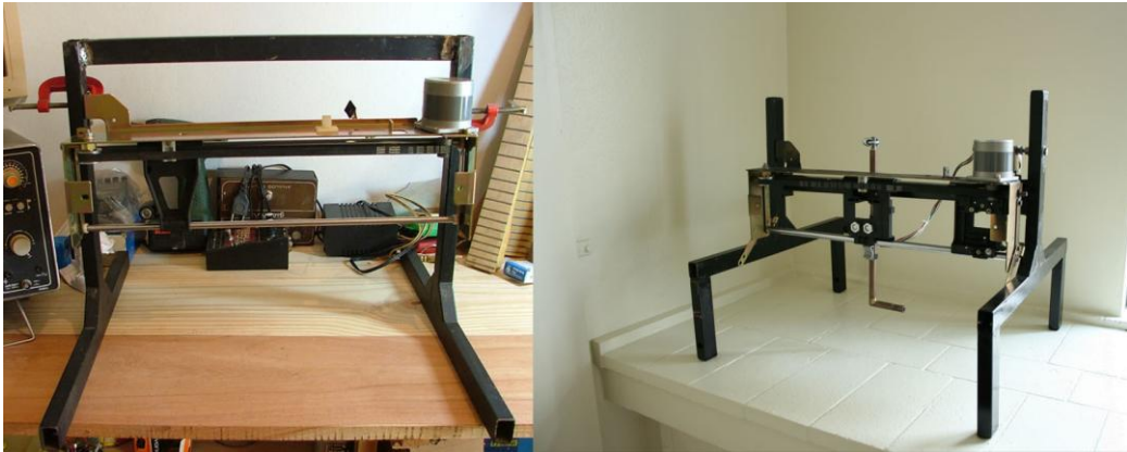
Figura 17 - O reator proposto: Estrutura inicial à esquerda e a atual à direita com mais espaço, permitindo melhor posicionamento da cuba.
