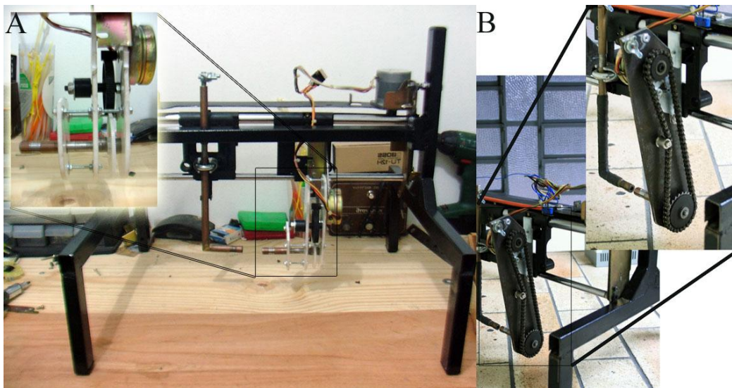
Figura 18 - Reator proposto: Detalhes do suporte e transmissão (A) em nylon e (B) em aço
