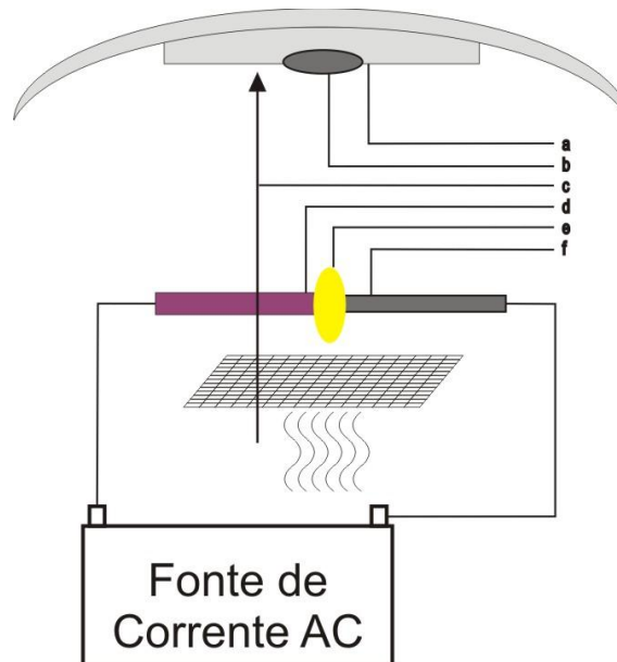
Figura 16 - Esquema do aparato utilizado para avaliar as condições de formação do plasma: (a) alumínio (com temperatura < 0^{\circ}\text{C} ), (b) crescimento de NTC, (c) fluxo de gases (provenientes da sublimação), (d) eletrodo de ferro, (e) plasma, (f) eletrodo de grafite
