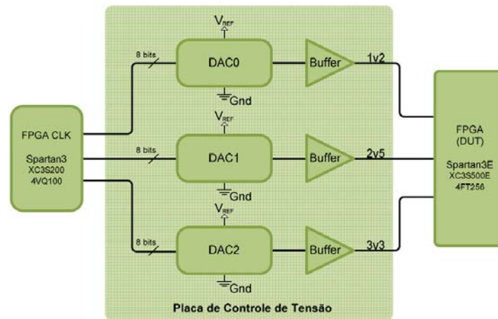
Figura 6.5 - Diagrama da placa de alimentação e injeção de falhas (61).
