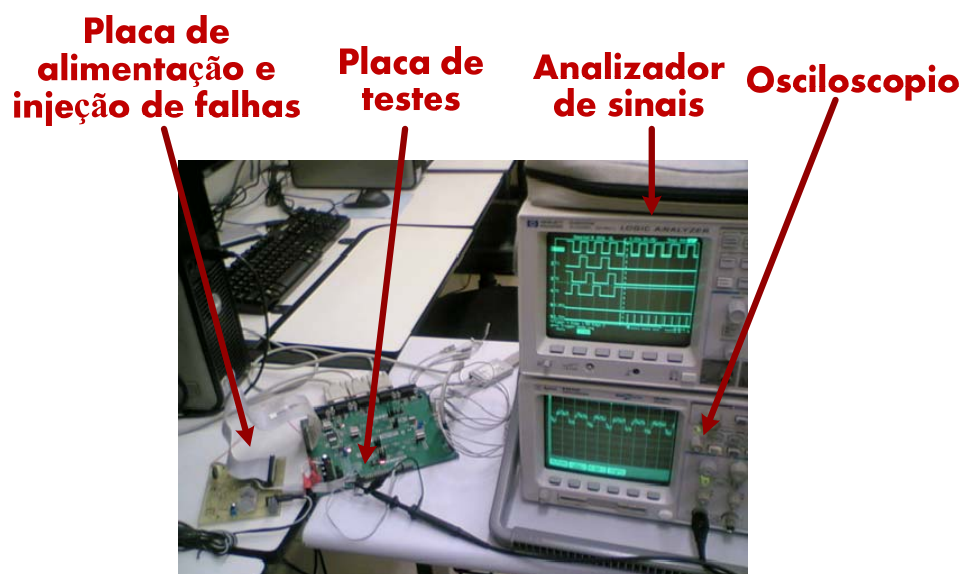
Figura 10.4 – Conexão dos componentes para os experimentos.
