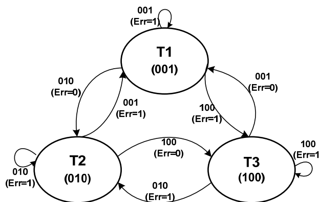
Figura 5.4 - Máquina de estados que determina erros de seqüência num ambiente Round Robin .
