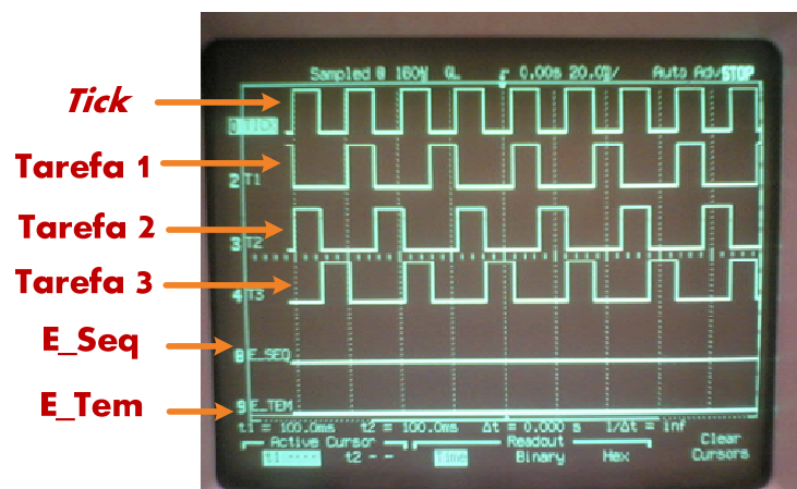
Figura 10.1 – Sinais E_Seq e E_Tem quando as tarefas T1, T2 e T3 não apresentam falhas.
