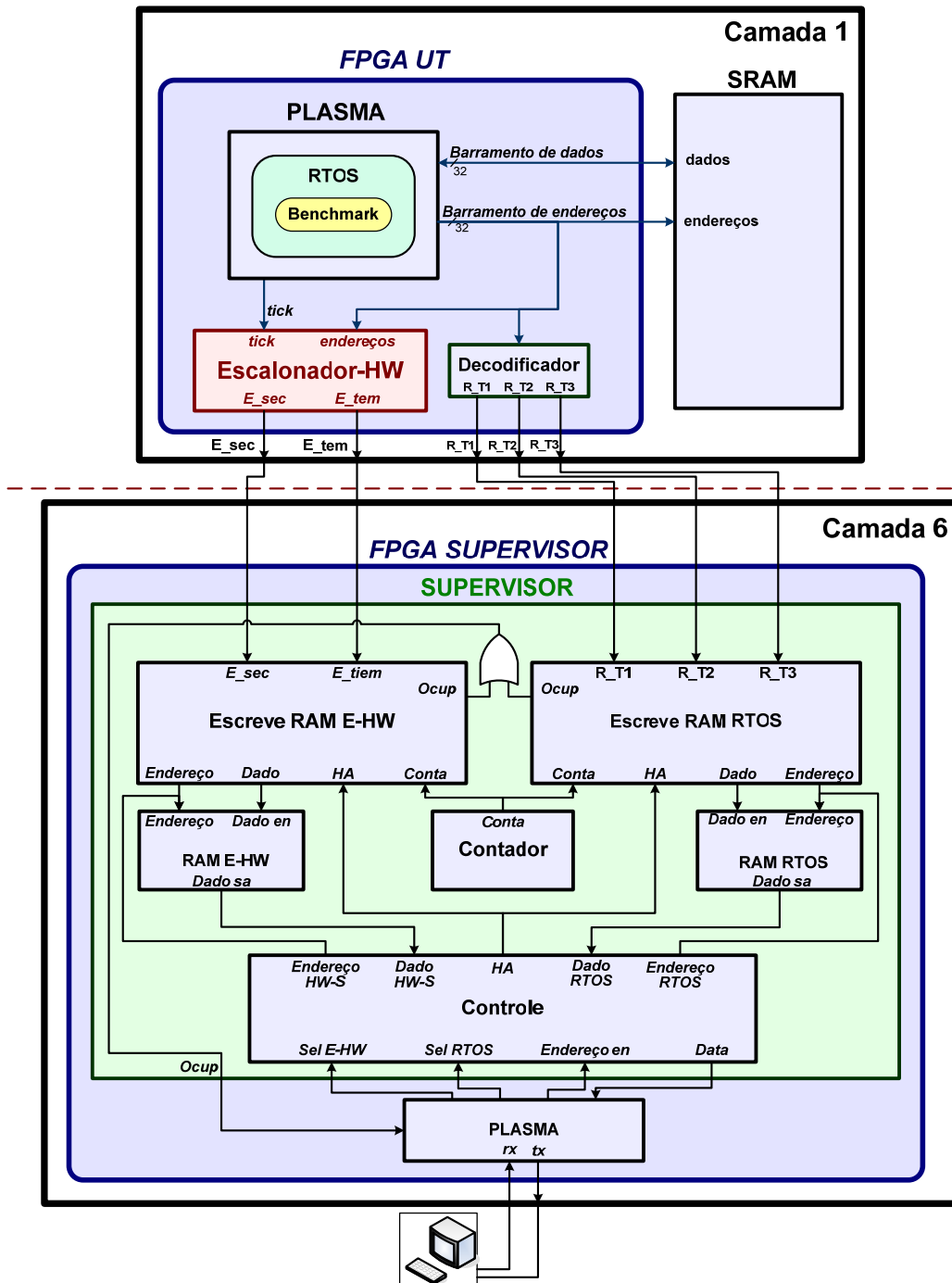
Figura 8.1 - Esquema da plataforma de teste.
