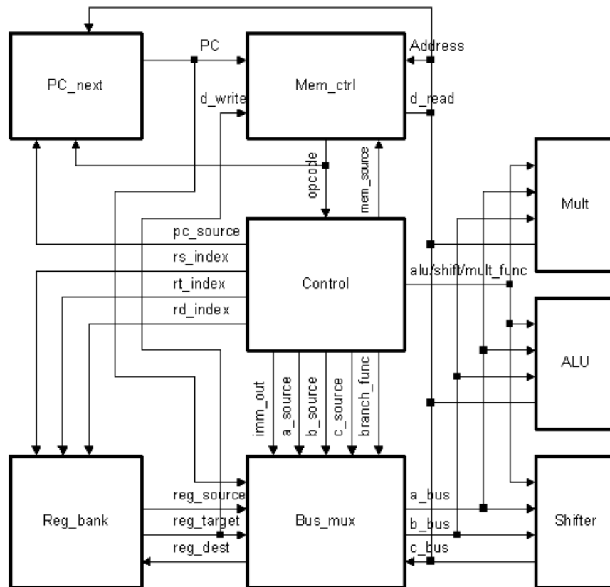
Figura 6.1 - Diagrama de blocos da arquitetura básica do processador Plasma (59).
