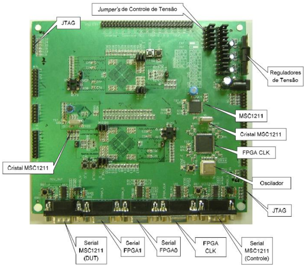
Figura 6.3 - Vista inferior da plataforma de teste (Camada 6) (61).
