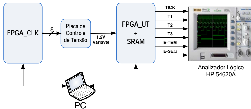
Figura 9.5 - Diagrama de conexões utilizada para realização de injeção de falhas por ruído em linha de alimentação.
