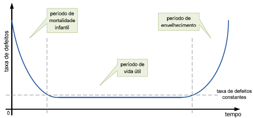
Figura 3.5: Curva da banheira (37).
