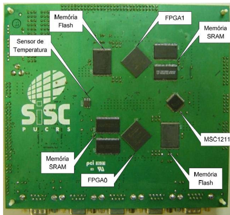
Figura 6.4 - Vista superior da plataforma de teste (Camada 1) (61).
