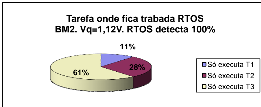
Figura 10.12 - Porcentagem de vezes que o RTOS ficou executando cada tarefa, usando Vq=1,12V.
