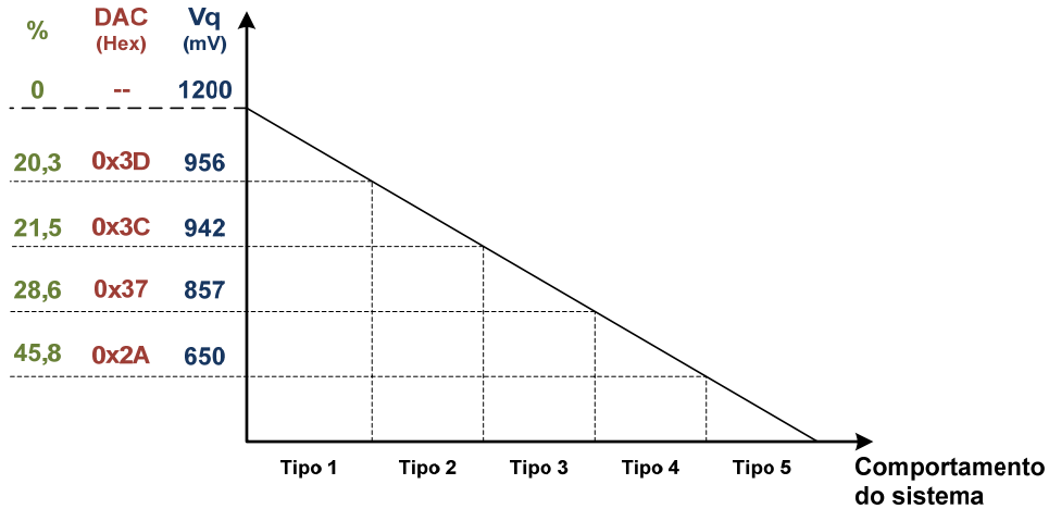
Figura 10.6 - Comportamento do Sistema a variação de tensão tipo queda para BM1
