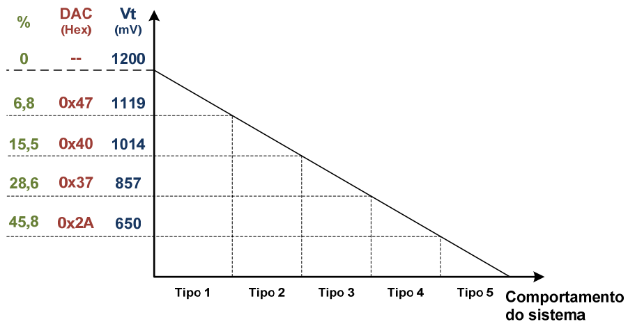
Figura 10.10 - Comportamento do Sistema a variação de voltagem tipo rampa para BM2.
