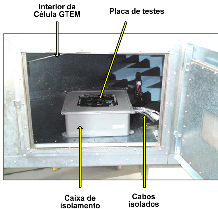
Figura 10.14 – Imagens dos equipamentos utilizados nos experimentos da EMI irradiada, nos laboratórios do INTI – Argentina. a) Todos os equipamentos utilizados. b) Interior da célula GTEM com a placa de teste na caixa metálica e cabos isolados.
