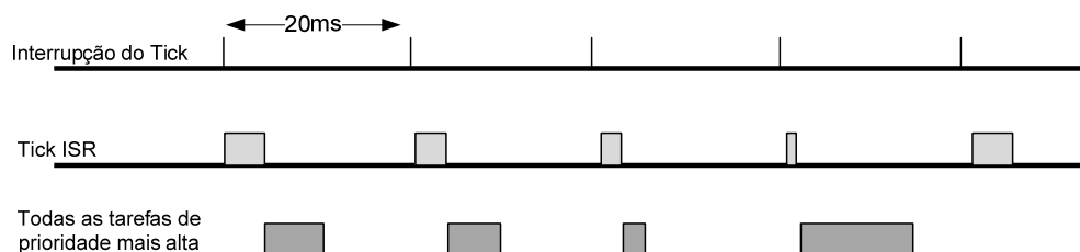
Figura 2.4 - Exemplo do Tick e o escalonamento das tarefas (baseado em (28)).
