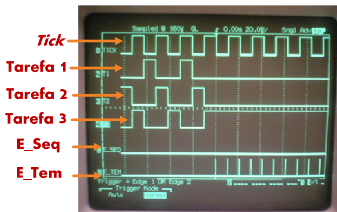
Figura 10.7 – Momento do primeiro erro de tempo.
