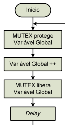
Figura 7.6: Fluxograma das tarefas do BM3.
