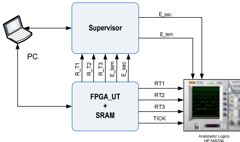
Figura 9.1 - Esquema de conexões para realização da validação.
