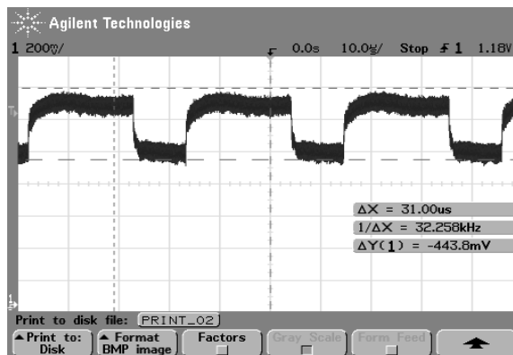
Figura 9.4 - Imagem da variação de tensão na linha de alimentação.
