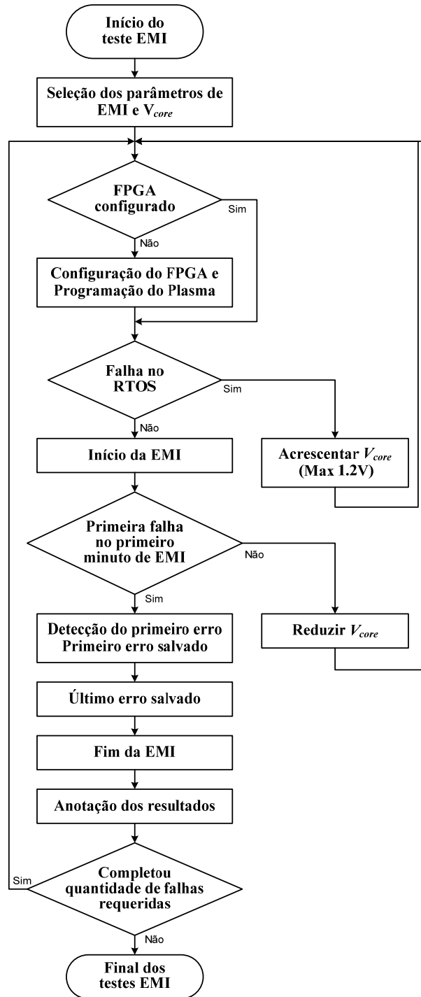
Figura 9.8: Fluxograma adotado durante os experimentos de EMI.
