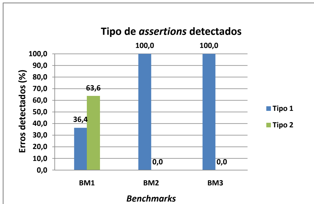
Figura 10.16 – Porcentagem de assertions enviados pelo RTOS nos experimentos de EMI.
