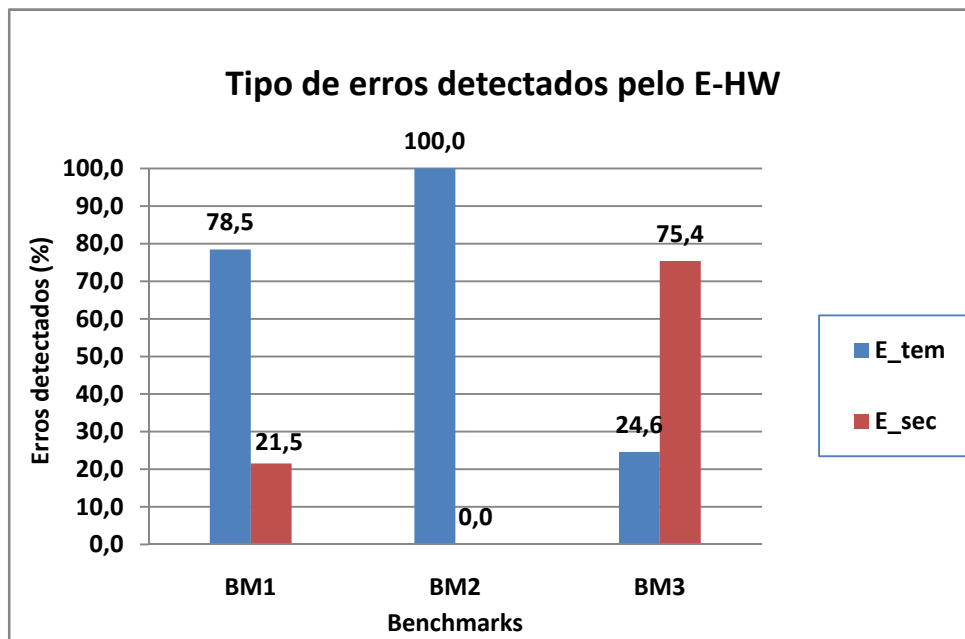
Figura 10.15 – Porcentagem dos tipos de erros detectados pelo E-HW.
