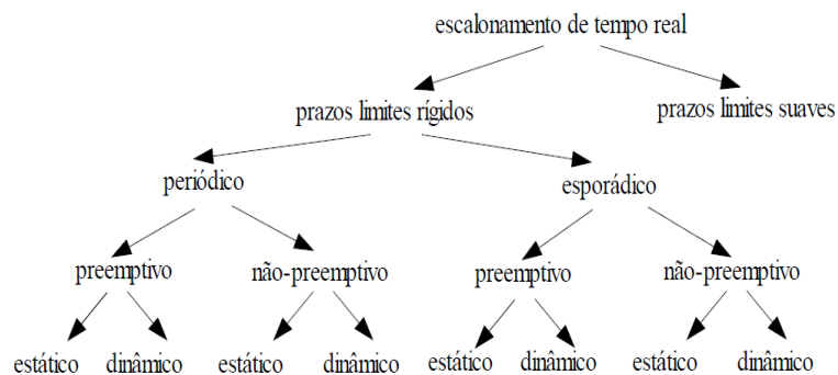
Figura 2.6 - Classes de algoritmos de escalonamento (34).
