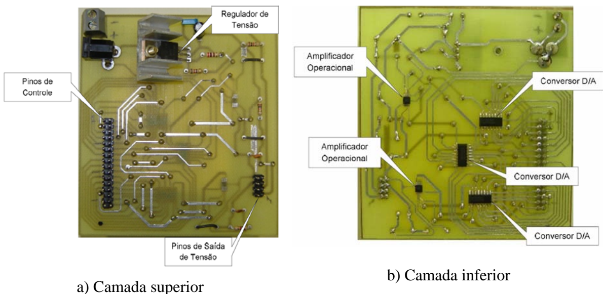
Figura 6.6 – Fotos da placa de alimentação e injeção de falhas.
