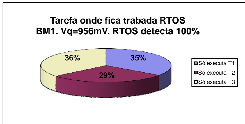
Figura 10.8 – Porcentagem de vezes que o RTOS ficou executando cada tarefa, usando Vq=956mV.
