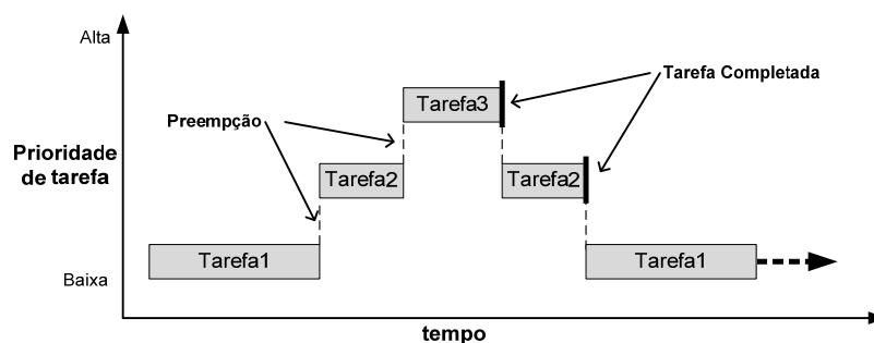
Figura 2.7 - Escalonamento preemptivo baseado em prioridades (22).
