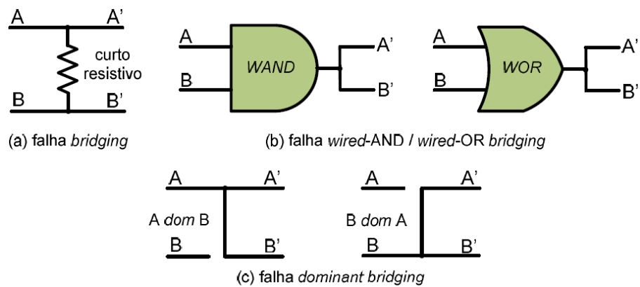
Figura 3.4 - Modelo de falha bridging (46).
