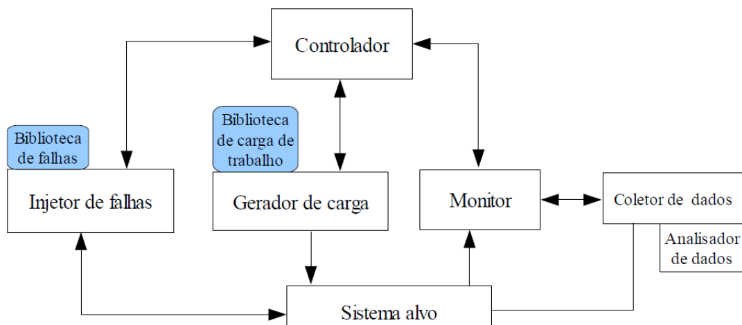
Figura 4.1 - Arquitetura de um Ambiente de Injeção de Falhas (51).
