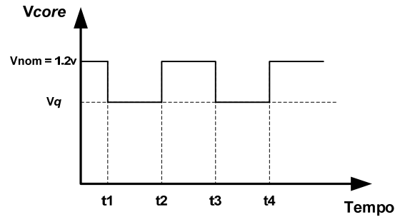
Figura 9.3 - Variação de tensão tipo queda.
