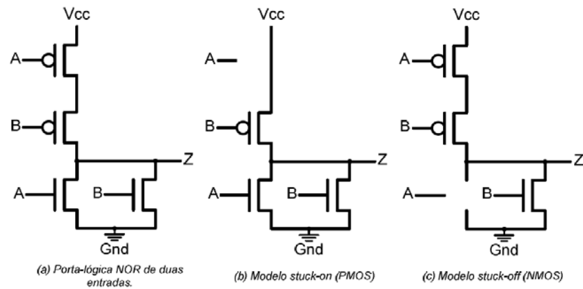
Figura 3.3 - Modelo de falha Transistor-Level Stuck (46).
