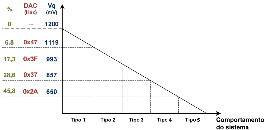
Figura 10.11 - Comportamento do Sistema a variação de voltagem tipo queda para BM2.
