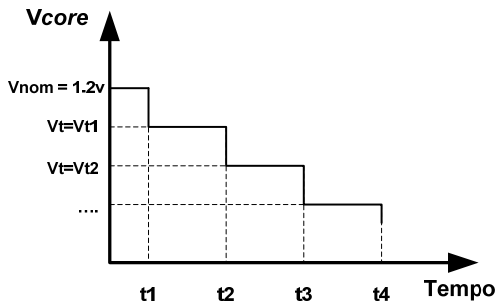
Figura 9.2 - Variação de tensão tipo Rampa.
