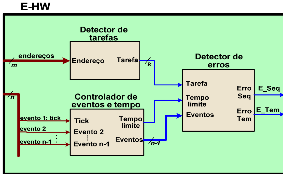
Figura 5.2 - Diagrama de blocos internos do E-HW.
