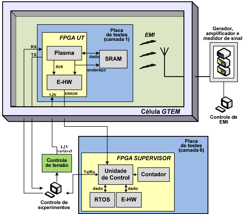
Figura 9.7 Esquema de conexões para teste EMI no INTI.
