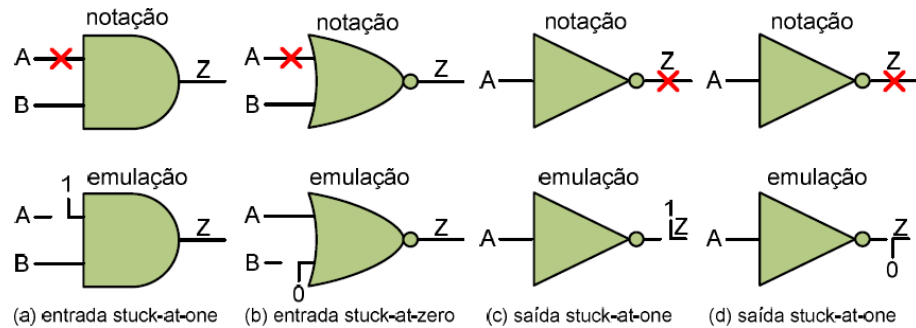
Figura 3.2 - Notação e emulação do modelo de falha Stuck-at (46).
