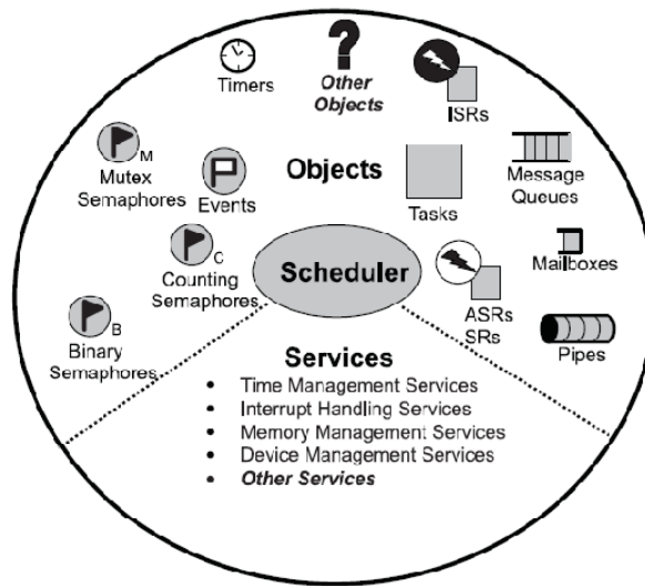
Figura 2.3 - Componentes típicos do kernel do RTOS (22).
