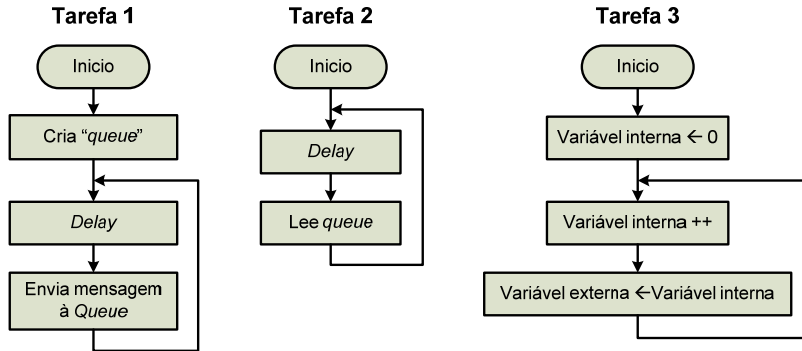
Figura 7.4 - Fluxogramas das tarefas do BM2.
