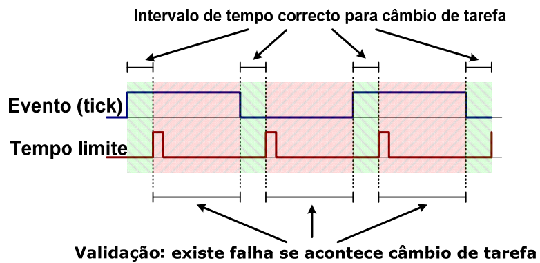
Figura 5.5 - Exemplo para determinação de erros de tempo associados a mudança de tarefa.
