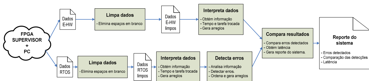
Figura 8.2 - Diagrama de blocos do Programa de Análise de Dados.
