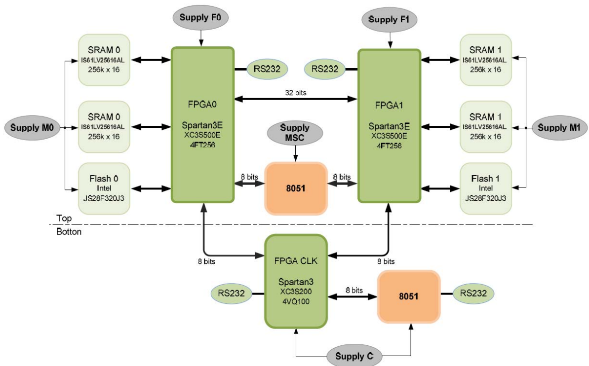
Figura 6.2 - Esquemático genérico da plataforma de teste (61).
