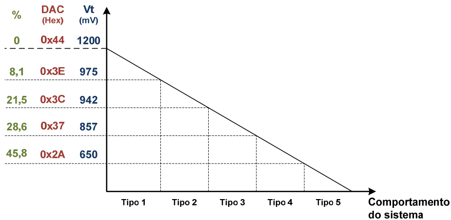
Figura 10.5 - Comportamento do Sistema a variação de tensão tipo rampa para BM1
