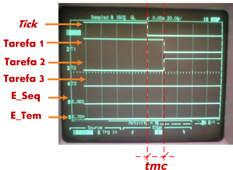
Figura 10.2 – Momento da mudança de contexto.
