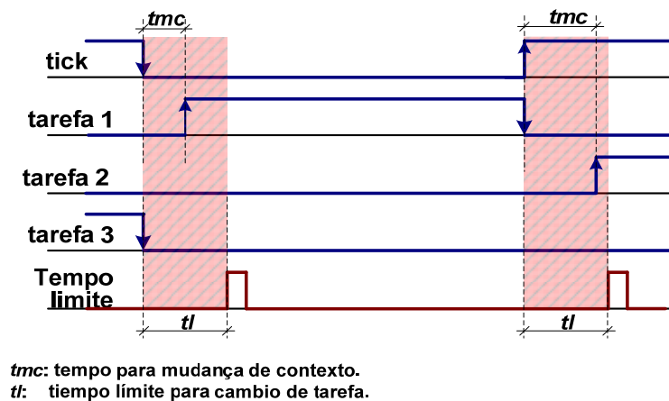
Figura 5.3 - Tempo limite gerado pelo bloco controlador de eventos e tempos .
