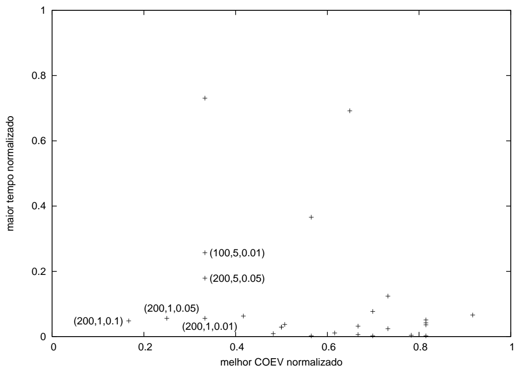
Figura 5.2: Resultados normalizados extremos obtidos com diferentes combinações de parâmetros.
