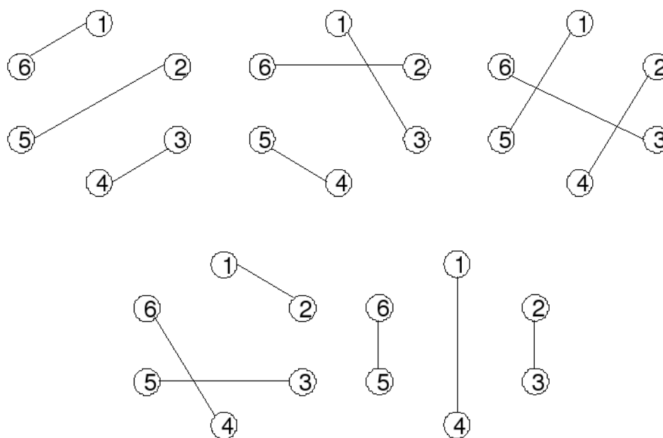
Figura 2.7: Exemplo de 1-fatoração do grafo completo K_6 .
