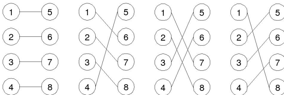
Figura 2.9: Primeira fase do método de de Werra aplicado sobre o grafo completo K_8 .
