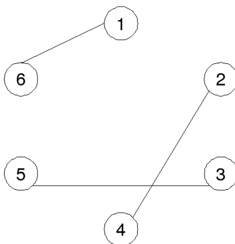
Figura 2.5: Exemplo de 1-fator do grafo completo K_6 .
