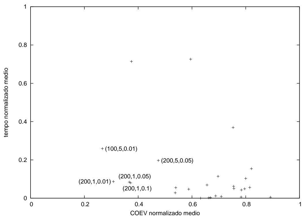
Figura 5.1: Resultados normalizados médios obtidos com diferentes combinações de parâmetros.
