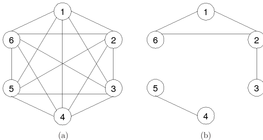
Figura 2.4: (a) Grafo completo K_6 e (b) um de seus possíveis fatores.
