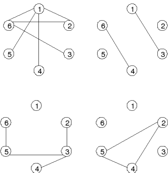
Figura 2.6: Exemplo de fatoração do grafo completo K_6 .
