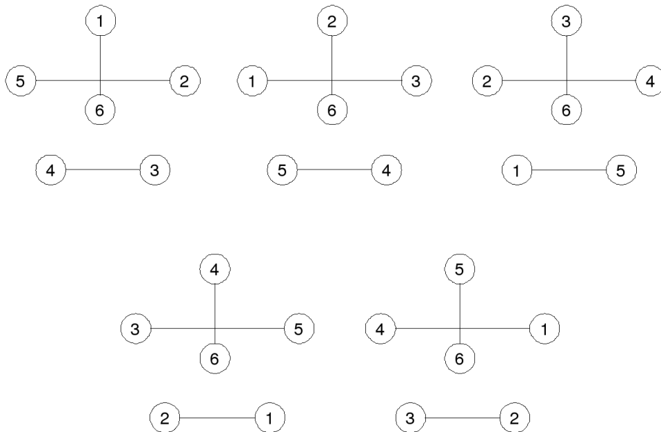
Figura 2.8: Método do polígono aplicado sobre o grafo completo K_6 .
