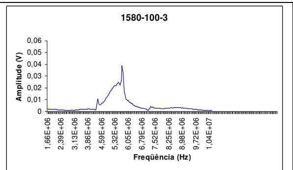
Pastilha 1580-100-3 com porosidade de 5,54%
