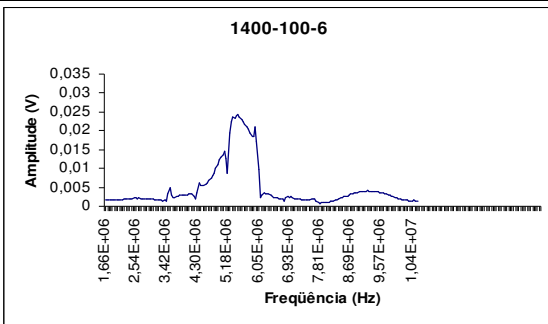
Pastilha 1400-100-6 com porosidade de 29,00%
