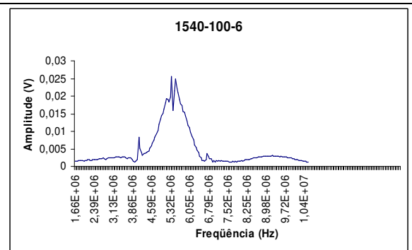
Pastilha 1540-100-6 com porosidade de 10,80%
