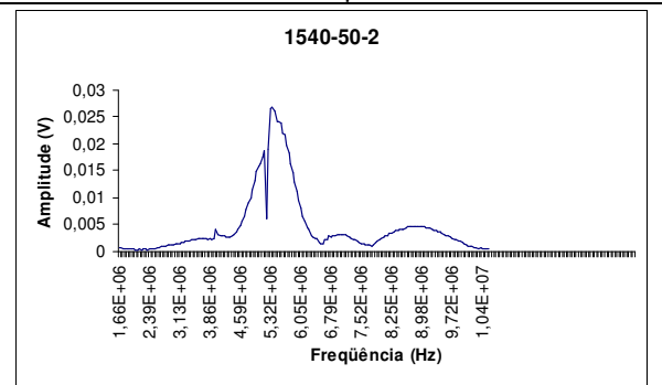
Pastilha 1540-50-2 com porosidade de 11,10%
