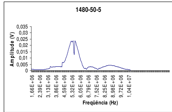
Pastilha 1480-50-5 com porosidade de 21,20%
