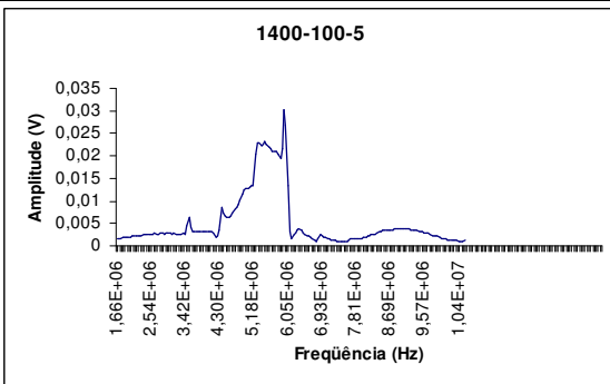
Pastilha 1400-100-5 com porosidade de 28,70%
