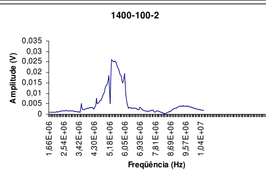
Pastilha 1400-100-2 com porosidade de 28,70%
