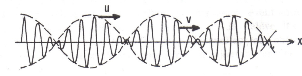
Figura 10: Pulso ultra-sônico, onde é possível notar as velocidades de fase ( v ) e a de grupo ( u ) [23].
