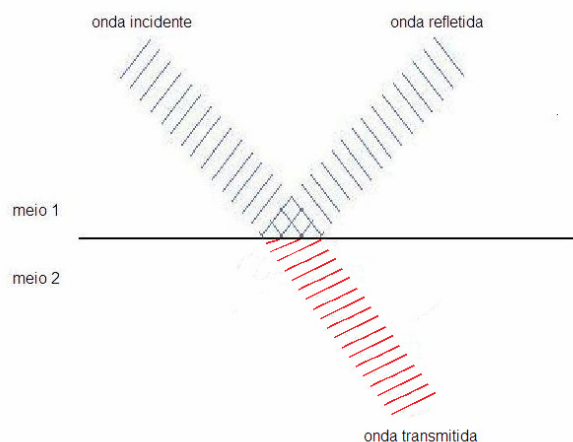
Figura 5: Reflexão e refração de uma onda mecânica.
