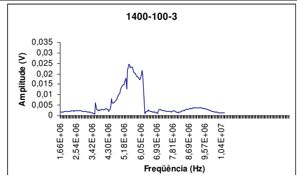
Pastilha 1400-100-3 com porosidade de 28,70%
