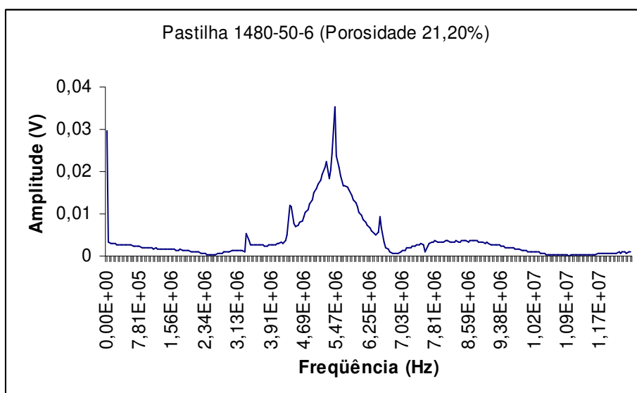
Figura 19: Espectro de frequência da pastilha 1480-50-6, que possui a porosidade de 21,20%, gerada por um transdutor longitudinal de 5MHz.
