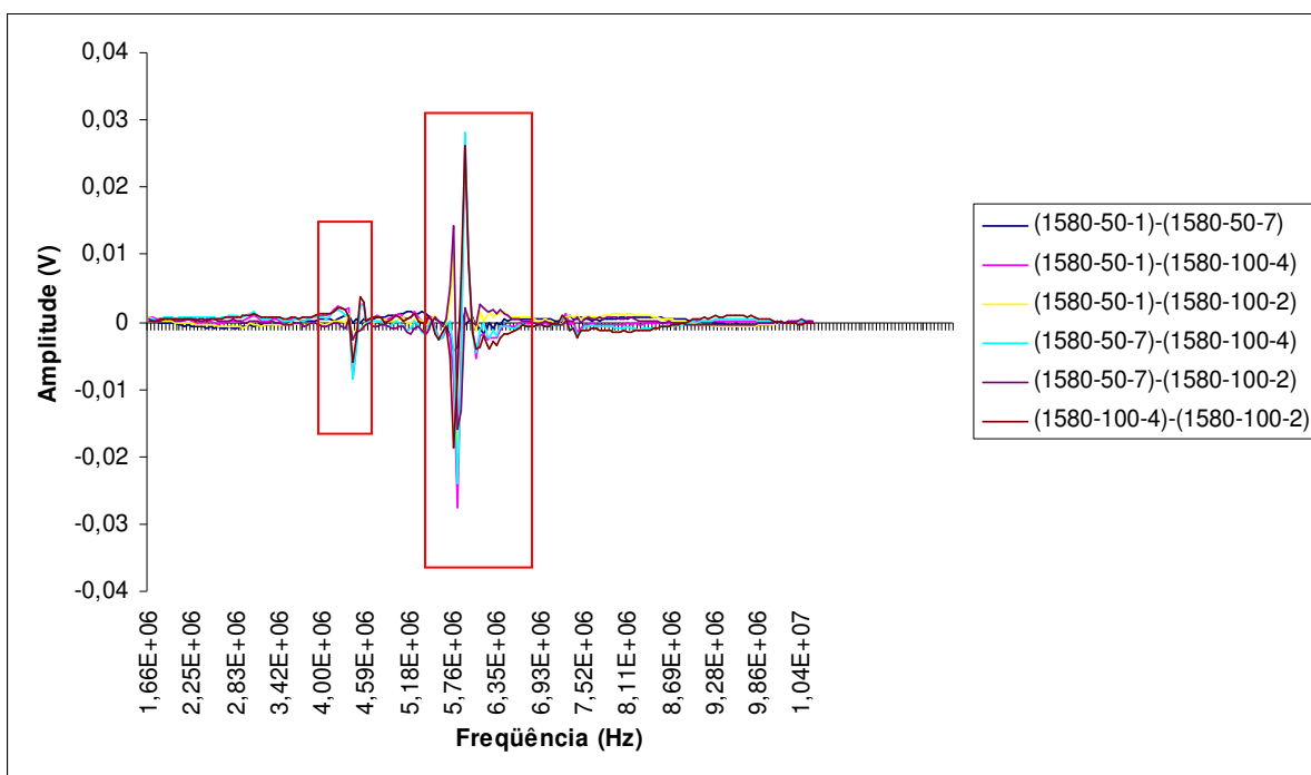
Figura 39: Diferenças dos espectros de freqüência das pastilhas sinterizadas a temperatura de 1580°C analisadas pelo MEV sobrepostos, mostrando as principais freqüências alteradas, entre os retângulos vermelhos, pelas distribuições de poros no interior dessas pastilhas.
