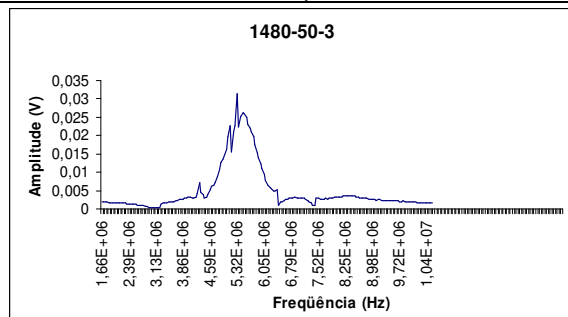
Pastilha 1480-50-3 com porosidade de 20,60%
