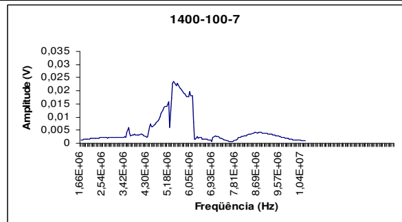
Pastilha 1400-100-7 com porosidade de 28,70%
