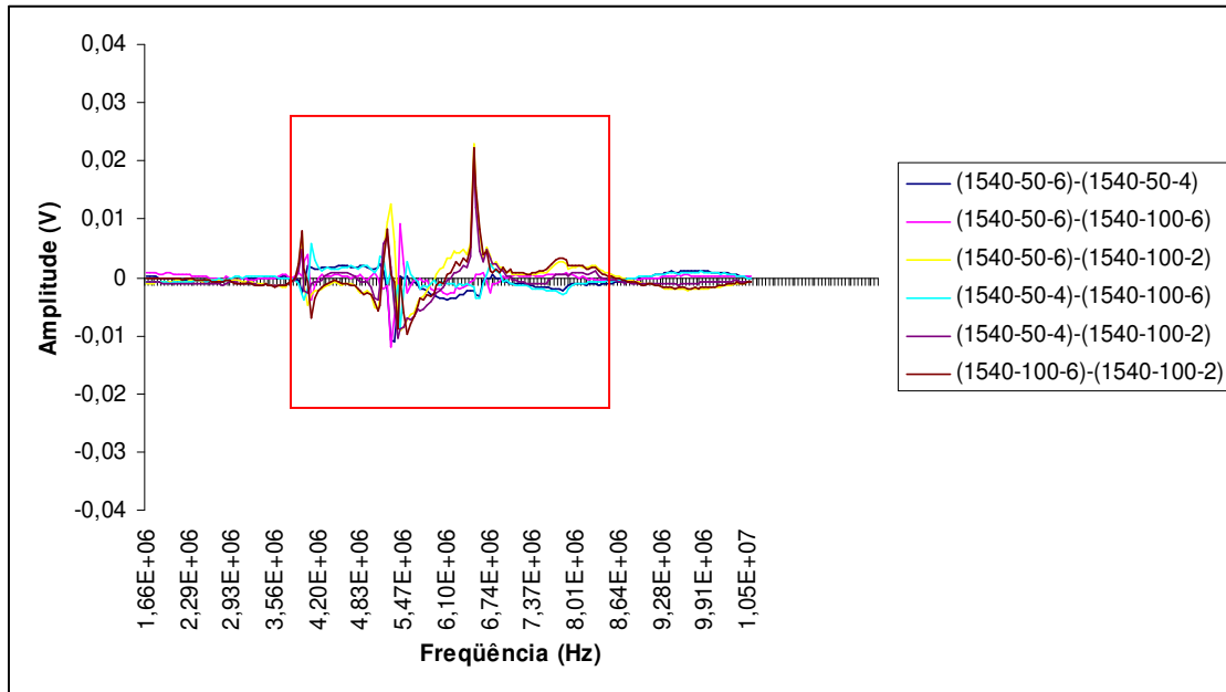
Figura 42: Diferenças dos espectros de freqüência das pastilhas sinterizadas a temperatura de 1540°C analisadas pelo MEV sobrepostos, mostrando as principais freqüências alteradas, entre o retângulo vermelho, pelas distribuições de poros no interior dessas pastilhas.
