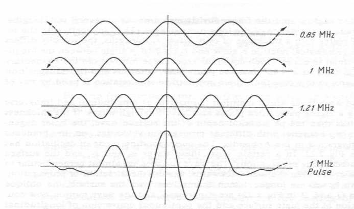
Figura 9: Superposição de três ondas de frequências 0,85MHz, 1MHz e 1,21MHz gerando um pulso de 1MHz [19].
