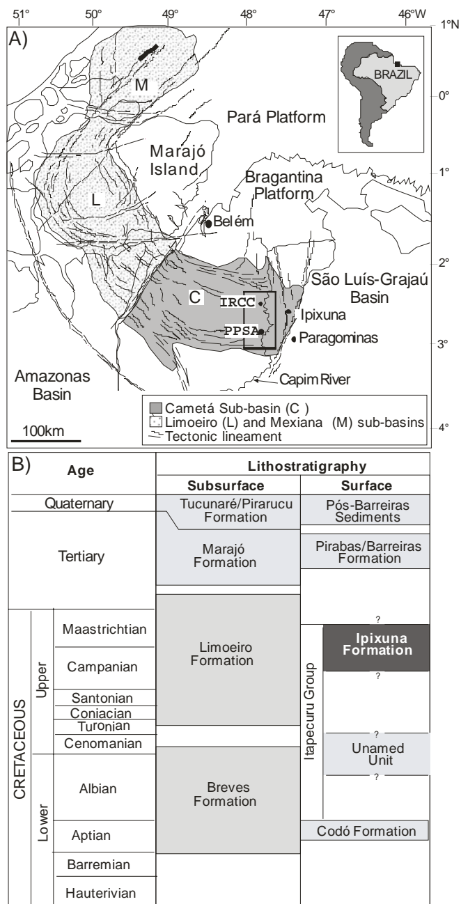
Figura 1.1: A) Mapa de localização da área de estudo, Sub-Bacia de Cameté, Sistema de Graben do Marajó, com indicação das minas de caulim estudadas, PPSA e RCC. SBC=Sub-Bacia de Cameté, SBL=Sub-Bacia de Limoeiro e SBM=Sub-Bacia de Mexiana. B) Carta Litoestratigráfica da Sub-Bacia de Cameté.
