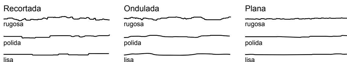
Figura 3 – Perfis de rugosidade (Barton et al. 1974 apud Serra Junior e Ojima, 1998).
