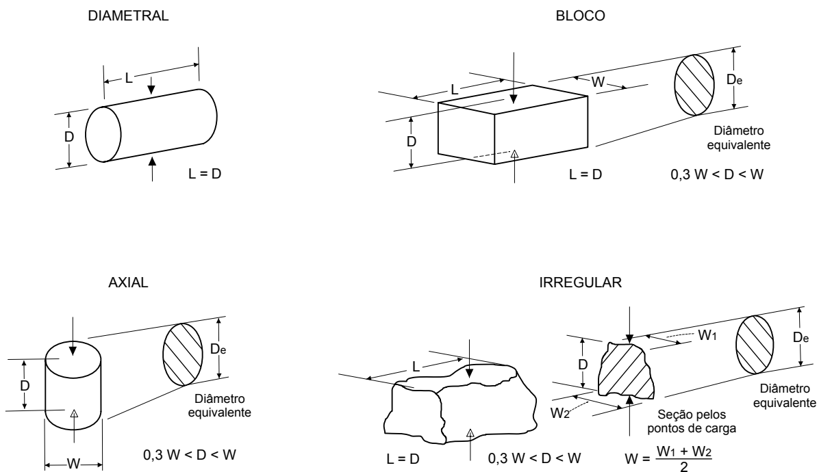
Figura 1 – Forma da amostra e tipo de ensaio de compressão puntual indicado. (ISRM, 1985)
