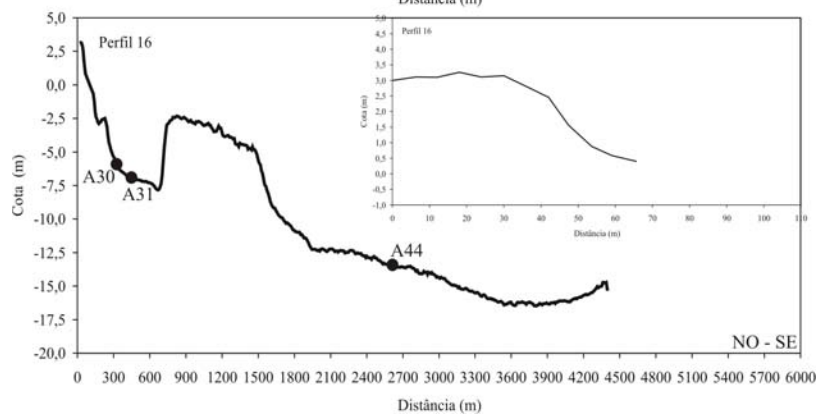
Perfis Topobatimétricos de 13 a 16.
