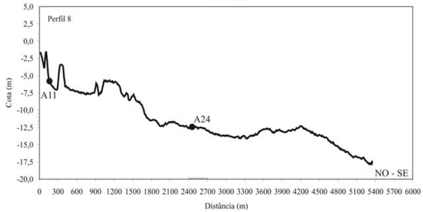
Perfis Batimétricos de 5 a 8.
