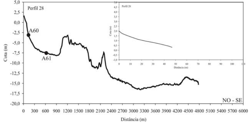
Perfis Topobatimétricos de 25 a 28.
