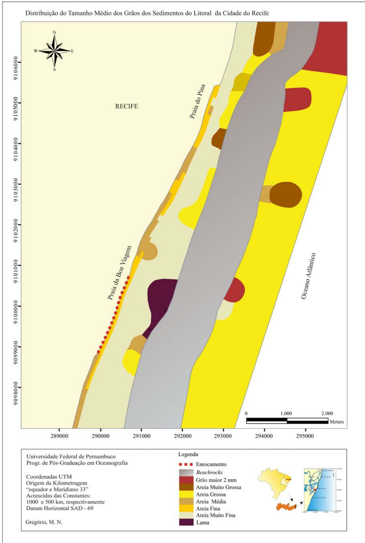
Figura 6 - Distribuição dos valores do tamanho médio do grão na região da pós-praia, face da praia e plataforma continental interna.
