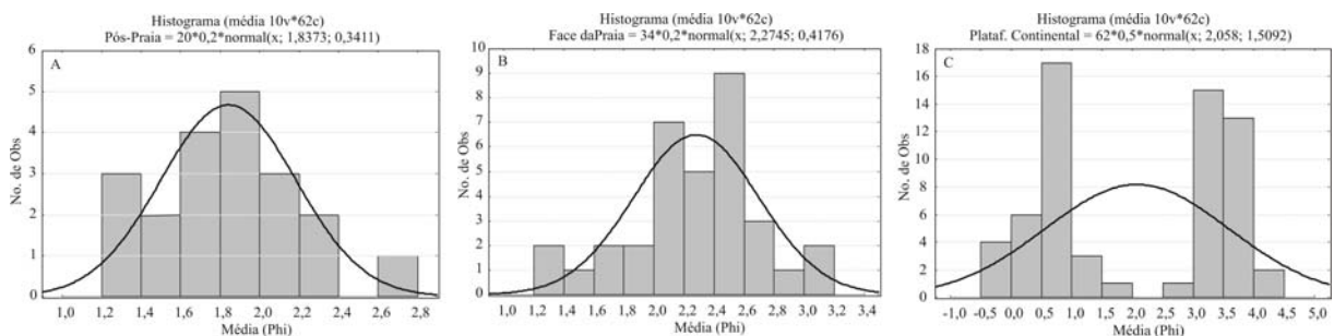
Figura 5 – Histogramas do tamanho médio dos grãos das regiões: A - pós-praia; B - face da Praia; C – plataforma continental interna.
