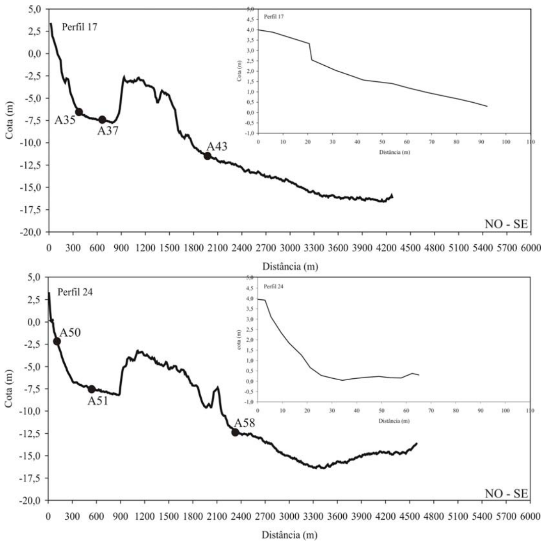
Figura 18 - Perfis batimétricos e topográficos 17 e 24 localizados no Setor B, e localização das amostras de sedimentos.
