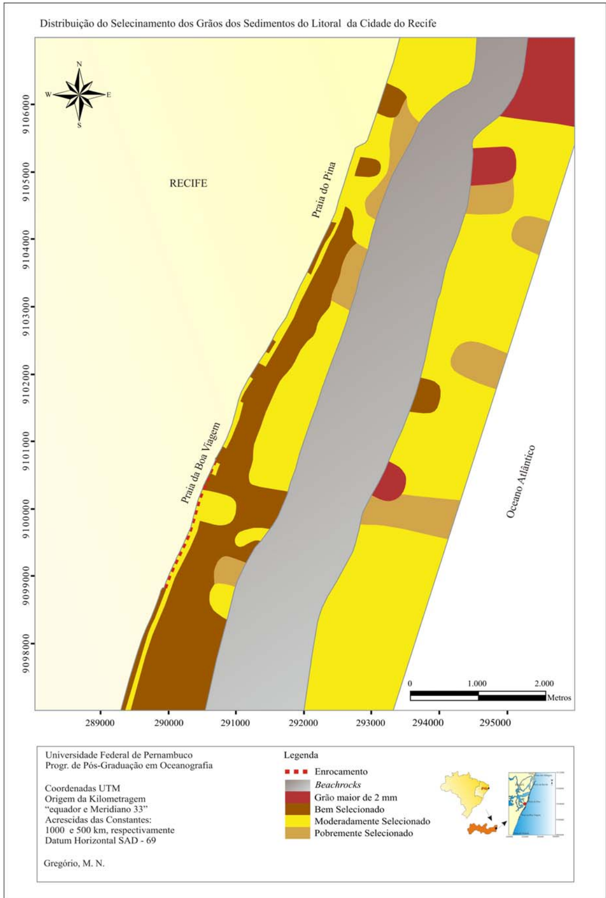
Figura 8 – Distribuição dos valores de seleccionamento dos grãos das regiões da pós-praia, face da praia e plataforma continental interna.
