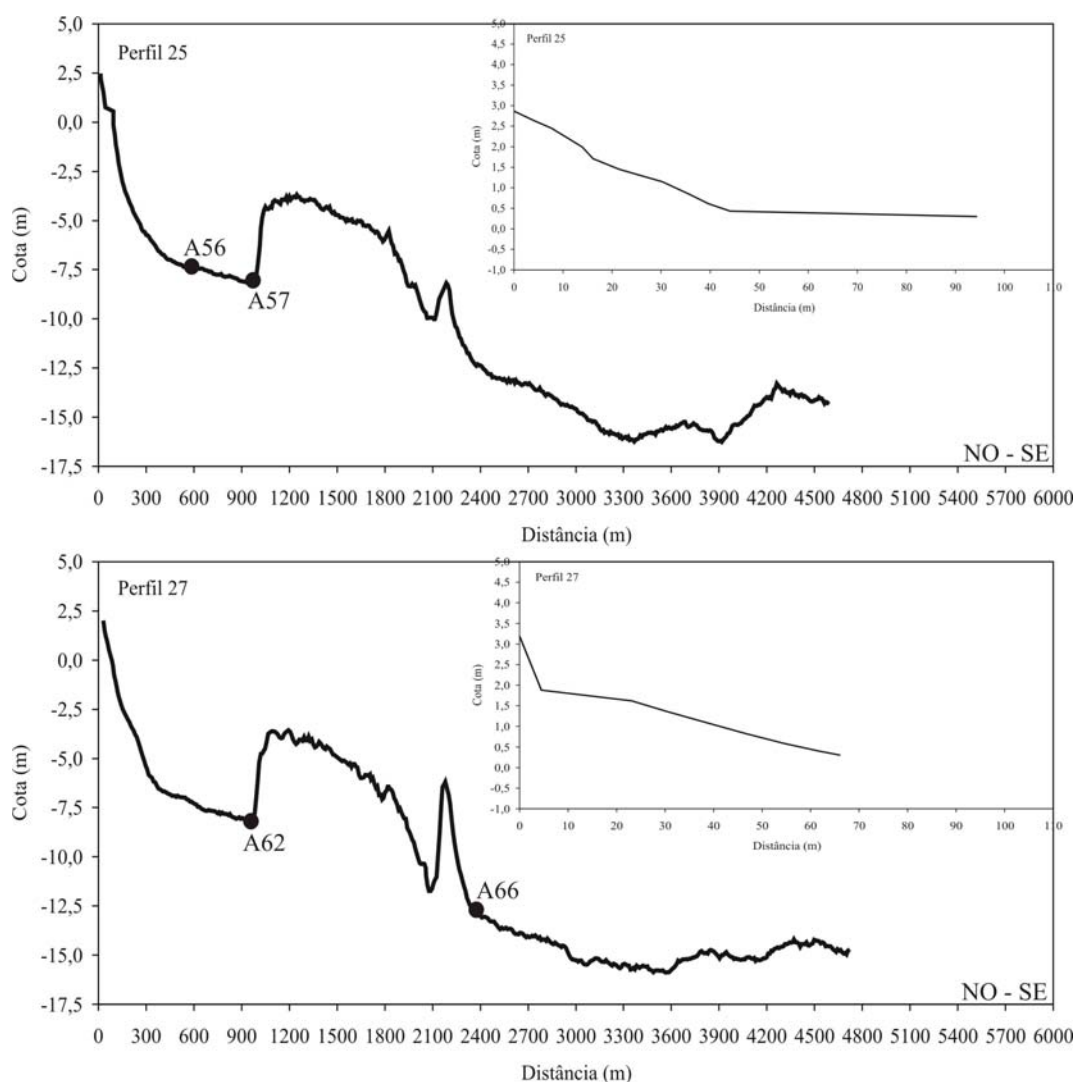
Figura 19 - Perfis batimétricos e topográficos 25 e 27 localizados no Setor B, e localização das amostras de sedimentos.
