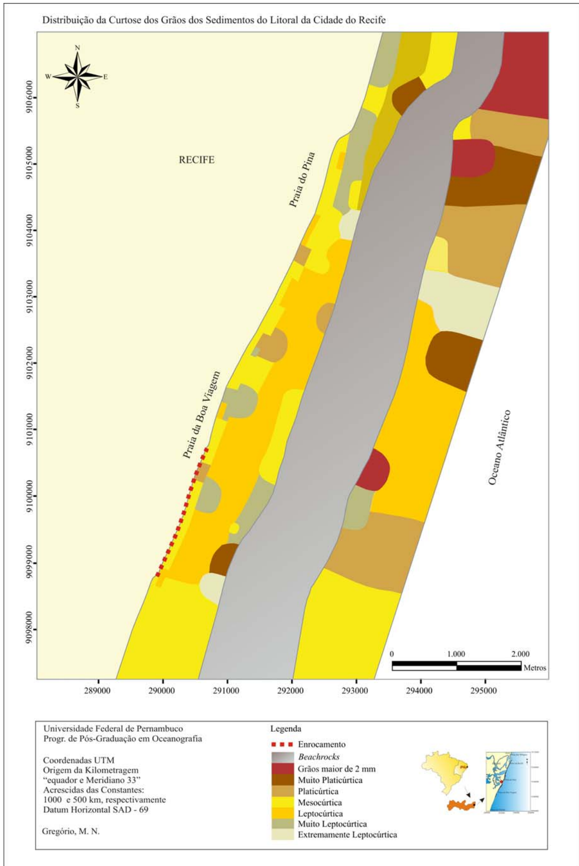
Figura 12 – Distribuição dos valores de curtose das regiões pós-praia, face da praia e plataforma continental interna.
