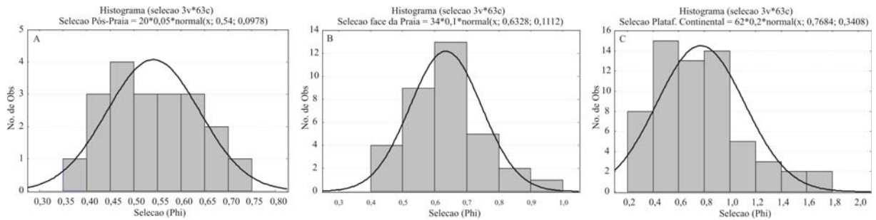
Figura 7 – Histograma dos valores de seleção dos grãos das regiões: A - pós-praia; B - face da praia; C – plataforma continental interna.
