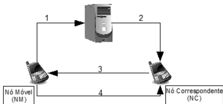
Figura 5.9: Estabelecimento da associação em HIP.
