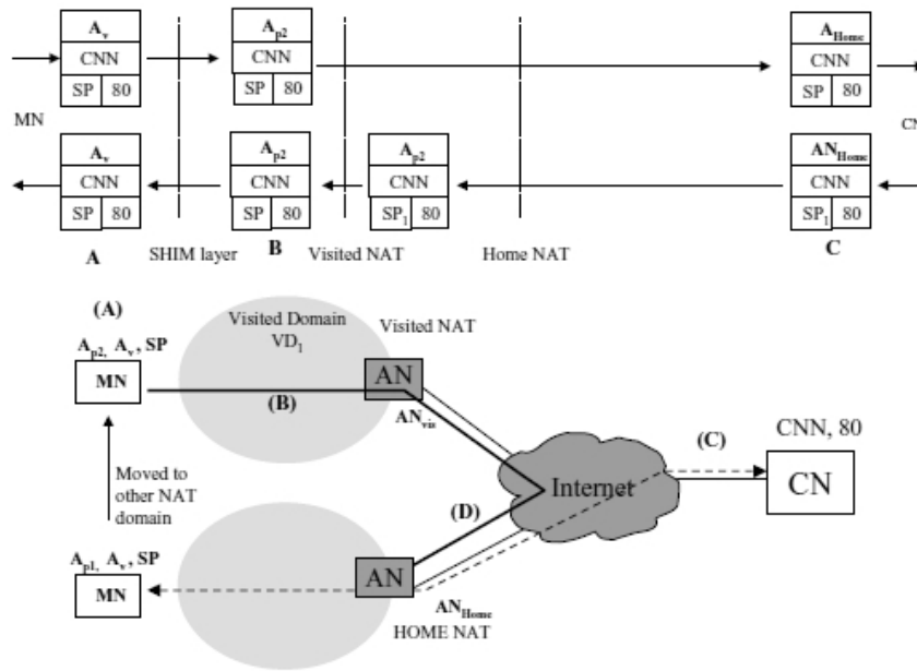
Figura 5.7: Mobilidade entre diferentes domínios, preservando as conexões no nível de Transporte. (fonte: [Buddhikot et al. 2005])
