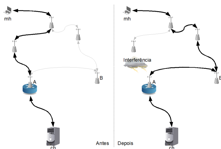
Figura 3.1: Exemplo de uma mudança de rota causada por problemas de conectividade.
