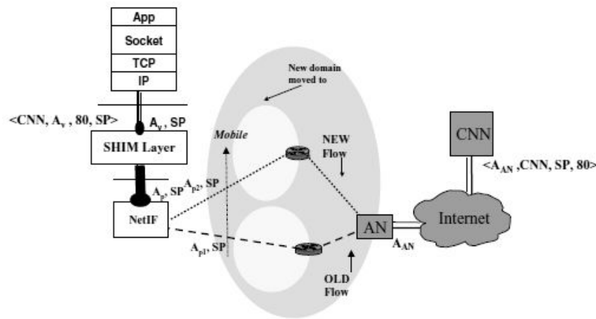
Figura 5.6: Suporte a mobilidade intra-domínio. (fonte: [Buddhikot et al. 2005])
