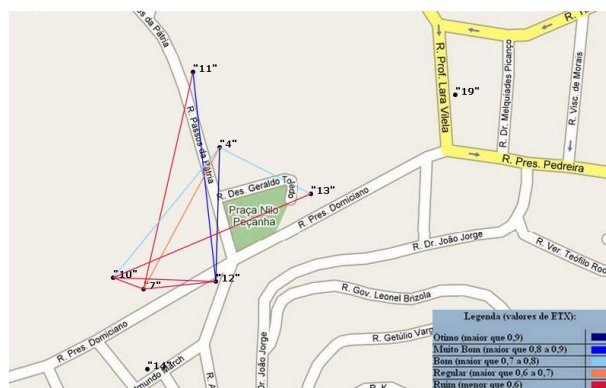
Figura 4.2: Imagem da topologia da rede Remesh produzida pela ferramenta.
