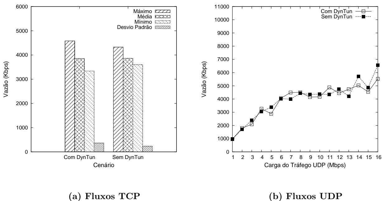
Figura 3.8: Demonstração do baixo impacto da solução sobre diferentes fluxos de dados.
