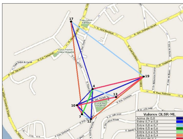
Figura 3.4: Visualização da topologia externa utilizada nos testes.
