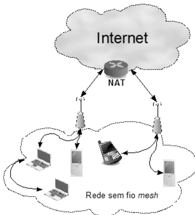
Figura 5.11: Um único gateway com NAT atende a todos os gateways da rede mesh
