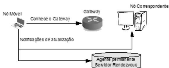
Figura 6.1: Classe Ia: O dispositivo móvel controla a sua mobilidade.
