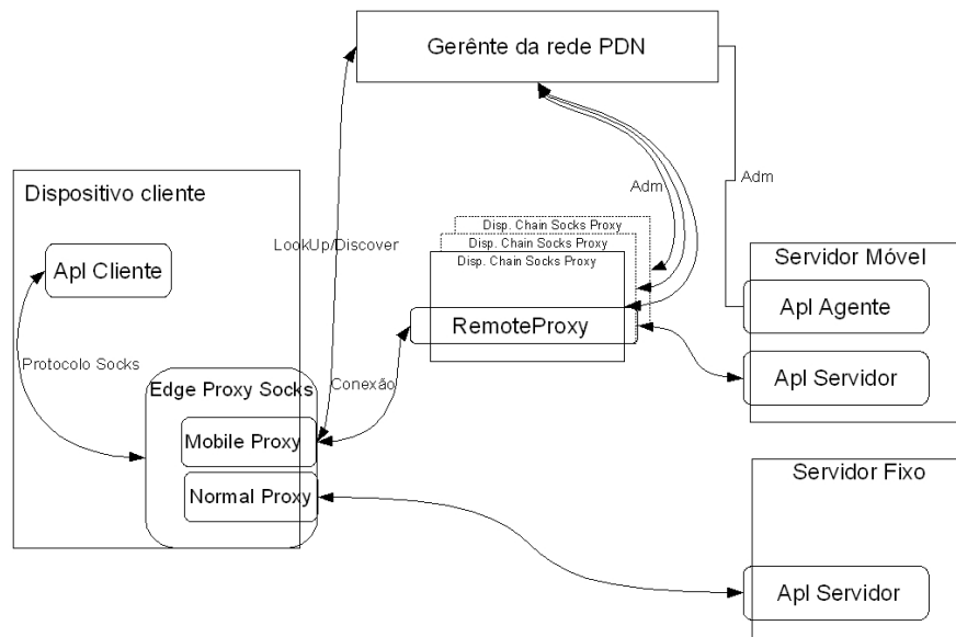
Figura 6.4: Arquitetura do Mproxy
