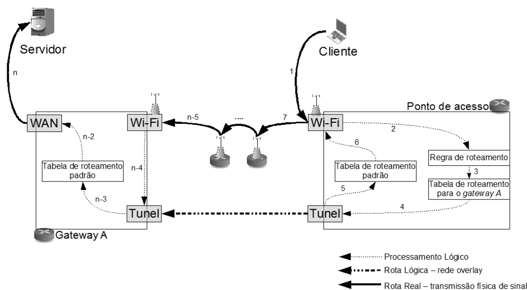
Figura 3.5: Roteamento com DynTun.
