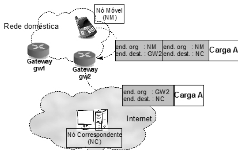
Figura 5.12: Todos os gateways realizam NAT; Técnica de tunelamento é necessária.
