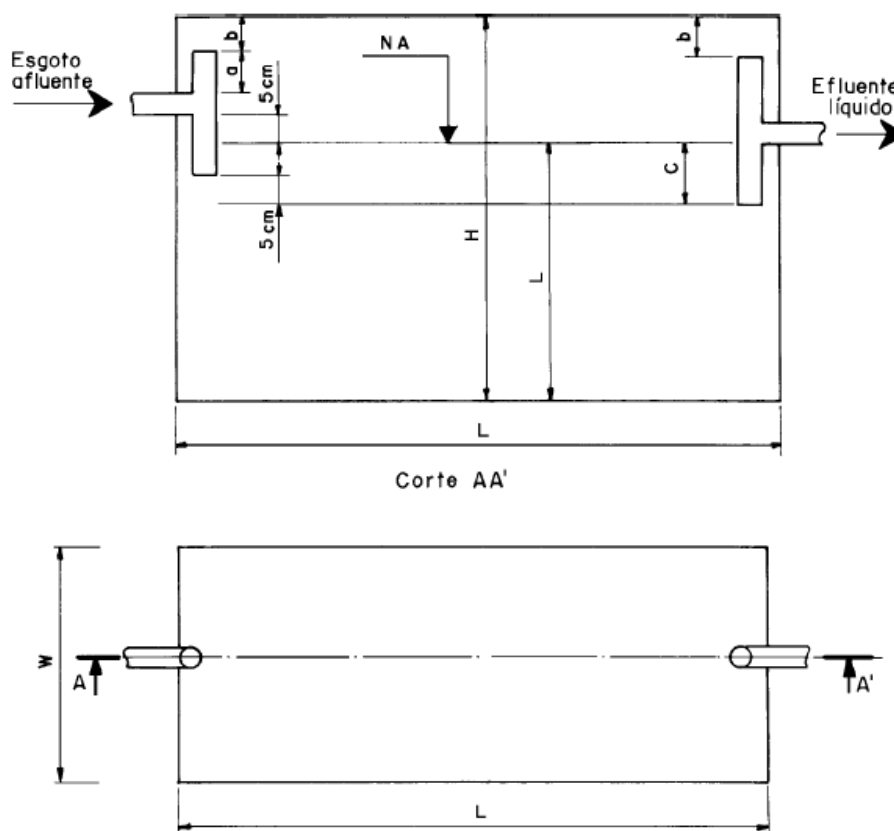
FIGURA 3.3 - DETALHES E DIMENSÕES DE UM TS DE CÂMARA ÚNICA
