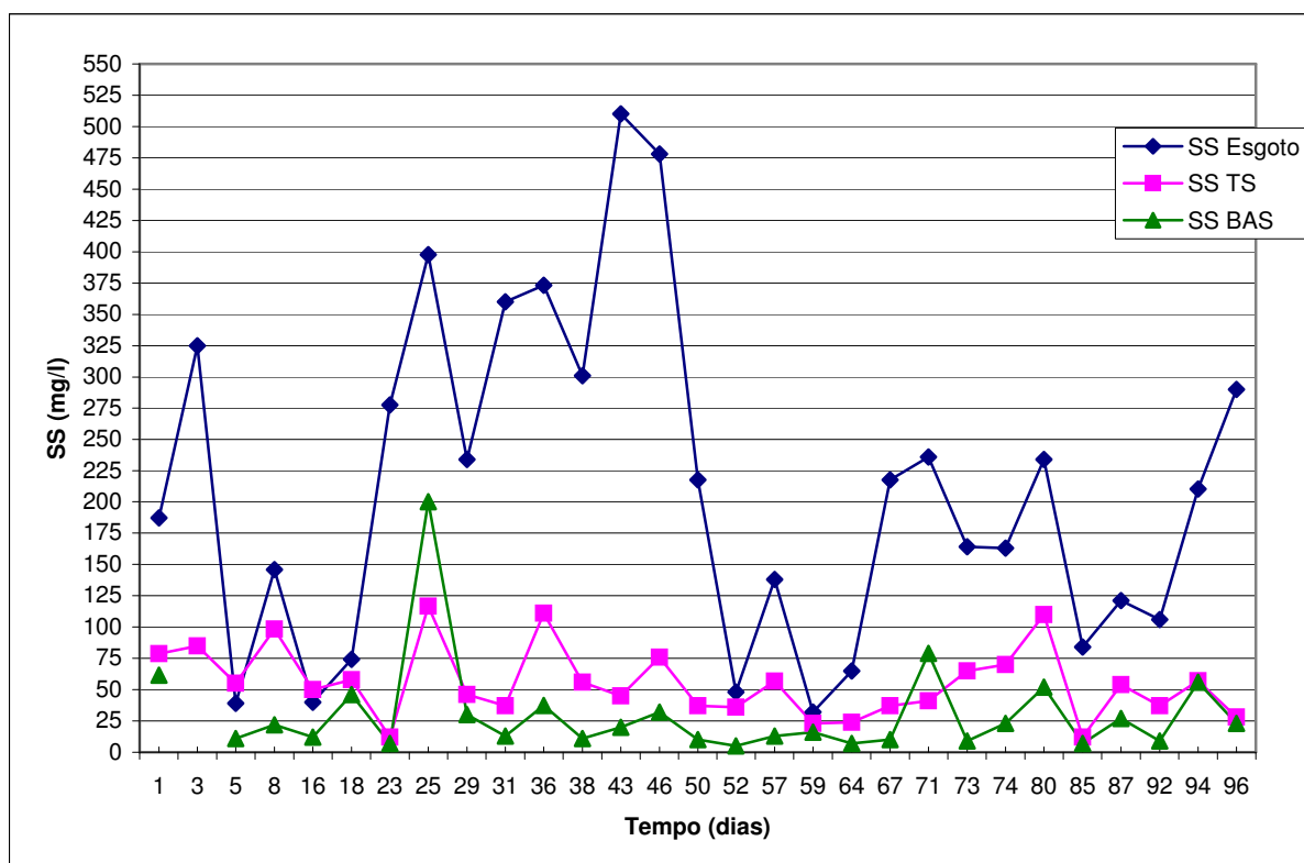
GRÁFICO 5.42 - MONITORAMENTO DE SS NO SISTEMA TS+BAS
