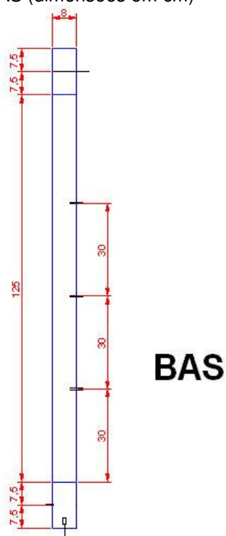
FIGURA 4.8 - PROJETO DA UNIDADE BAS (dimensões em cm)
