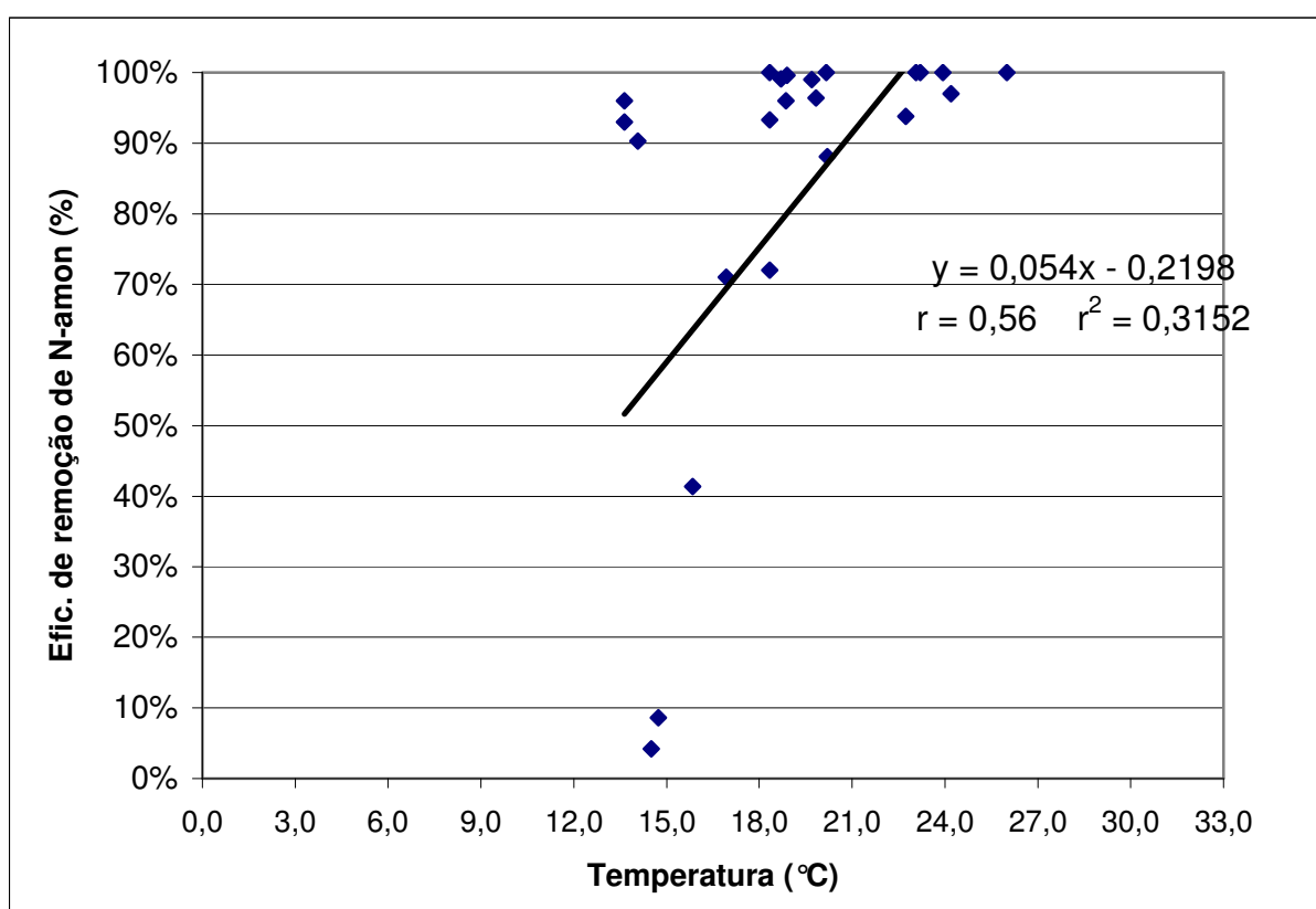
GRÁFICO 5.60 - CORRELAÇÃO ENTRE A TEMPERATURA E A EFICIÊNCIA DE REMOÇÃO DE N-AMON NA UNIDADE BAS
