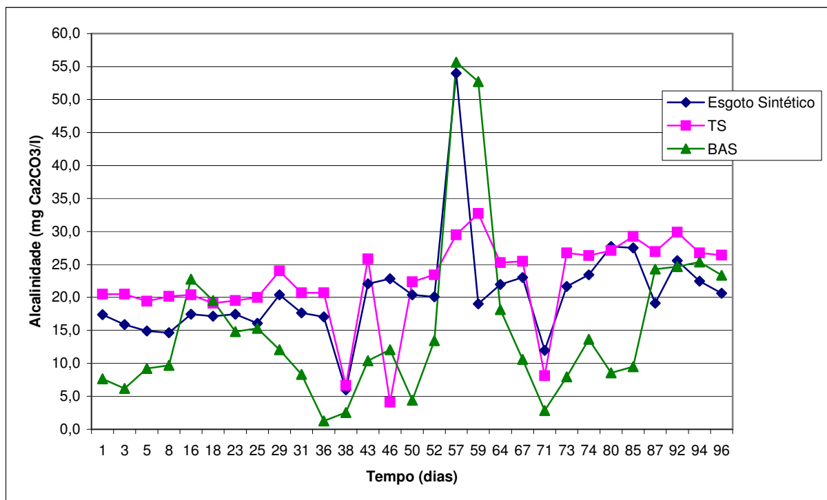
GRÁFICO 5.56 - MONITORAMENTO DA ALCALINIDADE NO SISTEMA TS+BAS
