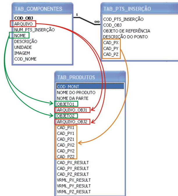
Figura 46: Relacionamento da tabela de componentes e da tabela de pontos de inserção. Fonte: a autora.
