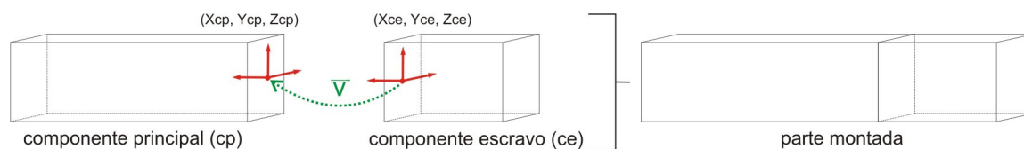
Figura 64: Movimento de translação do componente escravo até o componente principal. Fonte: A autora.
