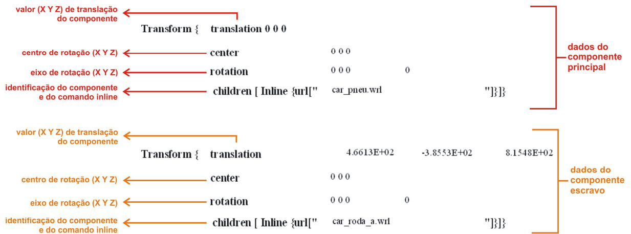
Figura 61: Descrição dos dados de montagem no relatório de montagem.
