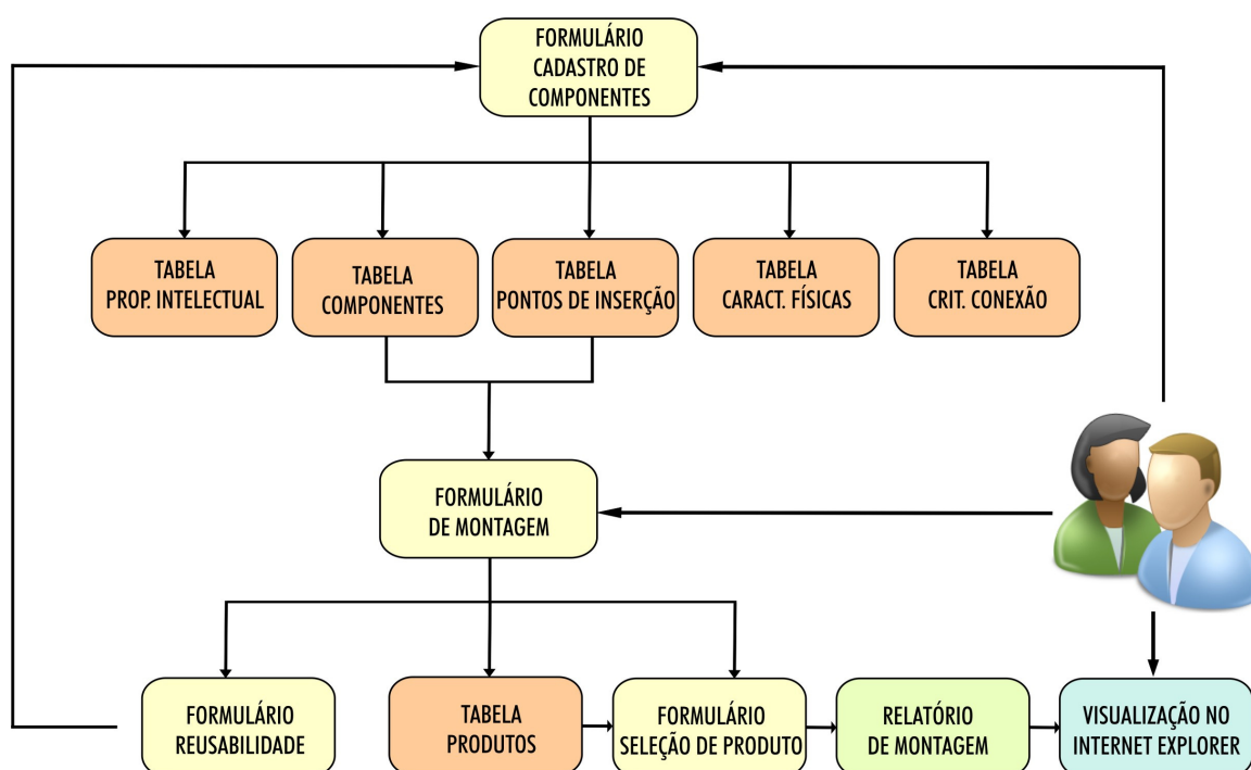
Figura 74: Diagrama de funcionamento do aplicativo dvPro . Fonte: a autora.
