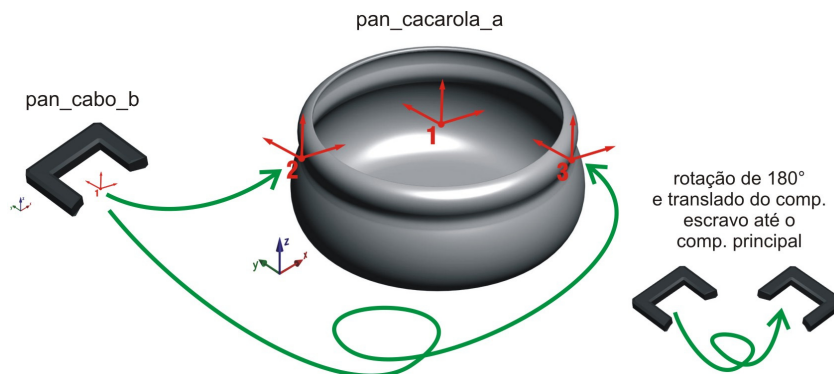
Figura 90: Esquema de rotação dos componentes para a correta montagem. Fonte: a autora.
