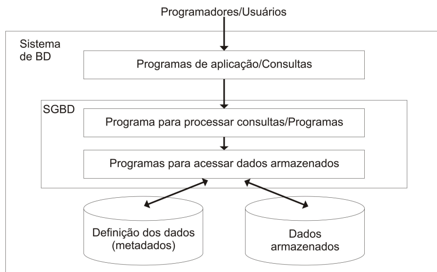
Figura 25: Ambiente de um Sistema de BD Fonte: Elmasri et al. (1989)
