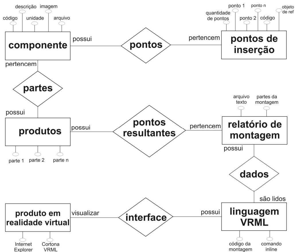
Figura 40: Modelo conceitual do banco de dados proposto.
