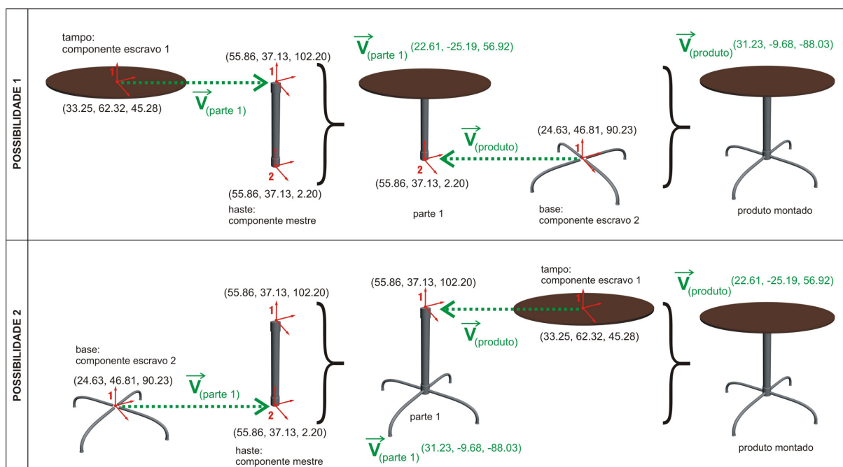
Figura 69: Exemplo de duas possibilidades de montagem de um mesmo produto.
