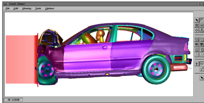
Figura 9: Simulação de colisão com protótipo virtual. Fonte: http://www.vis.uni-stuttgart.de/~frisch/h/diss.htm .
