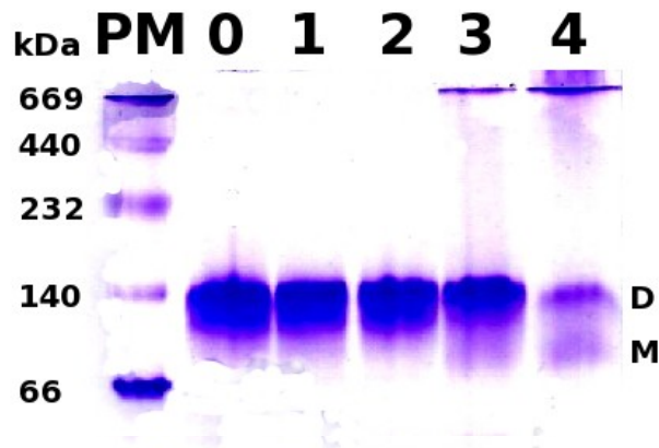
Figura 24. Desnaturalização de hRXR \alpha \Delta AB do Pico 2 por uréia acompanhada por PAGE. Gel de gradiente nativo 8-25% de hRXR \alpha \Delta AB incubada em uréia. As colunas 0, 1, 2, 3 e 4 indicam, respectivamente, a concentração molar de uréia, 0 M, 1 M, 2 M, 3 M e 4 M.
