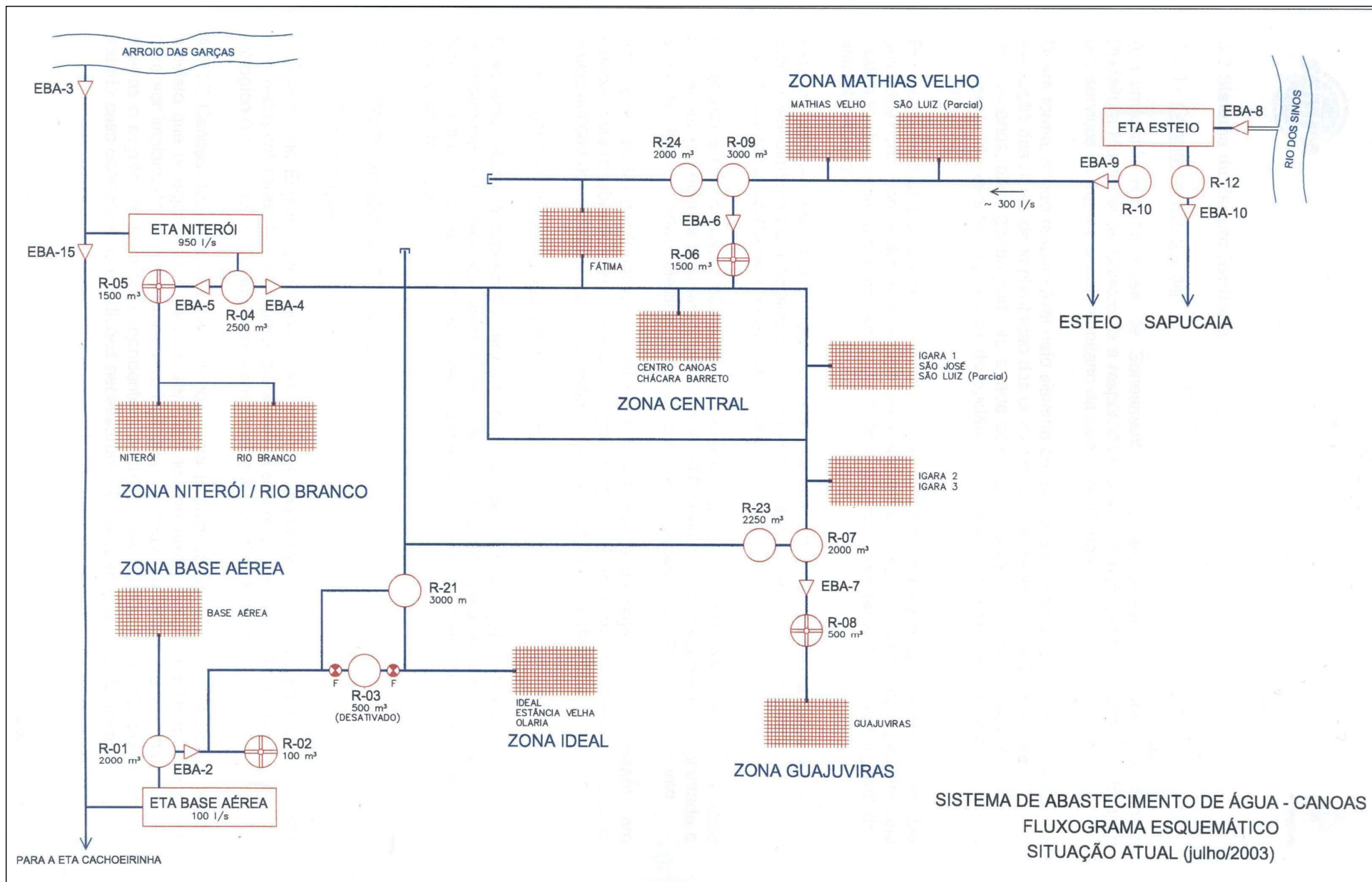
Figura 10: Diagrama de captação e abastecimento de água em Canoas – RS. (Fonte: Secretaria Municipal de Preservação Ambiental / Set.2003).
