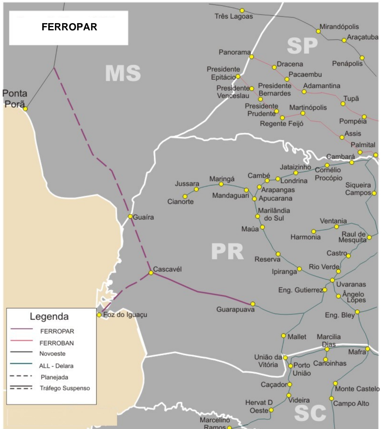
Figura 31 – Traçado da malha ferroviária da Ferrovias Paranaense S.A.
