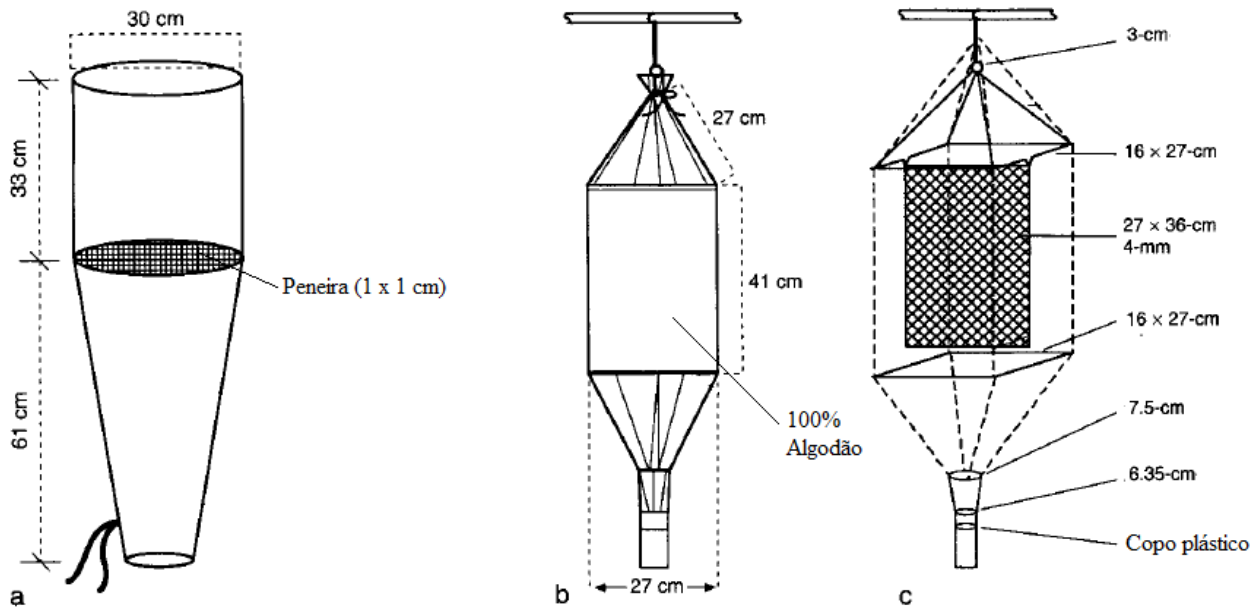
Figura 3 - (a) reconstituição da peneira para serrapilheira, (b) dimensões externas da “mini-Winkler” e (c) reconstituição interna da “mini-Winkler” (adaptado de Delabie 2000)
