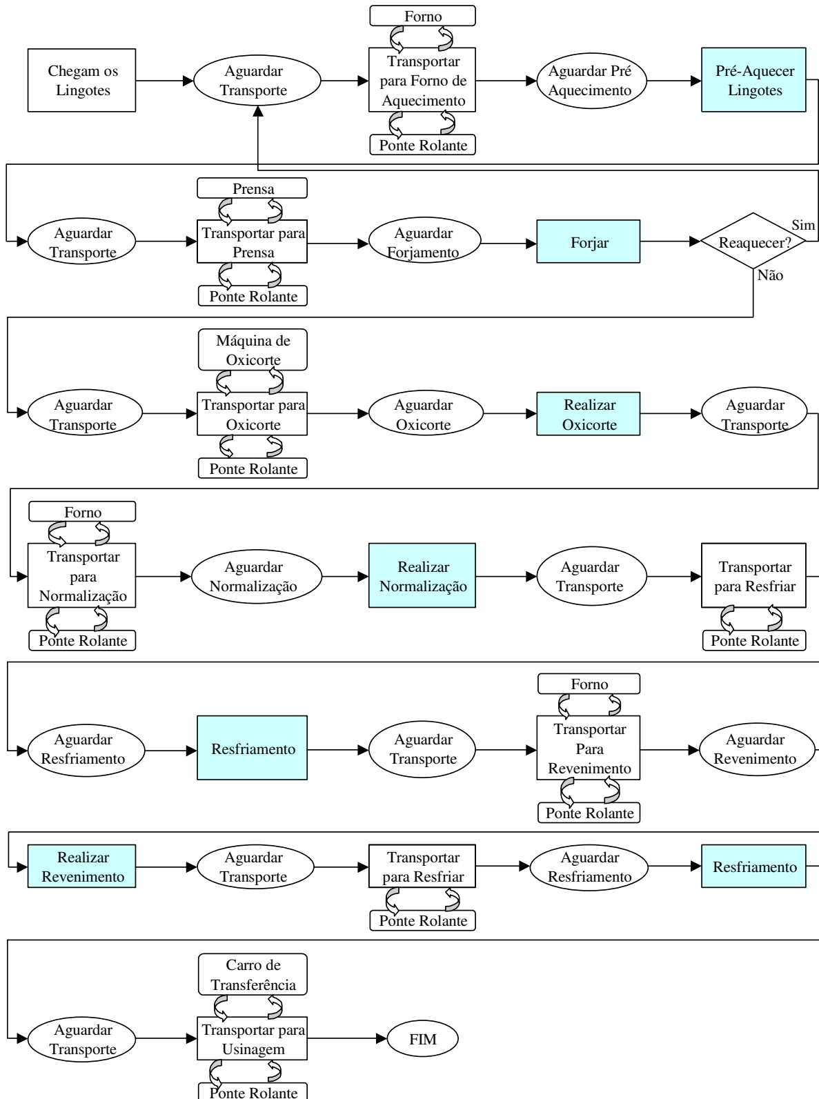
Figura 21 – Modelo conceitual completo
