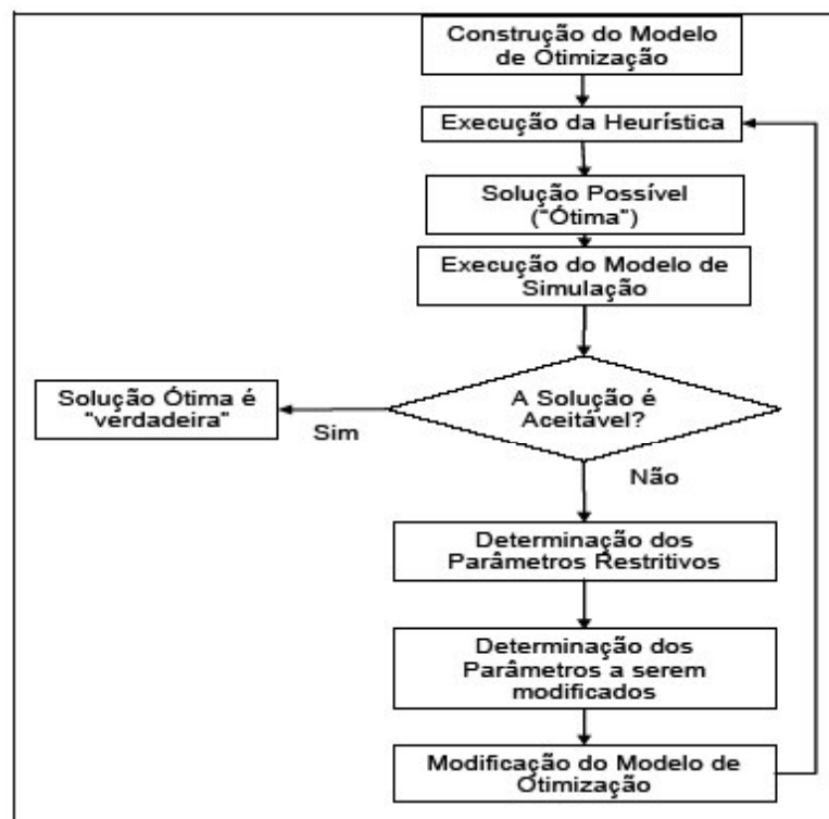
Figura 6 - Método proposto por Morito et al. (1999)
