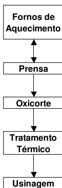
Figura 19 – Fluxo de Processo da Forjaria
