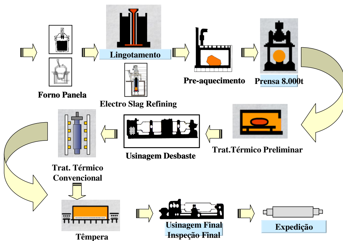
Figura 17 – Processo de fabricação de cilindros de encosto
