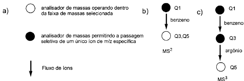
Figura 11: (a) Representação dos símbolos usados em um experimento (b) MS^2 e (c) MS^3
