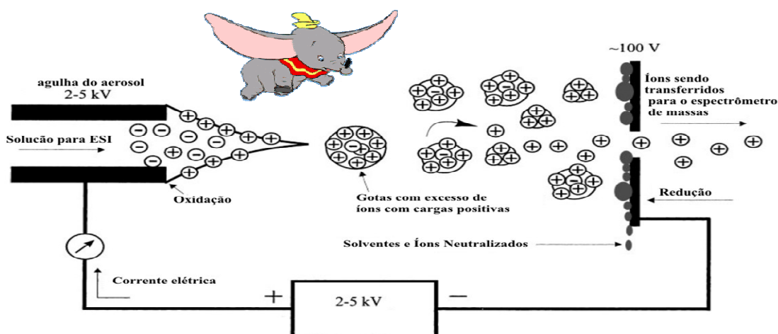
Figura 5. Ionização Electrospray (ESI): Transferência de íons da solução para a fase gasosa.
