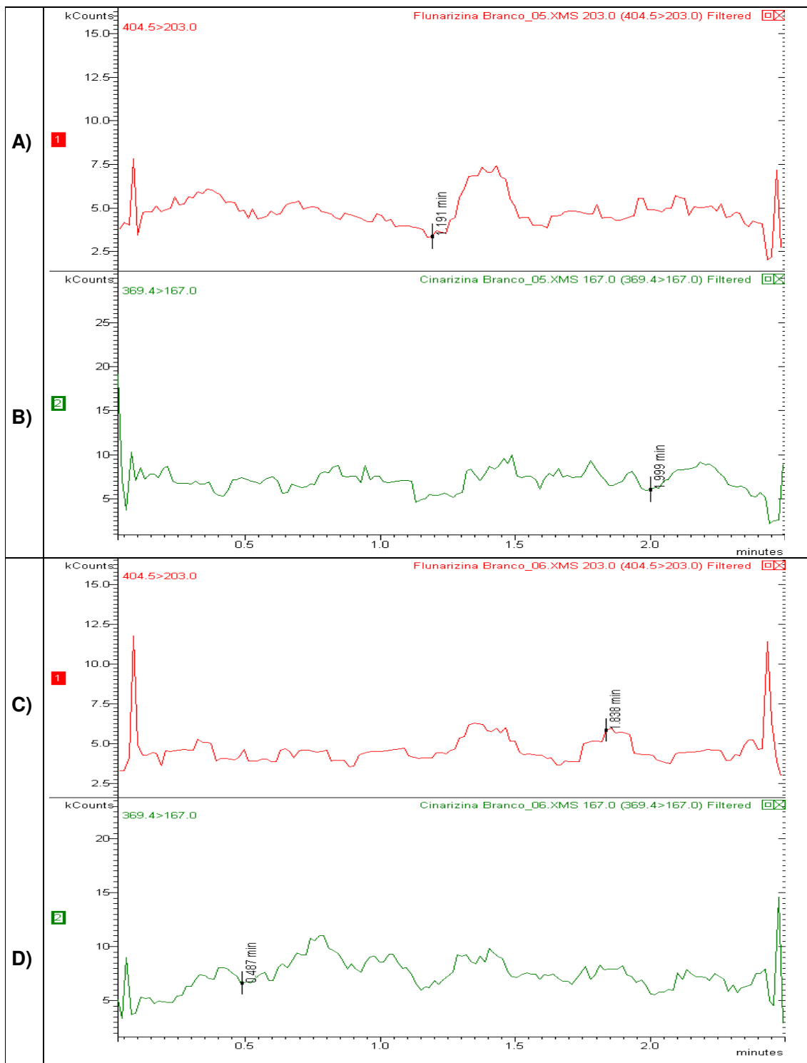
Figura 20: Cromatograma do plasma branco lipêmico (A,B), referente ao branco do analito, referente ao branco do padrão interno. Cromatograma do plasma branco Hemolisado (C,D), referente ao branco do analito, referente ao branco do padrão interno.
