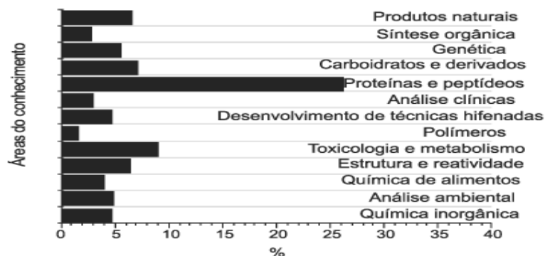
Figura 8. Utilização da espectrometria de massas em diferentes áreas do conhecimento (CROTTI, 2006).
