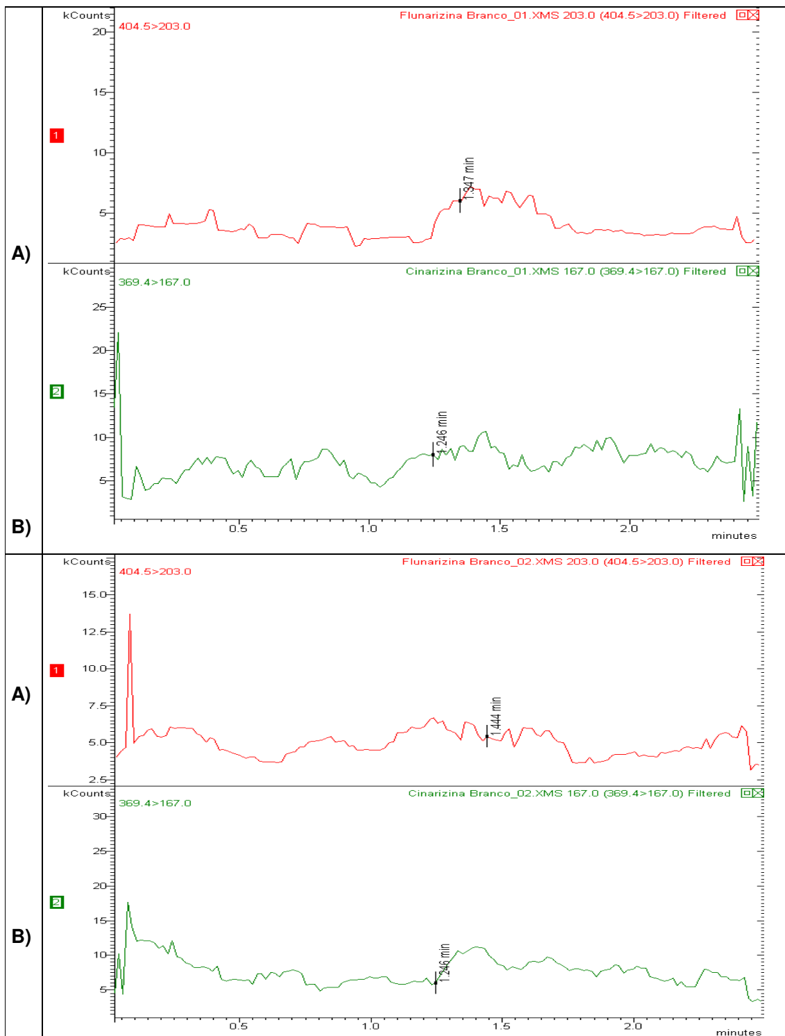
Figura 18: Cromatograma de amostras de plasma branco normal, referente ao analito e ao padrão interno, demonstrando que não existe interferência em nenhum dos canais.
