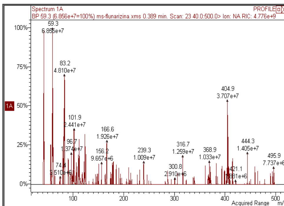
Figura15. Espectro de massas da Flunarizina em modo MS
