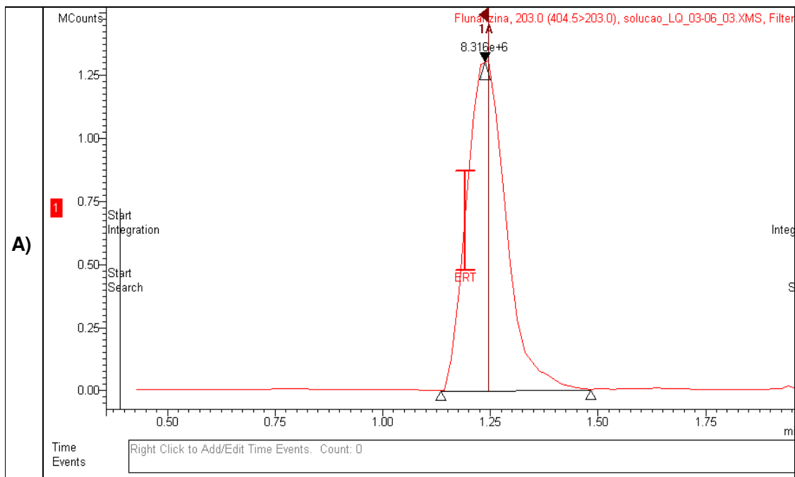
Figura 21: A) Cromatograma referente à Solução de Flunarizina 0,3 ng/mL (LQ).
