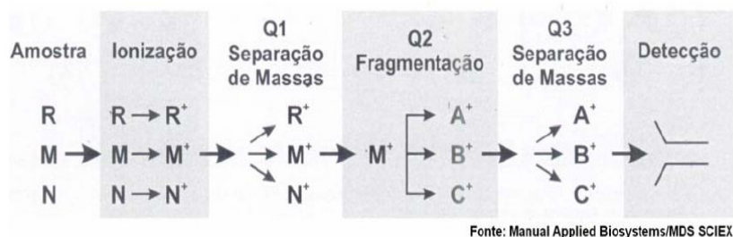
Figura 9. Esquema analítico de um espectrômetro de massas triploquadrupolo.
