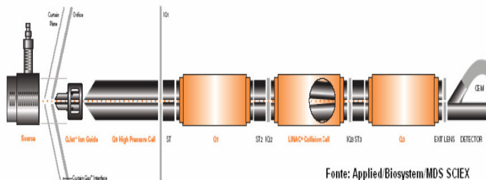
Figura 10. Esquema do interior de um de massas triploquadrupolo
