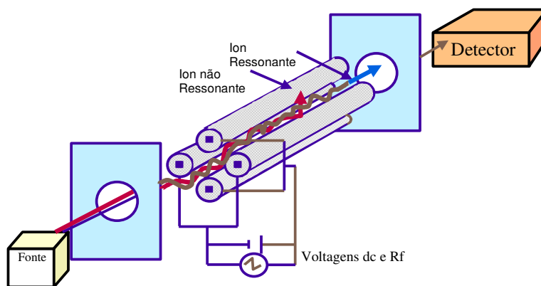
Figura 7. Analisador de Massas Quadrupolar
