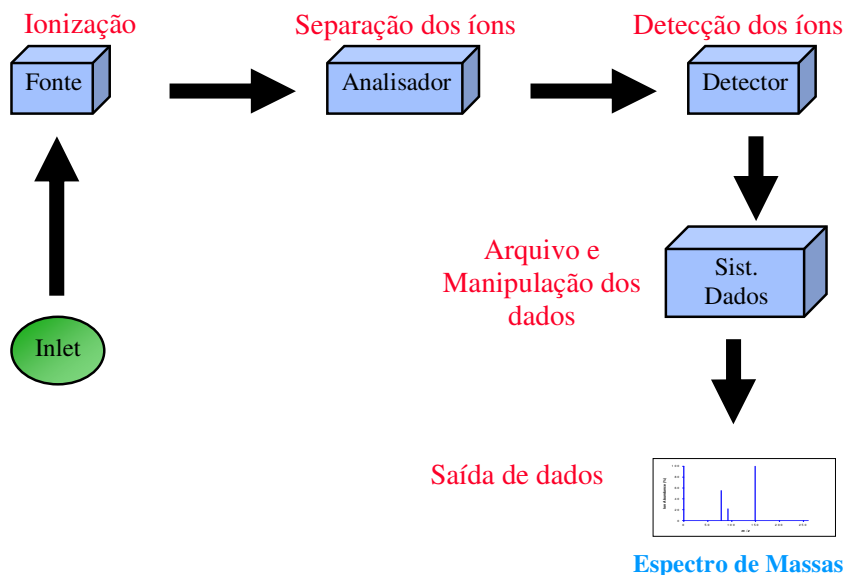
Figura 4. Componentes do Espectrômetro de Massas.
