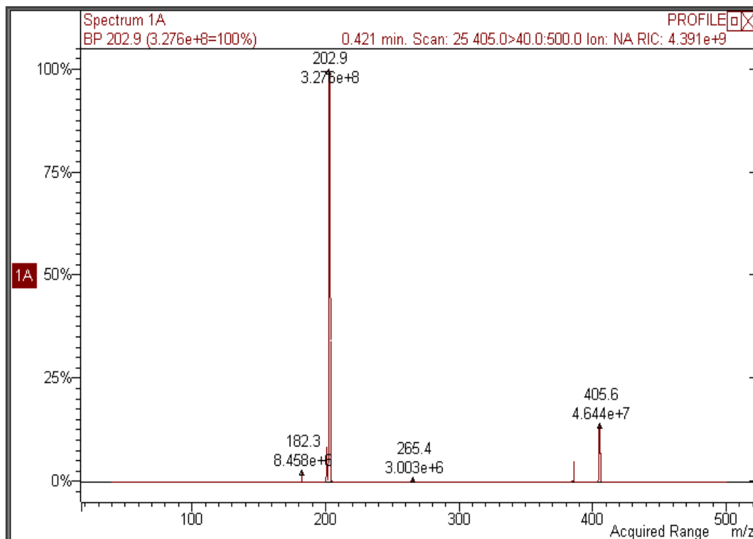
Figura16. Espectro de íons produtos no modo MS/MS
