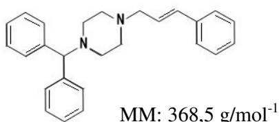
Figura 14. Estrutura Química da Cinarizina (C 26 H 28 N 2 ).
