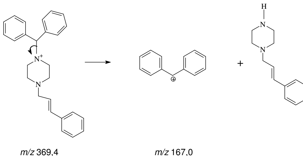
Figura 13. Proposta de fragmentação da Cinarizina.
