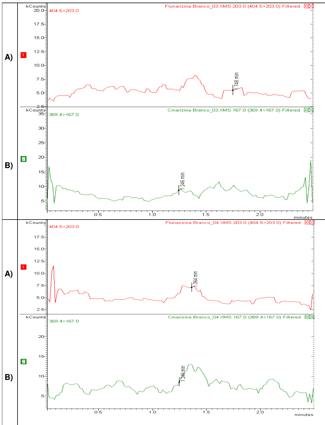
Figura 19: Cromatograma de amostras de plasma branco normal, referente ao analito e ao padrão interno, demonstrando que não existe interferência em nenhum dos canais.
