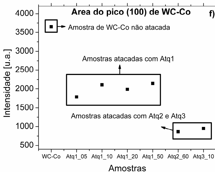
Figura 25: a-e) Apresenta os difratogramas das amostras após o ataque químico para remoção do cobalto; f) mostra as diferenças de intensidade do pico principal do WC-Co após o ataque químico.
