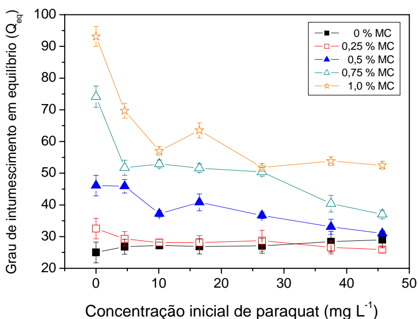
FIGURA 4.15: Dependência dos valores de Q_{eq} em função da concentração inicial de paraquat na solução de intumescimento para hidrogéis (6,0-8,6-M) com M = 0; 0,25; 0,5; 0,75 e 1,0 \% (m/v), [\text{MBAAm}] = 8,6 \mu\text{mol mL}^{-1} e T = 25,0 \pm 0,1 \text{ } ^\circ\text{C} .
