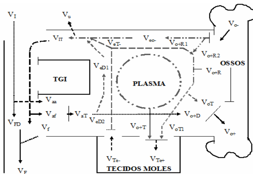
FIGURA 8 Representação esquemática do modelo Fernández modificado por Lopes et al. (2001) usado para o metabolismo de P em cordeiros (Dias, 2006). Trato gastrointestinal (TGI); P ingerido ( V_I ); P total nas fezes ( V_F ); P endógeno fecal ( V_f ); P nas fezes de origem dietética ( V_{FD} ); P na urina ( V_u ); P absorvido de origem alimentar ( V_{aa} ); P de origem endógena que chega ao trato gastrointestinal ( V_{IT} ); P endógeno reabsorvido no trato gastrointestinal ( V_{af} ); P total absorvido ( V_{aT} ); P incorporado no osso ( V_{o+} ); P reabsorvido do osso ( V_{o-} ); P do osso reciclado para osso e tecidos moles ( V_{o+R2} ); P reabsorvido do osso que retorna ao trato gastrointestinal ( V_{e0-} ); P do V_{aT} incorporado no osso ( V_{o+D} ); P incorporado nos tecidos moles ( V_{Te+} ); P reabsorvido dos tecidos moles ( V_{Te-} ); P dos tecidos moles reciclado para osso e tecidos moles ( V_{o+R1} ); P total reciclado para osso e tecidos moles ( V_{o+R} ); P reabsorvido dos tecidos que retorna ao trato gastrointestinal ( V_{eT} ); P do V_{aT} que retorna para o trato gastrointestinal ( V_{eD1} ); P do V_{aT} distribuído para o osso e tecidos moles ( V_{eD2} ); P do V_{o+R} incorporado nos tecidos moles ( V_{oT1} ); P do V_{o+R} reincorporado no osso ( V_{oT2} ). Adaptado de Dias (2006).
