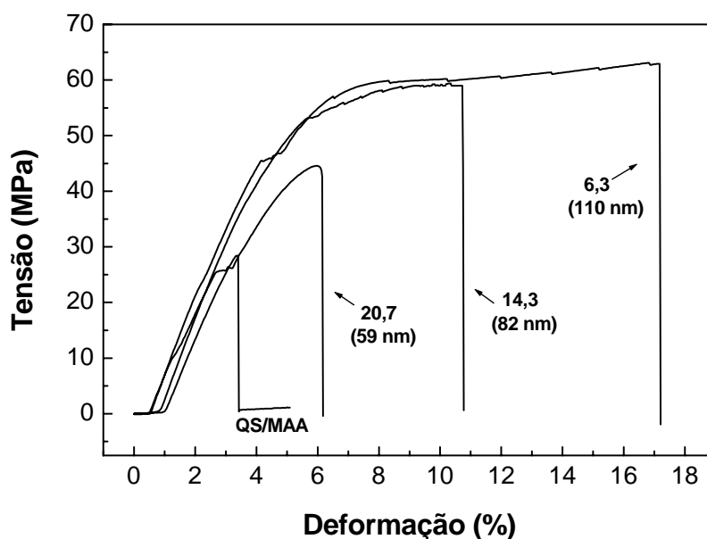
FIGURA 3.3: Curva de tensão-deformação para filmes de HPMC com 6,3 % (110 nm), 14,3% (82 nm) e 20,7% (59 nm) de nanopartículas QS-PMAA adicionadas e com uma curva de filme contendo somente quitosana sem nanopartículas (QS-MAA).
