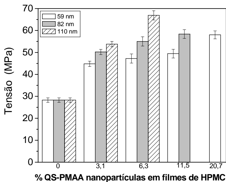
FIGURA 3.4: Tensão dos filmes de HPMC com diferentes concentrações e tamanhos de nanopartículas. Os valores médios são apresentados e as barras indicam os erros das medidas.
