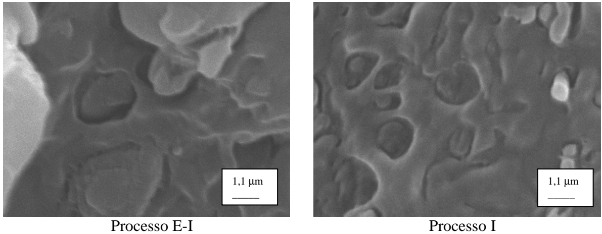
Figura 4.15: Imagens de amostras dos processos E-I e I (originais com 40000x de aumento)
