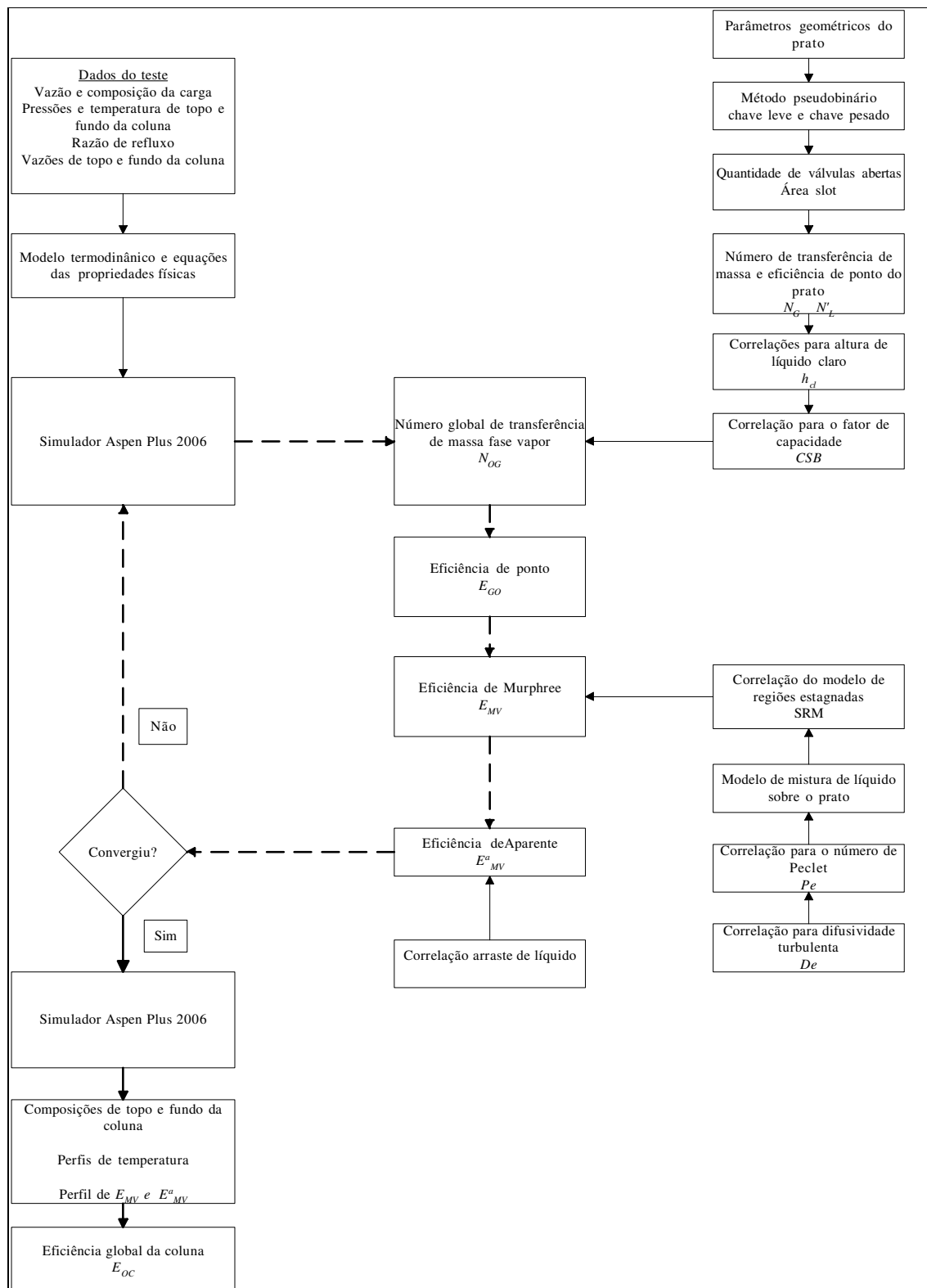
Figura 5.2: Algoritmo para o cálculo da eficiência de prato aparente de Murphree ( E_{MV}^a ) e eficiência global da coluna ( E_{OC} ).
