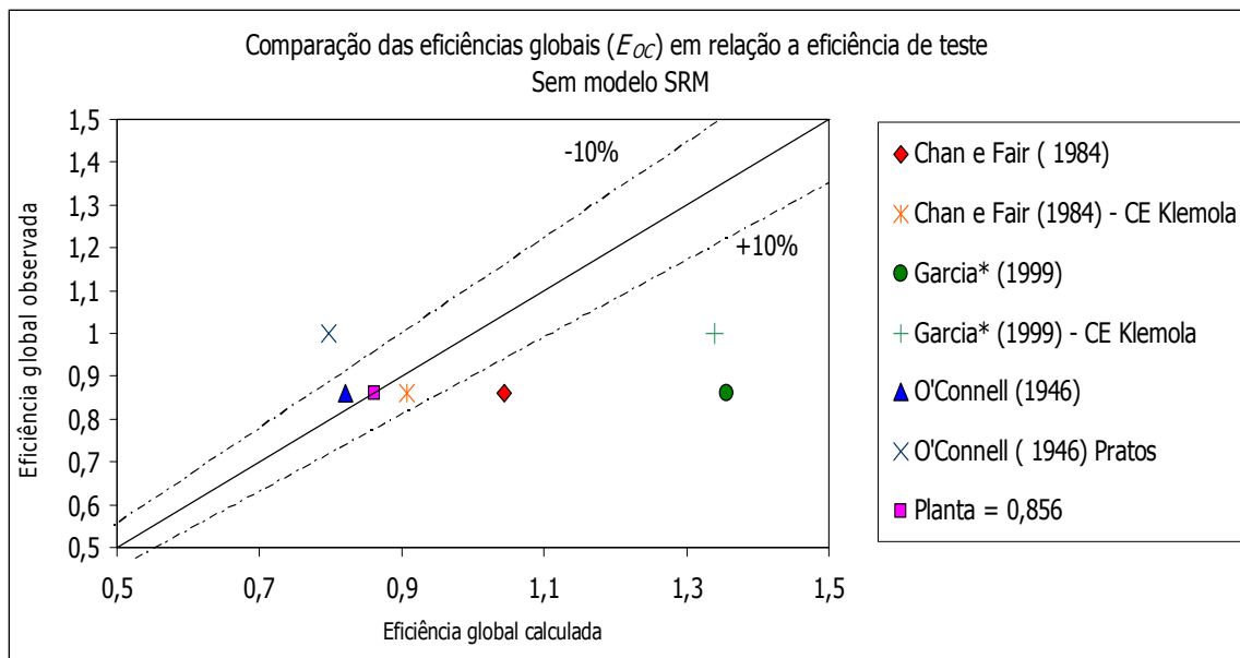
Figura 6.4: Comparação das eficiências globais previstas ( E_{OC} ) em relação à eficiência global ajustada no simulador para a fracionadora de butadieno – sem o modelo SRM.
