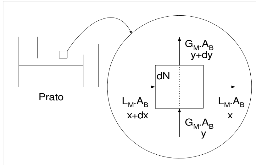
Figura 2.1: Balanço de um componente no elemento diferencial da dispersão.
