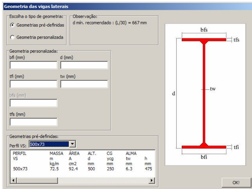
Figura 4.8 - Definição das dimensões das vigas laterais
