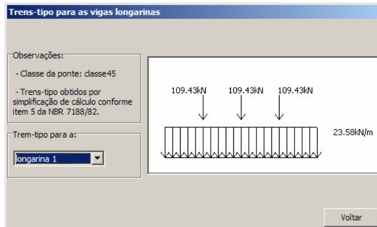
Figura 4.20 - Trem-tipo para a viga principal 1.
