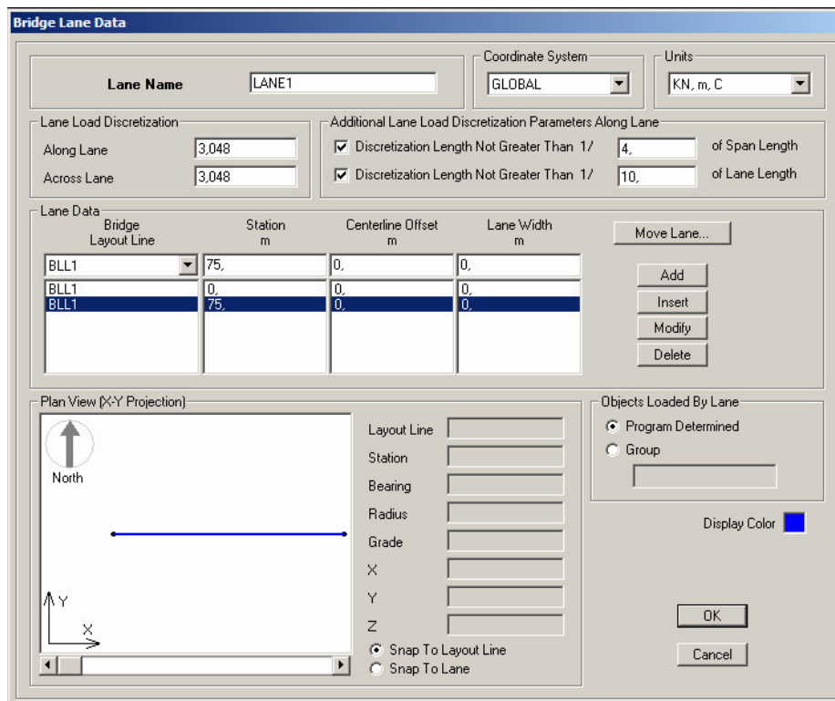
Figura 4.71 - Dados da lane para as vigas principais laterais e centrais.
