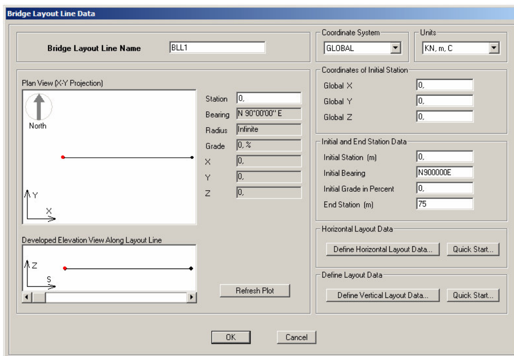
Figura 4.41 - Dados da linha de referência para a ponte.
