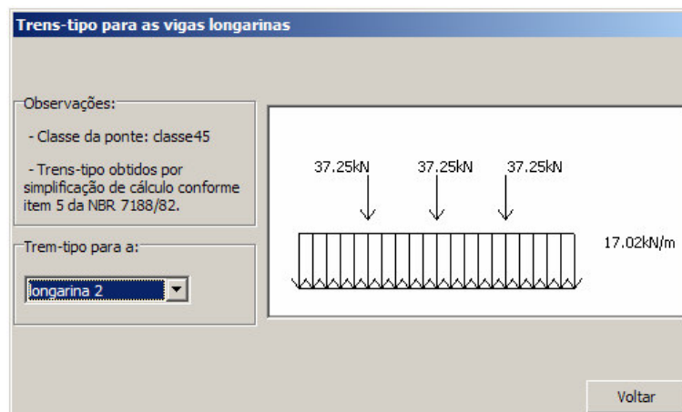
Figura 4.21 - Trem-tipo para a viga principal 2.
