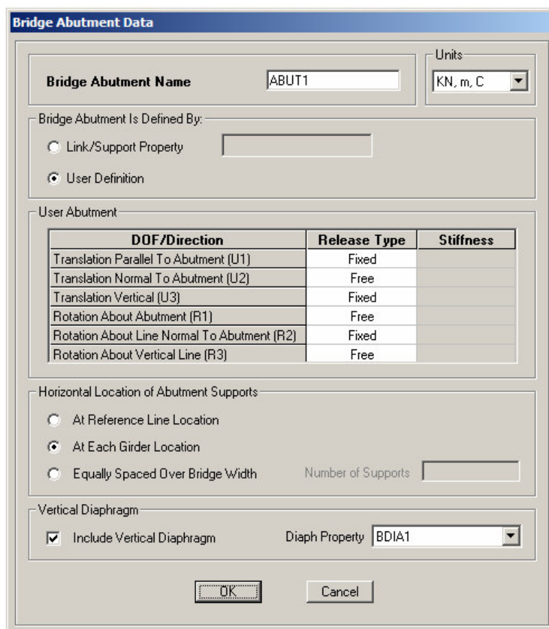
Figura 4.47 - Graus de liberdade a serem liberados/restringidos nos apoios e sua localização.
