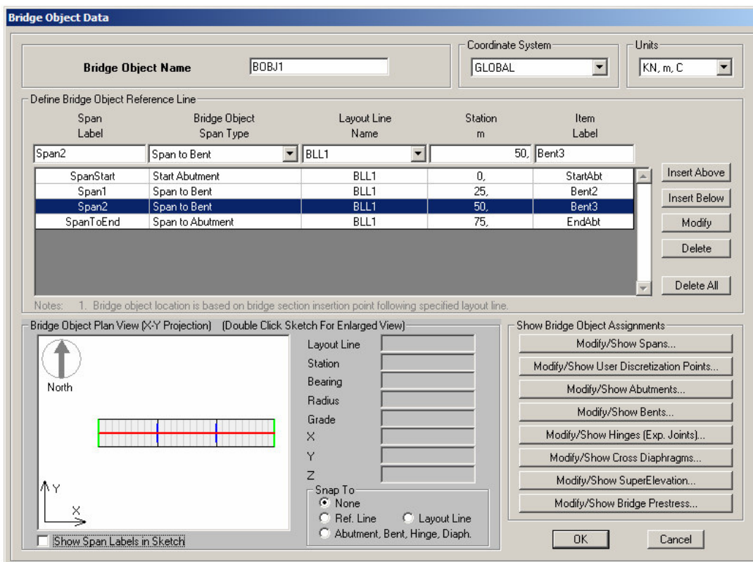
Figura 4.54 - Dados referentes ao posicionamento das cap beams.
