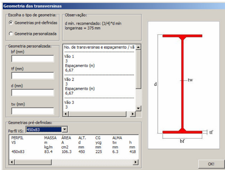
Figura 4.10 - Definição das dimensões das transversinas.
