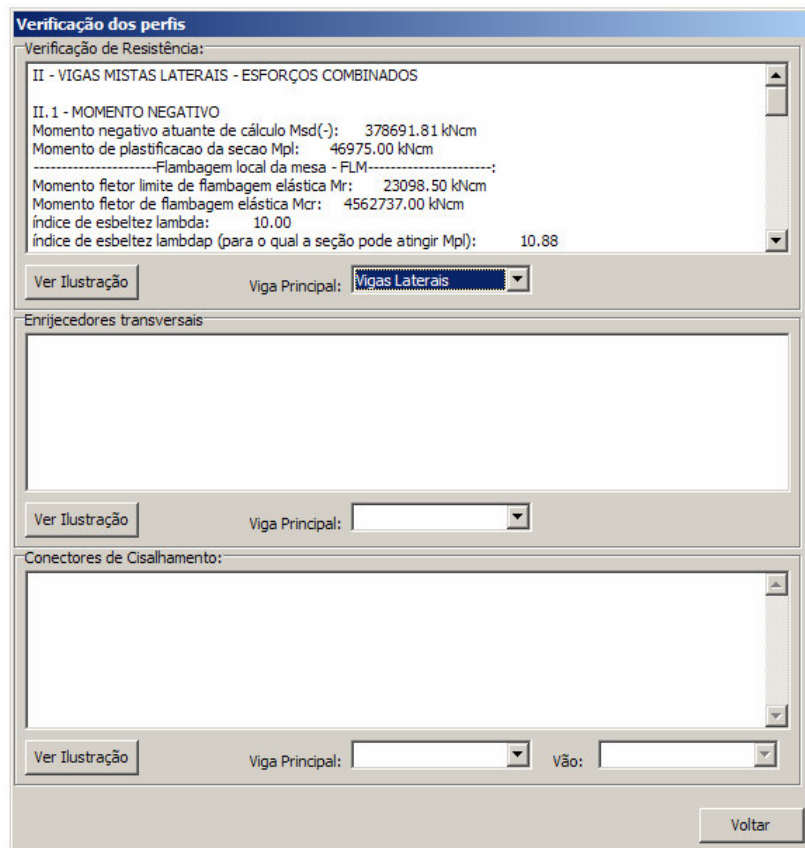
Figura 4.32 - Verificação das vigas mistas laterais aos esforços atuantes de cálculo.
