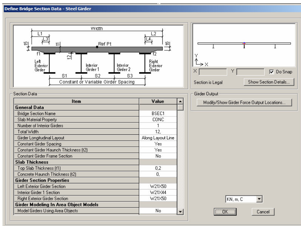
Figura 4.45 - Entrada de dados para seção transversal do tipo steel-girders .
