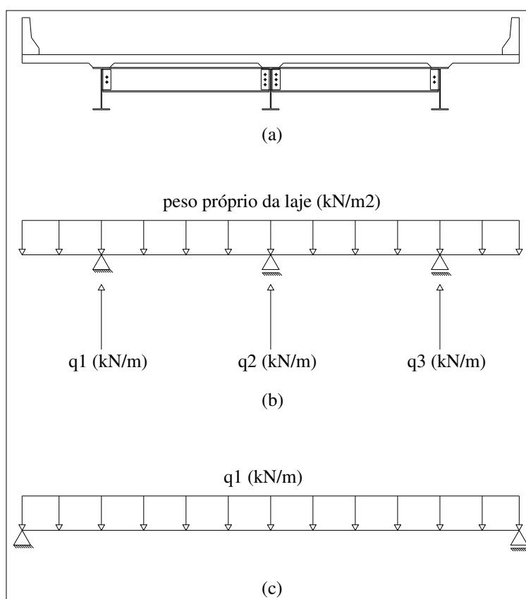
Figura 4.2 - Distribuição de cargas devidas ao peso próprio da laje de concreto e do peso próprio das vigas principais.
