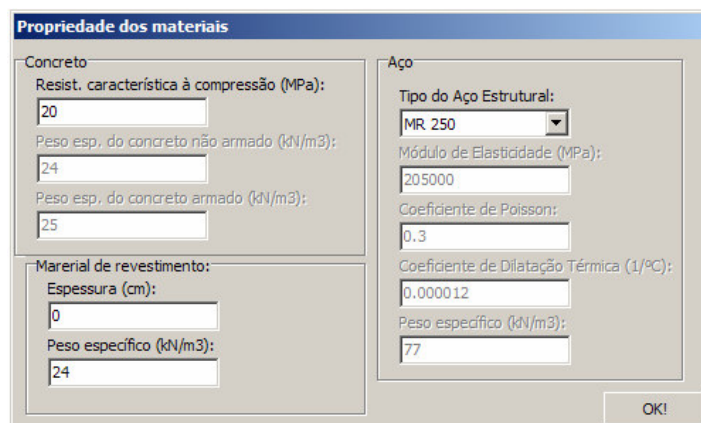
Figura 4.13 - Definição das propriedades físicas dos materiais.
