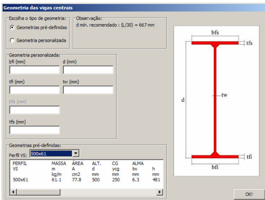
Figura 4.9 - Definição das dimensões das vigas centrais.
