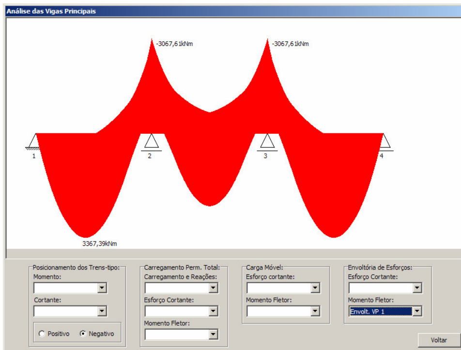
Figura 4.30 - Envoltória de momento fletor devido ao carregamento total para a viga principal 1.
