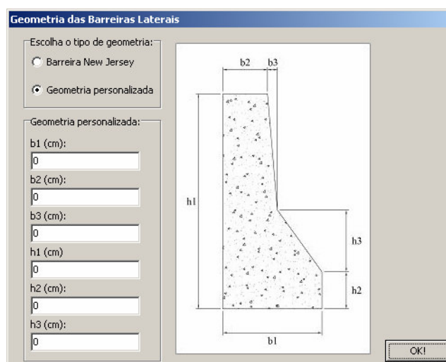
Figura 4.11 - Dimensões das barreiras laterais.
