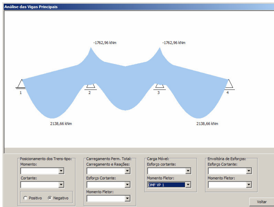
Figura 4.28 - Envolvória de momento fletor devido ao carregamento móvel para a viga principal 1.
