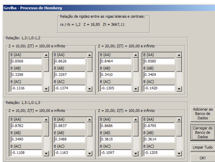
Figura 4.15 - Entrada de dados para a curva de distribuição transversal pelo método de Homberg-Trenks.
