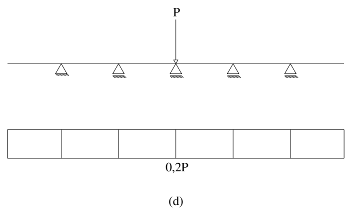
Figura 2.6 - Distribuição de cargas pelo Método da Transversina de Rigidez Infinita.
