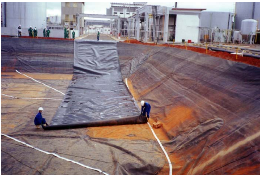
Figura 24 - Colocação do revestimento de PEAD. Fonte: (INB, 2001).
