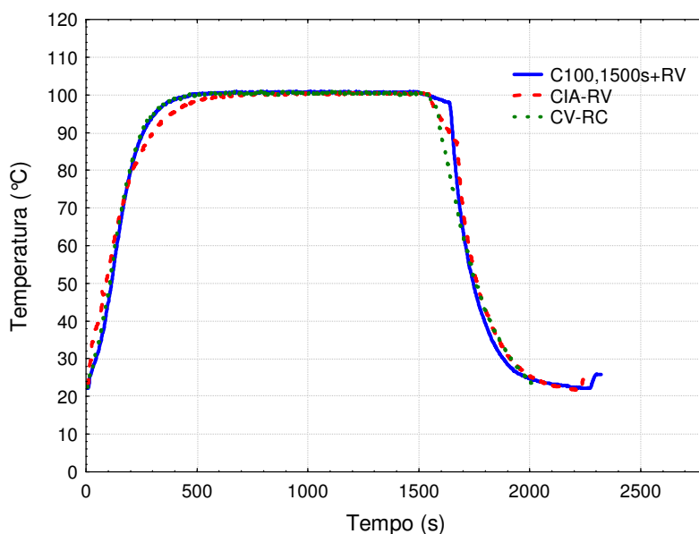
Figura 4.14 Comparativo entre o resfriamento a vácuo (C100,1500s+RV) e em câmara fria (CV-RC) após cozimento a vapor e o resfriamento a vácuo após a drenagem da água de cozimento de cenouras cozidas (CIA) (tempo de cozimento de 1500s).
