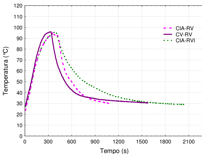
Figura 4.6 Comparativo dos processos integrados de cozimento no vapor e em imersão até as amostras atingirem 90°C seguido de resfriamento a vácuo. CV-RV: Coz. a vapor seguido de resfriamento a vácuo; CIA-RVI: Coz. imerso seguido de resfriamento a vácuo imerso na mesma água do cozimento; CIA-RV: Coz. imerso seguido de resfriamento a vácuo com drenagem da água de cozimento.
