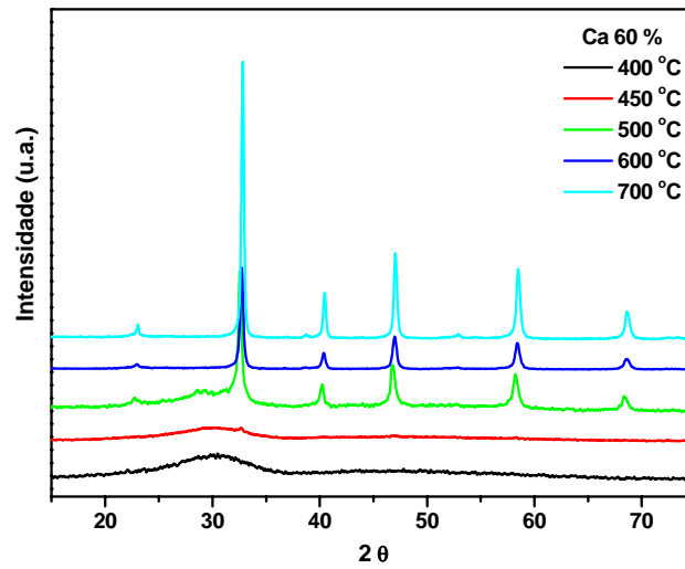
FIGURA 3.5: Difratomogramas obtidos em função da temperatura de calcinação para a amostra Ca 60%.
