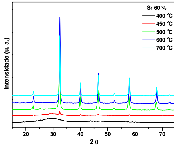
FIGURA 3.4: Difratomogramas obtidos em função da temperatura de calcinação para a amostra Sr 60%.
