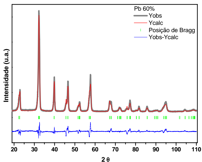
FIGURA 3.12: Difratogramas obtidos através do refinamento pelo método de Rietveld para a amostra Pb 60% calcinada a 700 °C.
