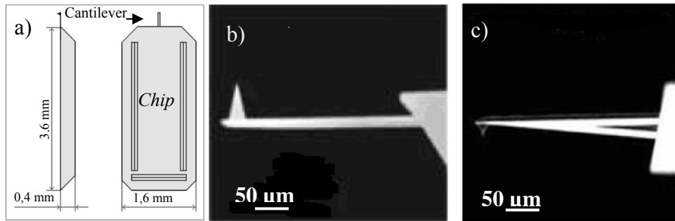
Fig. 2: a) Esquema de chip com cantilever retangular; b) cantilever retangular; c) triangular [6].
