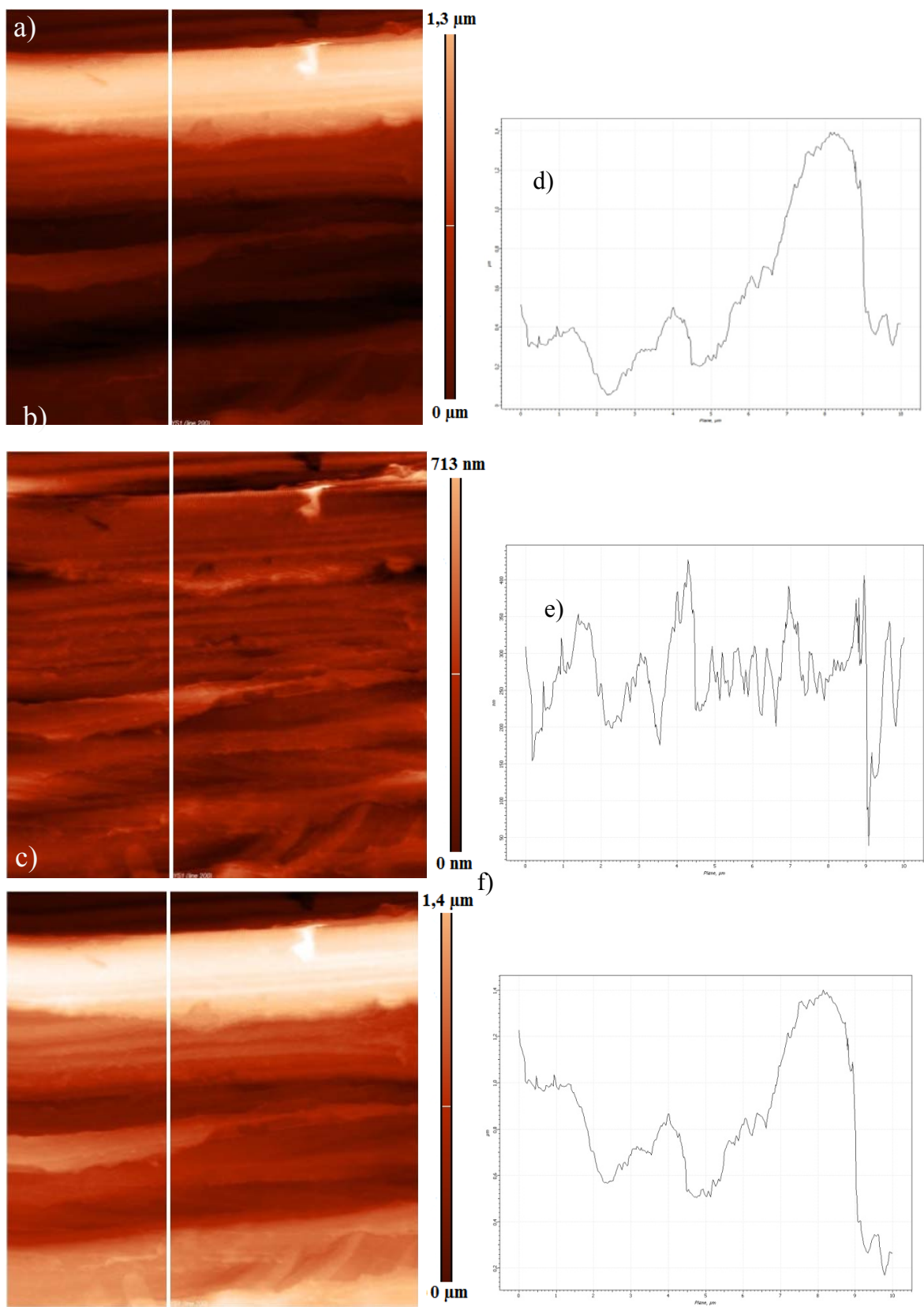
Fig. 28: Imagens topográficas (AFM in-situ ) de (5 \times 5) \mu\text{m}^2 A) imagem sem tratamento; B) imagem com ajuste de Flatten ; C) imagem nivelada. Perfis da linha destacada: D) imagem sem tratamento; E) imagem com ajuste de Flatten e F) imagem nivelada.
