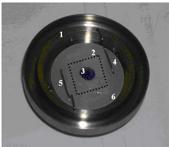
Fig. 20: 1 - Célula líquida; 2 - amostra (destacado pelo pontilhado); 3 - marca posição amostra (marca azul); 4 e 5 - grampos e 6 - porta amostra (pastilha branca).
