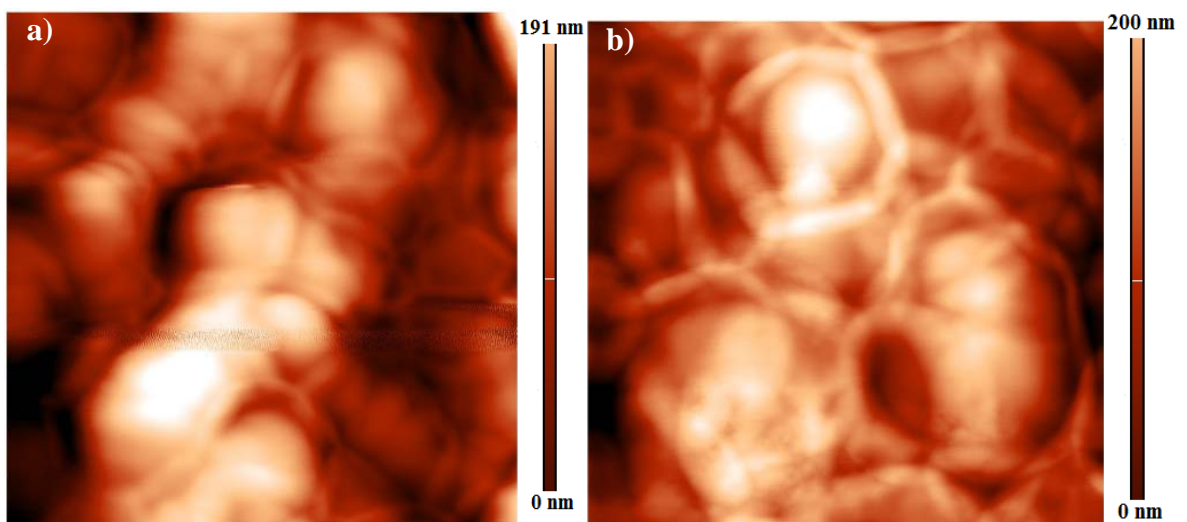
Fig. 40: Nafion Casting Dopado , imagens topográfica (AFM in-situ ) de (2 X 2) \mu\text{m}^2 : a) lado A e b) lado B. É evidente a presença de partículas parcialmente imersa na matriz polimérica.
