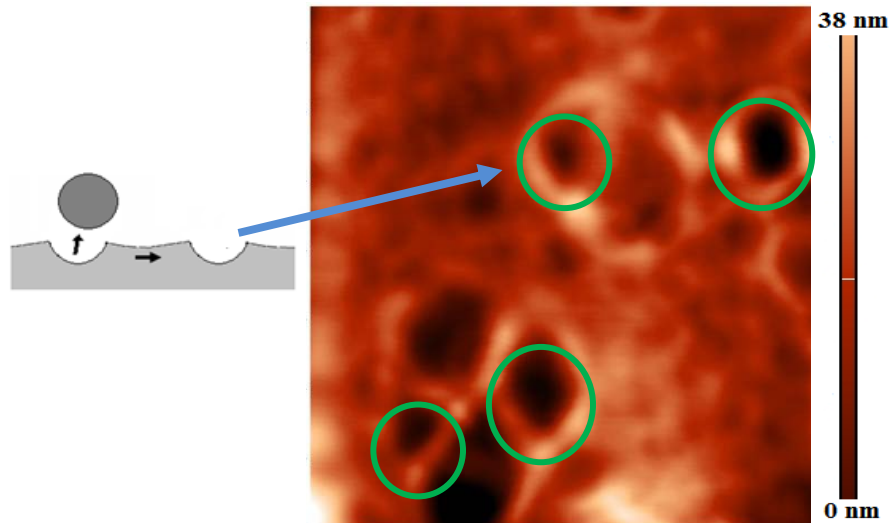
Fig. 38: Nafion Casting Dopado A ) esquema de partícula se despreendendo da superfície, B) imagem topográfica (AFM in-situ ) (1,5 X 1,5) \mu\text{m}^2 . Em destaque os pites (círculos verdes).
