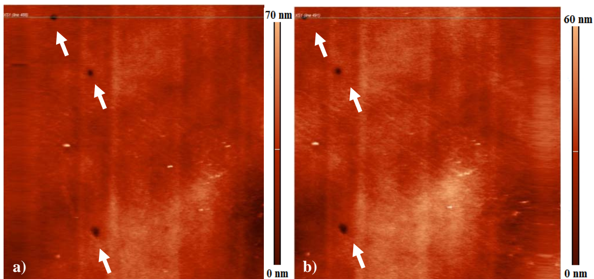
Fig. 27: Imagens topográficas (AFM in-situ ) de (5 \times 5) \mu\text{m}^2 . Imagem em trace (a) transladada para direita em relação a imagem retrace (b).
