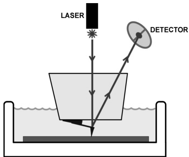
Fig. 14: Esquema ilustrativo do sistema de microscopia de força atômica in-situ vii .
