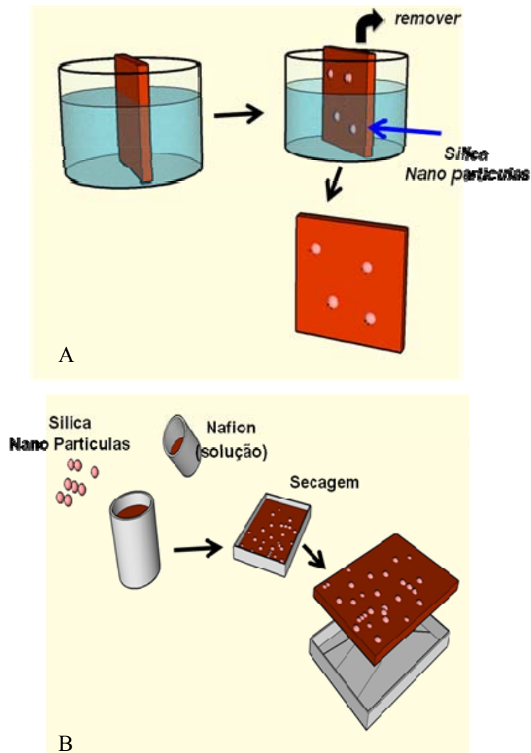
Fig. 17: Ilustração dos métodos de inserção de nanopartículas: a) Sol-gel e b) Casting.
