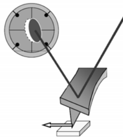
Fig. 5: Força lateral atuando na sonda: representação da mudança de posição lateral do feixe de laser coletado pelo fotodiodo.
