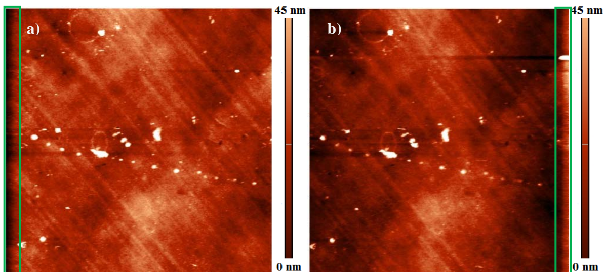
Fig. 26: Imagens topográficas (AFM in-situ ) de (10 \times 10) \mu\text{m}^2 ; efeito de torção do cantilever: a) Faixa lateral (escura) a esquerda na imagem Trace e b) Faixa lateral (clara) a direita na imagem Retrace .
