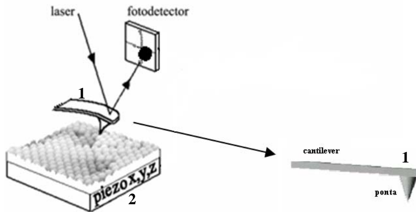
Fig. 1: Diagrama de organização do microscópio de força atômica. 1-sonda; 2- cerâmicas piezelétricas.
