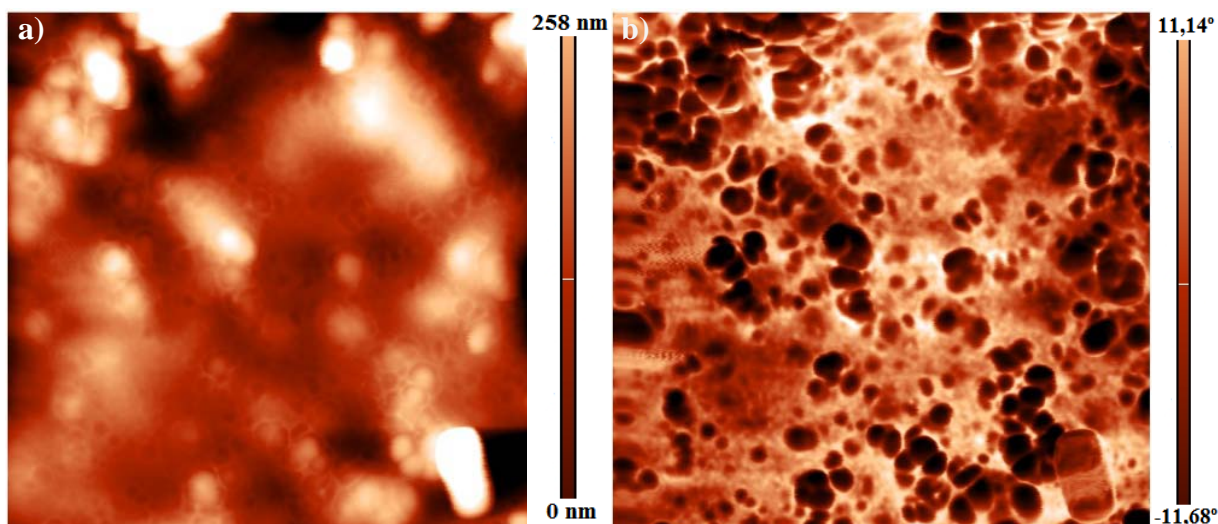
Fig. 37: Nafion Casting Dopado - partículas espalhadas sobre a superfície, imagens (AFM in-situ ) de (10 X 10) \mu\text{m}^2 : a) imagem topográfica e b) imagem de contraste de fase. Na imagem de contraste de fase (b) observa-se destaque das partículas na matriz polimérica.
