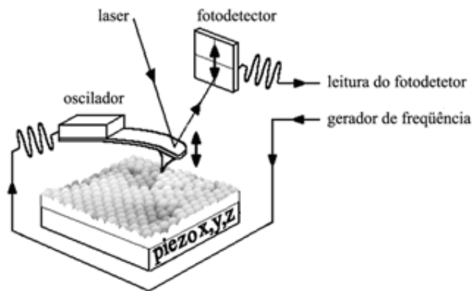
Fig. 11: Sonda oscilando sobre amostra. As senóides representam: a oscilação do piezo oscilador e do sinal detectado no fotodiodo (feixe laser refletido) [9].
