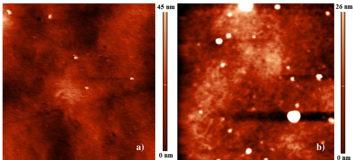
Fig. 33: Imagens topográficas (AFM in-stiu ) ( 5 \times 5 ) \mu\text{m}^2 : A) Nafion Comercial lado A e B) Nafion Comercial Dopado . Na imagem dopada é observada maior quantidade de partículas.
