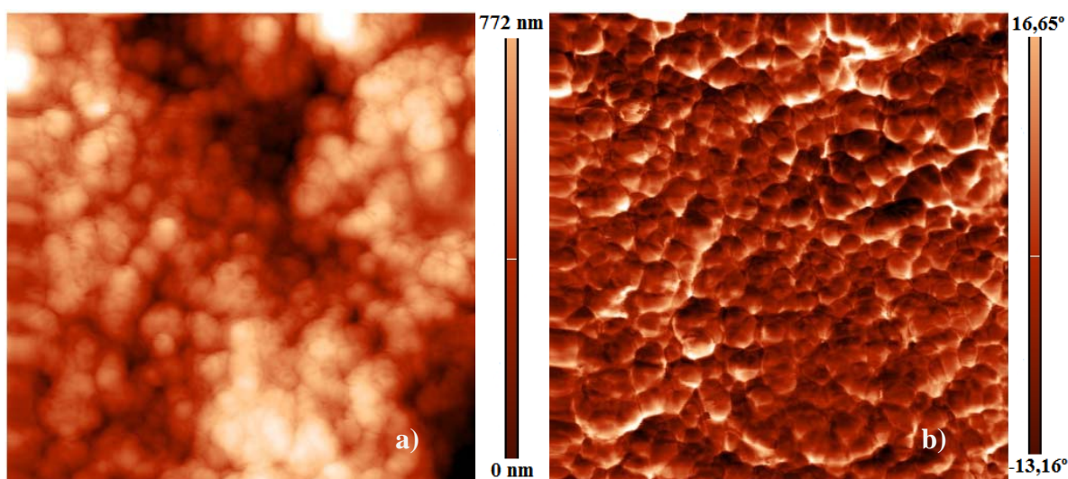
Fig. 36: Nafion Casting Dopado - , superfície recoberta por partículas, imagens de (10 \times 10) \mu\text{m}^2 : A) imagem topográfica e B) imagem de contraste de fase. (AFM in-situ ).
