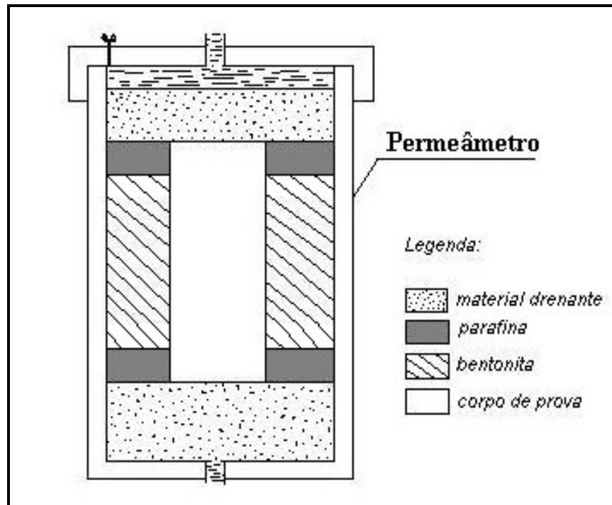
Figura 3.6: Esquema da montagem do ensaio de permeabilidade.
