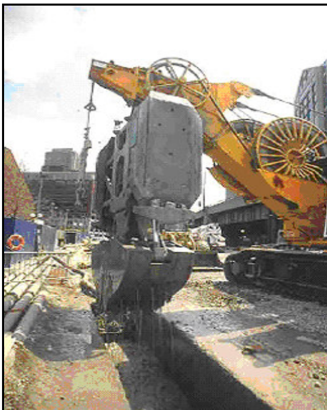
Figura 2.10: Equipamento para escavação da trincheira (Zulritz, 1994).
