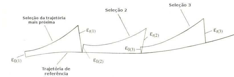
FIG. 3.6: Cálculo do Expoente de Lyapunov Médio
