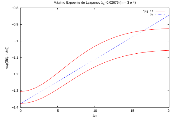
(f) Máximo Expoente de Lyapunov \lambda_1
