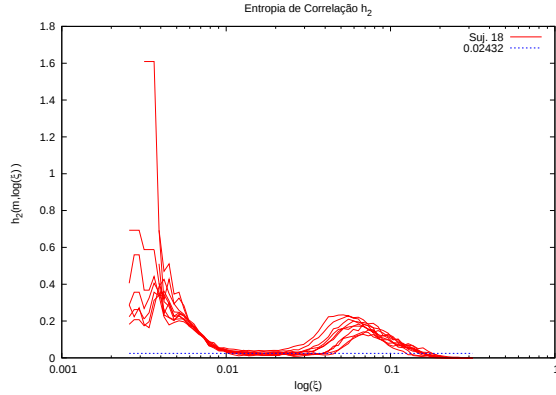
(e) Estimação de h_2 ( m=11,12,\dots,20 )
