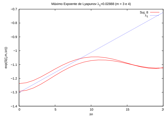
(f) Máximo Expoente de Lyapunov \lambda_1
