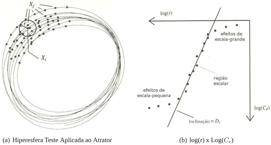
FIG. 3.4: Determinando a Dimensão de Correlação D_2
