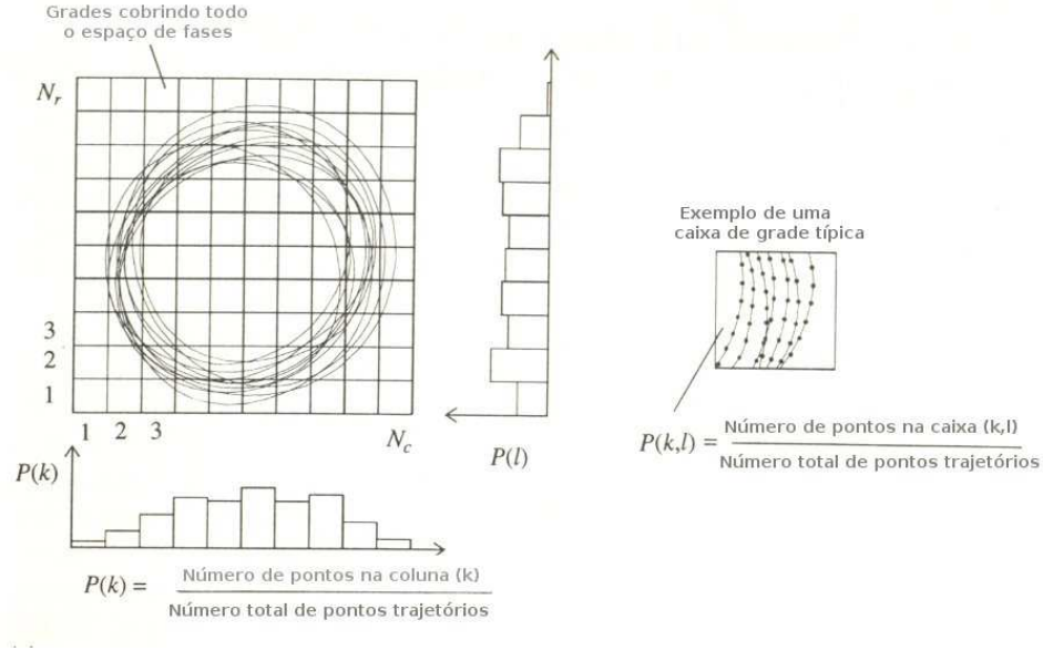
(a) Cálculo da Informação Mútua
