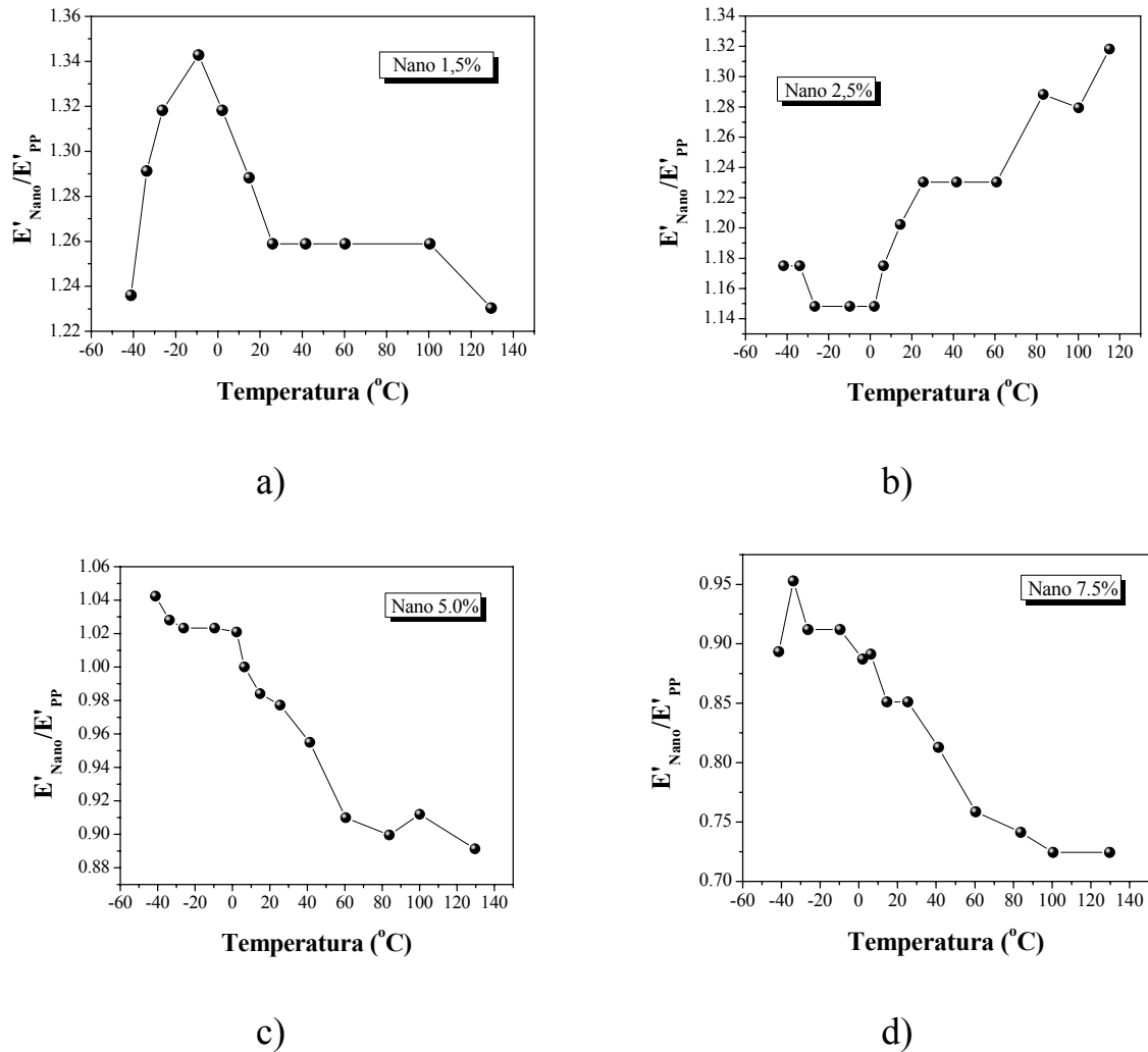
FIGURA 5. 21. Curvas dos módulos elásticos relativos ( E'_{Nano}/E'_{PP} ) em função da temperatura dos nanocompósitos com concentrações de: a) Nano 1,5%; b) Nano 2,5%; c) Nano 5,0% e d) Nano 7,5% de argila organofílica.
