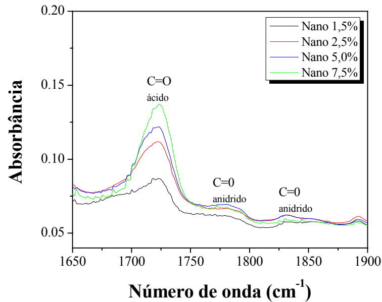
FIGURA 5. 10. Espectros de absorção na região do infravermelho, ampliado na região 1650\text{-}1900\text{ cm}^{-1} , das amostras de diversas concentrações.
