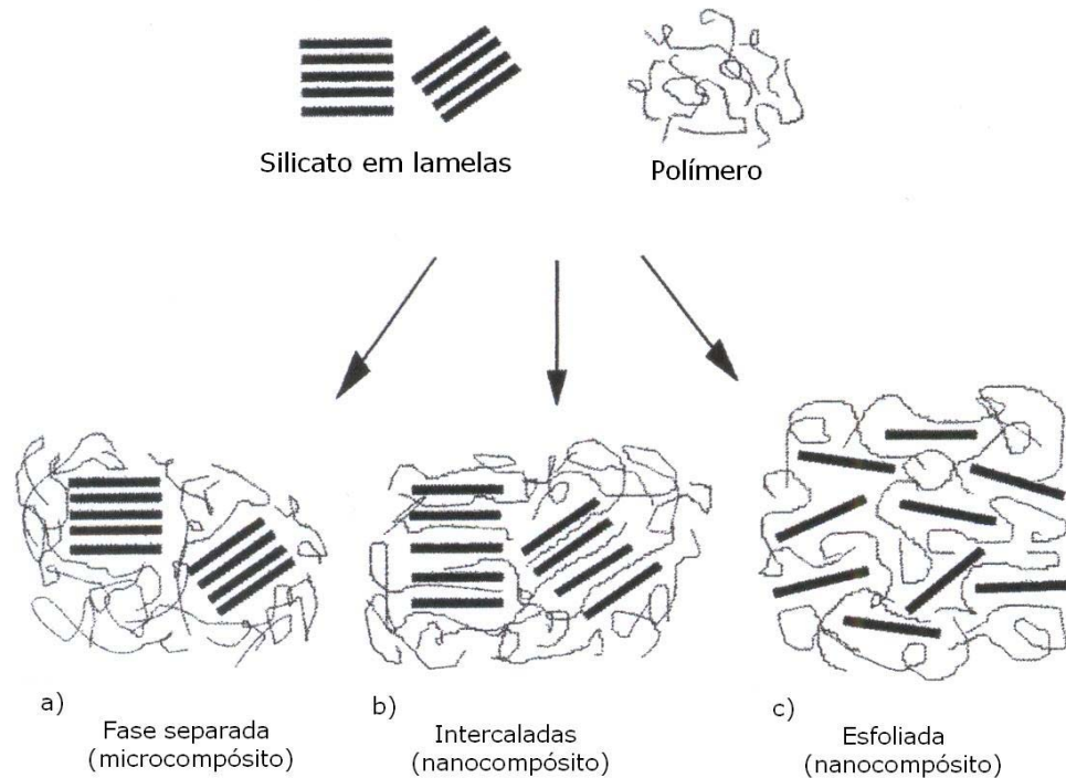
FIGURA 2. 7. Esquema de tipos diferentes de combinação da interação de silicatos em lamelas e um polímero: (a) fase separada - microcompósito (b) intercalada - nanocompósito e (c) esfoliado nanocompósito [7].
