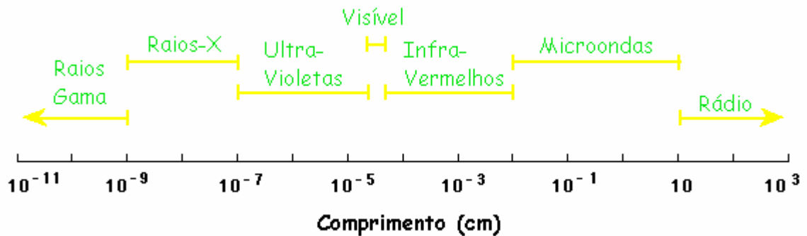
FIGURA 2.1 – ESPECTRO ELETROMAGNÉTICO
