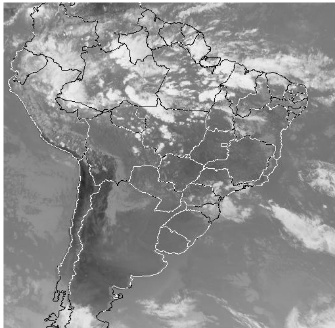
FIGURA 6.9 – IMAGEM DO SATELITE GOES-8 03/04/02 AS 15h09
