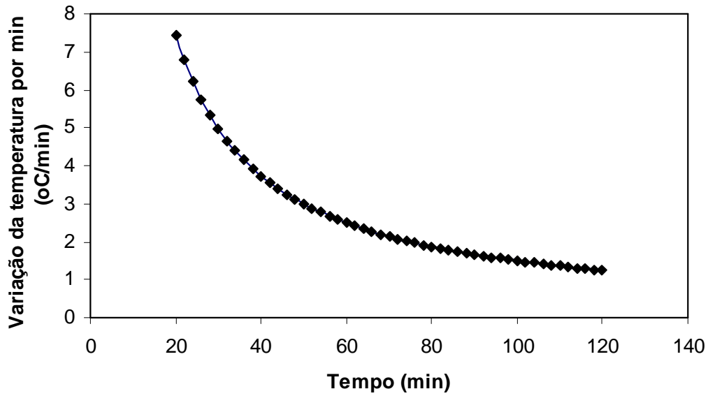
Figura 7: Gradiente temperatura-tempo da curva do incêndio-padrão.
