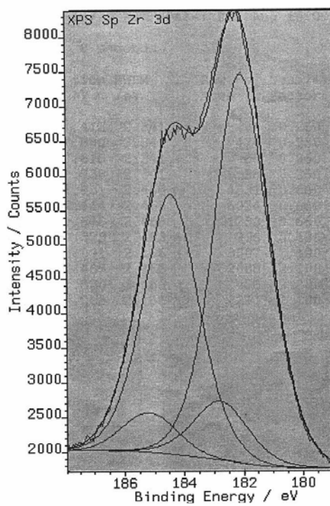
Figura Al.4: Espectro de XPS para alumina B recoberta com 30% (m/m) de ZrO_2 .
