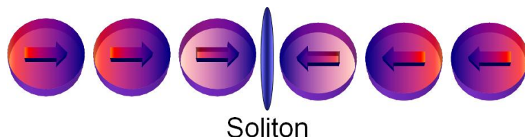
Figura 4.8: Movimento do soliton na estrutura. Análogo à parede de domínio.
