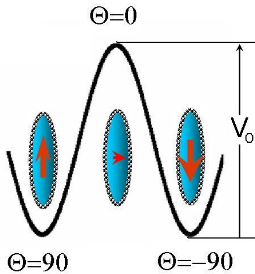
Figura 2.4: Figura mostrando os mínimos de energia magnetostática para \Theta = \pm 90 e máximo em \Theta = 0 . Os estados \Theta = \pm 90 estão separados por uma barreira de energia potencial V_0 que corresponde a altura dela
