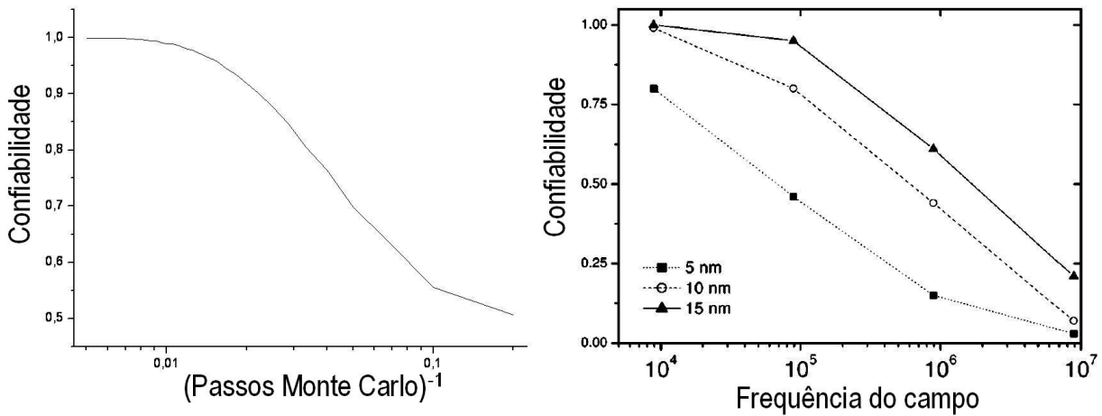
Figura 5.14: O gráfico de Média Confiabilidade por (\text{Número de passos Monte Carlo})^{-1} . O gráfico a esquerda é o resultado de nossas simulações. Direita mostramos um resultado encontrado na literatura (8).
