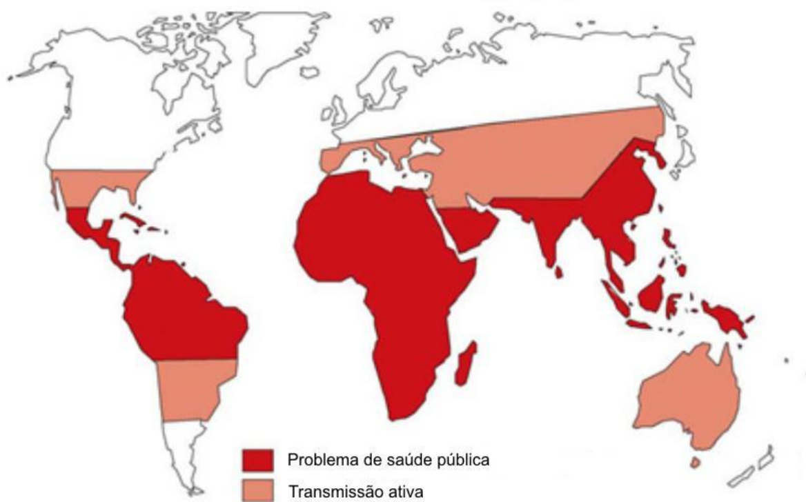
Figura 03: Distribuição mundial das enteroparasitoses transmitidas pelo contato com o solo. (Adaptado de http://www.who.int/intestinal_worms/epidemiology/map/en/index.html )
