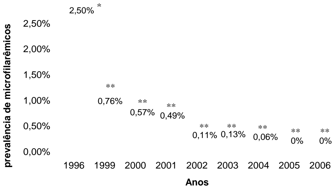
Figura 27: Redução da prevalência de microfilarêmicos em área endêmica de filariose linfática em Maceió e área circunvizinha à área endêmica desde a implantação do Programa de Eliminação da filariose linfática em Maceió-Alagoas (* Rocha et al. , 2000a; **Lima, 2007).
