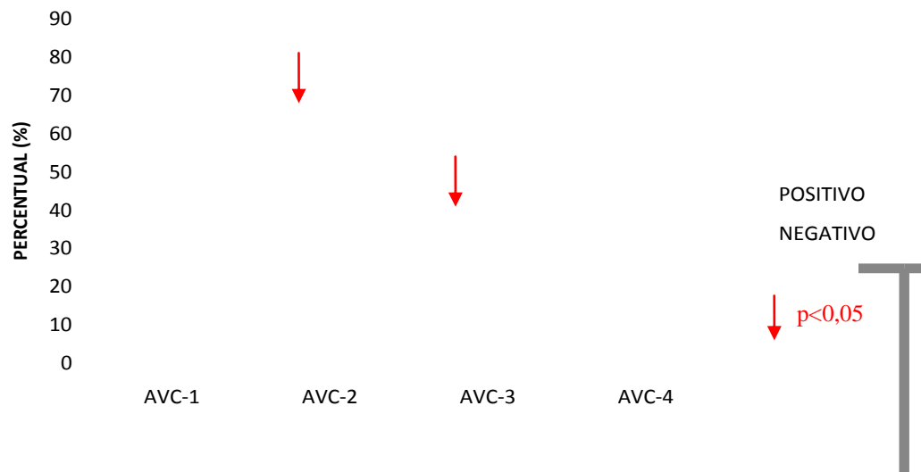
Figura 12: Frequência de indivíduos portadores de enteroparasitoses e/ou esquistossomose mansônica, identificados pelo método de Lutz, na avaliação 1 (AVC-1), avaliação 2 (AVC-2), avaliação 3 (AVC-3) e avaliação 4 (AVC-4) na sub-área controle de filariose linfática em Maceió – Alagoas.
