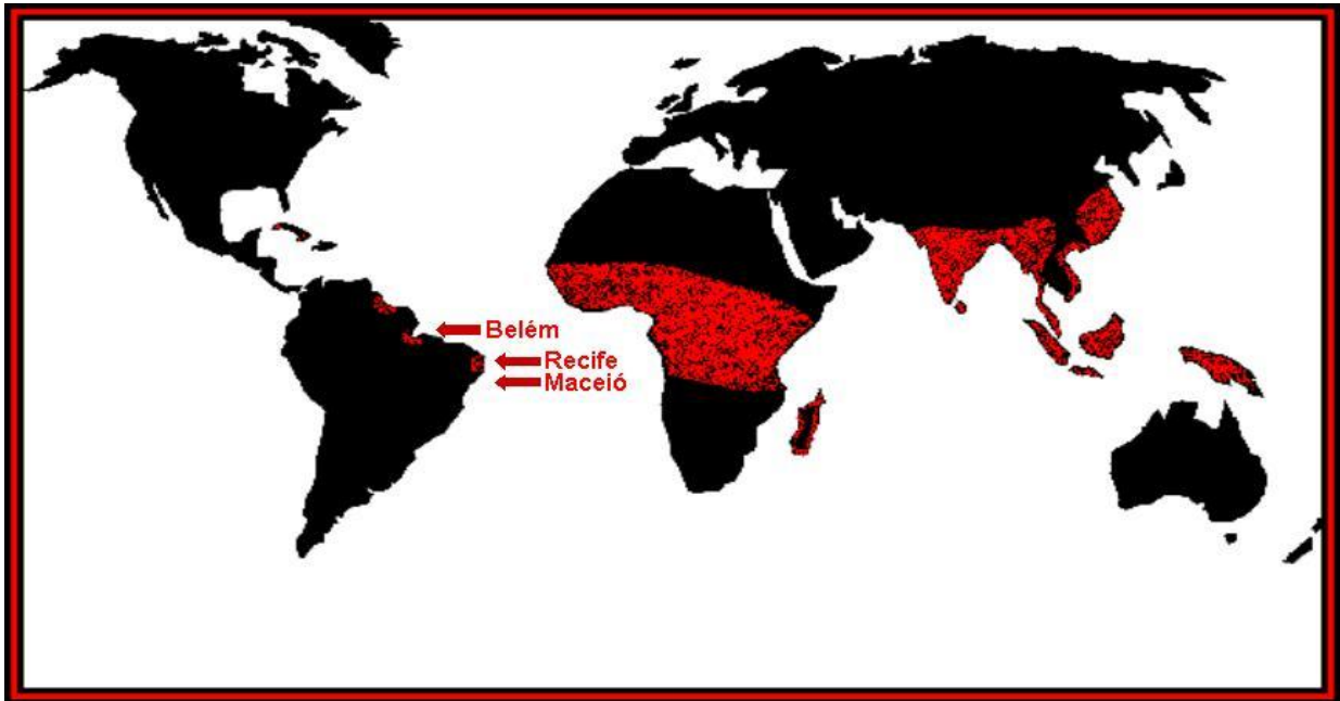
Figura 1: Distribuição mundial das áreas de risco para a filariose linfática. As setas mostram as localidades do Brasil onde a doença é encontrada ou está sob vigilância com transmissão sob controle.
