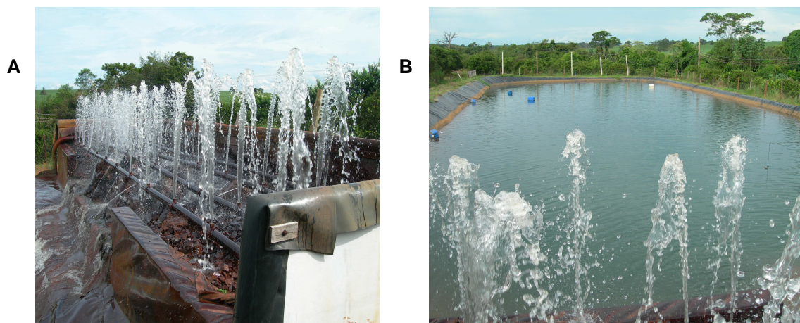
Figura 4. Fotografias do sistema de aerção (A) e do tanque de decantação (B) em momento de limpeza (sem tela de sombreamento).
