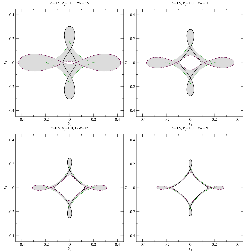
Figura 2.10: Forma da região L/W > C , no plano das fontes, para \kappa_s = 1.0 e e = 0.5 em diferentes valores de C . A linha pontilhada é a cáustica tangencial e as contínua e tracejada são L/W = C .
