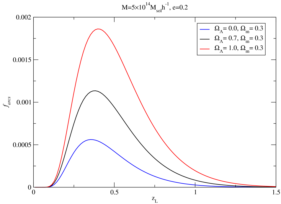
Figura 3.7: Fração de arcos para \Omega_{\Lambda} = 0, 0.7 e 1.0 , o que corresponde à curvatura do universo negativa, nula e positiva respectivamente.
