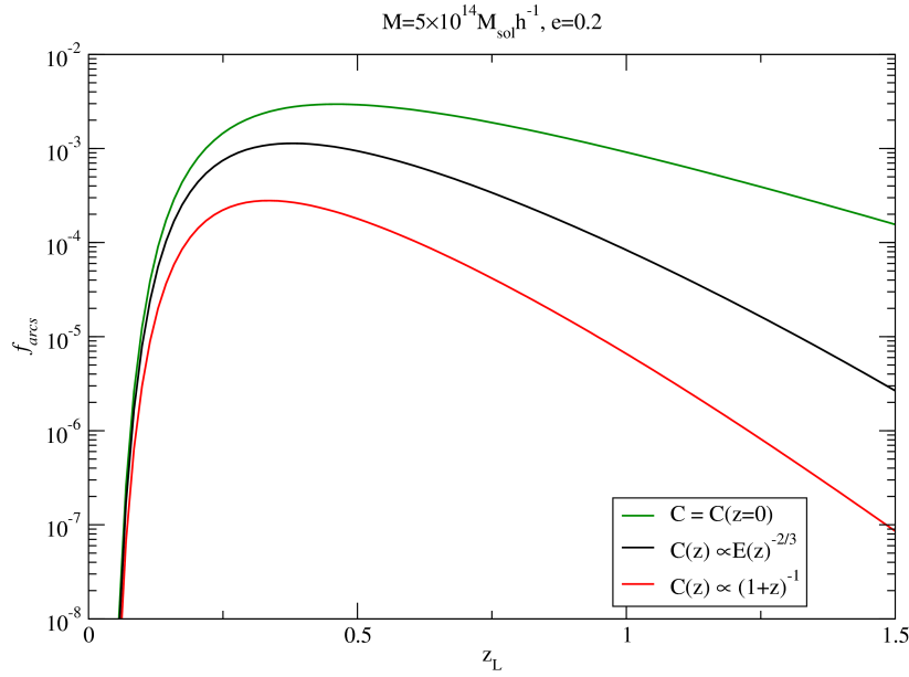
Figura 3.3: Cálculo da fração de arcos para os dois escalonamentos para C(z) (equações 3.23 e 3.22) e para C(z) = C(z = 0) .
