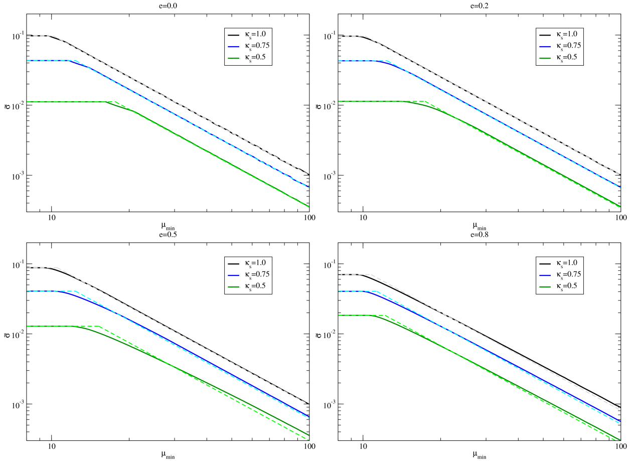
Figura 2.9: Comportamento da seção de choque em relação a \mu_{\min} , para diferentes valores de e e \kappa_s . As linhas contínuas representam o valor exato da seção de choque e as linhas pontilhadas a aproximação dada pela equação (2.34).
