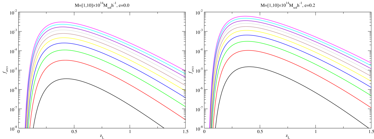
Figura 3.5: Fração de arcos em função do desvio para o vermelho da lente para valores de massa entre 1 \times 10^{14} M_{\odot} h^{-1} e 10 \times 10^{14} M_{\odot} h^{-1} .
