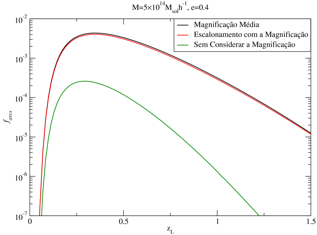
Figura 3.1: Comparação entre as três formas de calcular a seção de choque, para o modelo \Lambda CDM plano e C = 3 .
