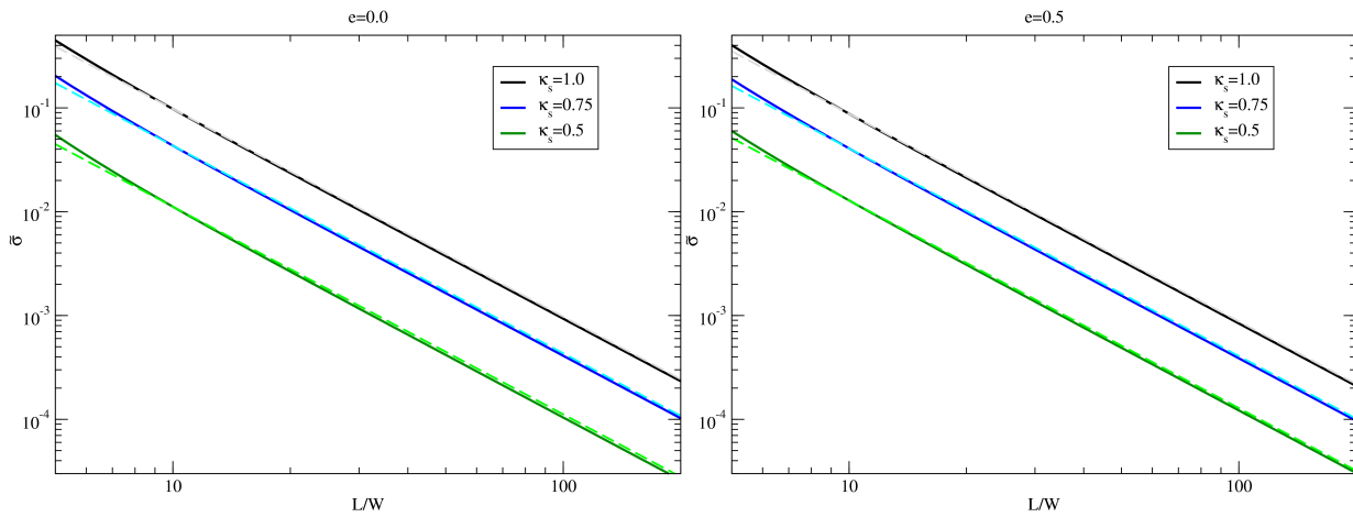
Figura 2.11: Comportamento da seção de choque em relação a R , para diferentes valores de elipticidade e \kappa_s . As linhas contínuas representam o valor exato da seção de choque e as linhas pontilhadas a aproximação dada pela equação (2.40).
