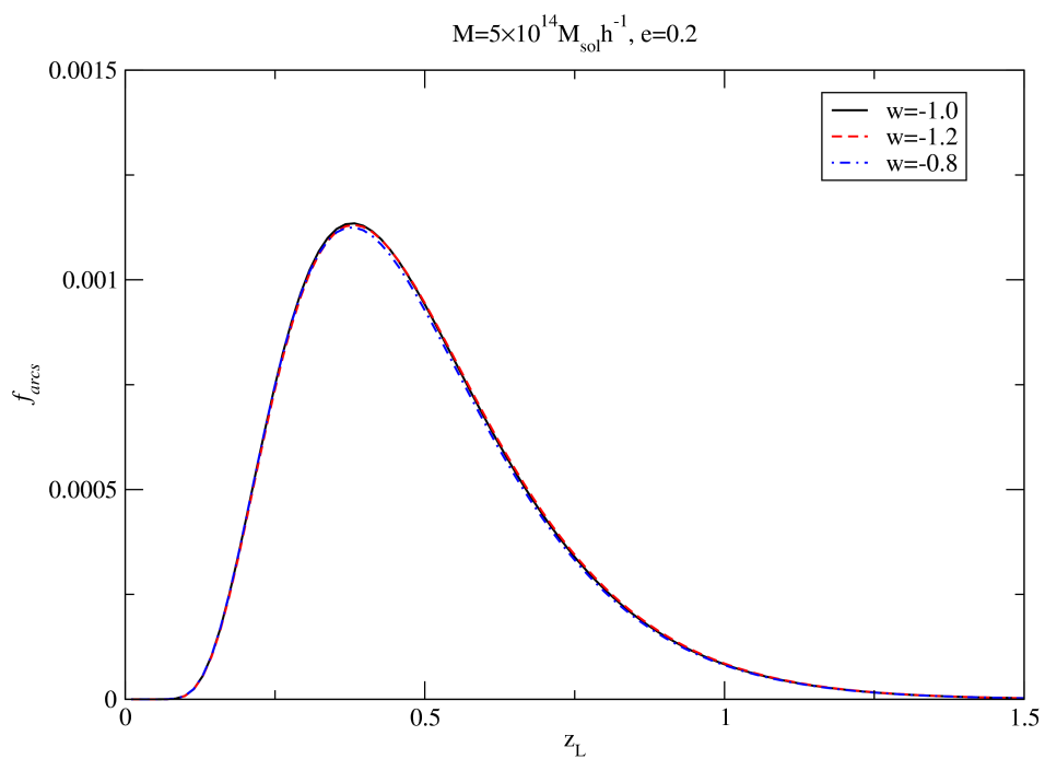
Figura 3.8: Fração de arcos considerando para um fluido com equação de estado p = w\rho , onde estão ilustrados os casos w = -1.2, 1.0 e 0.8
