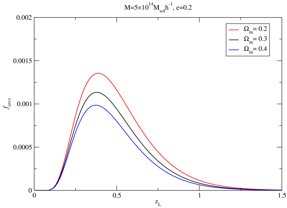
Figura 3.6: Fração de arcos para diferentes valores de \Omega_{0m} em um universo plano para aglomerados com elipticidade 0.2.
