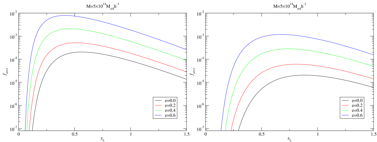
Figura 3.2: Cálculo da fração de arcos feito através da aproximação por \mu_{\text{med}} para duas diferentes definições de massa e alguns valores de elipticidade ( e ). Na figura da esquerda foi utilizada a densidade crítica do universo como \rho_{\text{ref}} , já na direita foi utilizada a densidade de massa do universo (para ambas foi considerado \Delta_{200} = 200 e C = 3 ).
