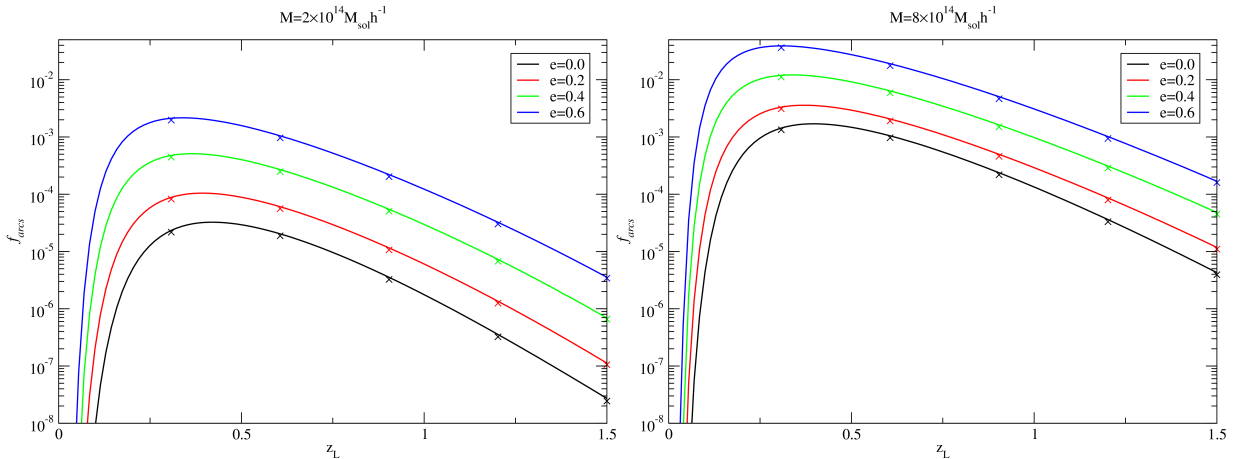
Figura 3.4: Fração de arcos em função do desvio para o vermelho da lente para diferentes valores de massa e elipticidade. Este cálculo foi feito utilizando o modelo \Lambda CDM plano, a parametrização de C(z) dada pela equação (3.23) e a massa definida em uma região cuja densidade média é 200\rho_{\text{crit}} .
