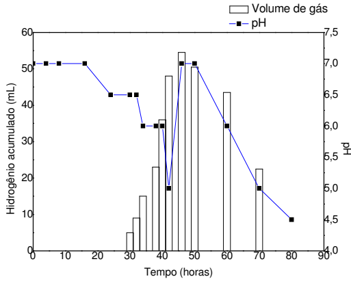
Figura 18: Volume de hidrogênio produzido e acompanhamento da variação do pH durante o cultivo de C. acetobutylicum , realizado com 7,5 gDQO/L de substrato.
