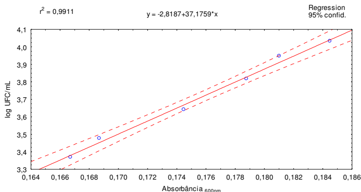
Figura 9: Correlação entre Unidades Formadoras de Colônia (UFC) e Absorvância durante a curva de crescimento de C. acetobutylicum em meio CGM com 0,7% de glicose
