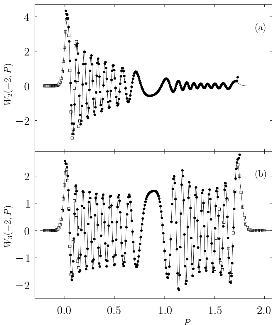
Figura 3.10: Seções da função de Wigner exata (linha contínua) vs WKB (pontos). Na figura (a) são mostradas, para n = 2 , as seções W_n(Q = -2, P) e W_n^{sc}(Q = -2, P) . Em (b) mostramos as mesmas seções para n = 3 . A aproximação adotada, longe das cústicas, coincide ponto a ponto com a solução exata. A aproximação de transição, (3.77), aparece em quadrados e funciona muito bem perto da cústica.
