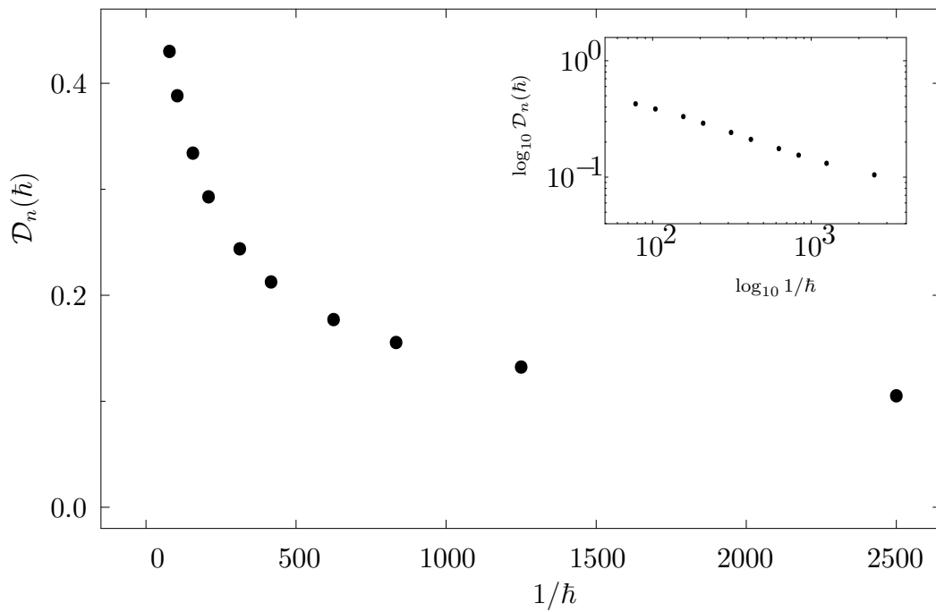
Figura 3.15: A distância média \mathcal{D}_n(\hbar) da AOA como função de 1/\hbar , no instante n = 3 . O gráfico menor, numa escala Log-Log, mostra \log_{10} \mathcal{D}_n(\hbar) vs \log_{10} 1/\hbar . No limite em que \hbar \rightarrow 0 , a distância média entre W_n(X) e W_n^{AOA}(X) diminui.
