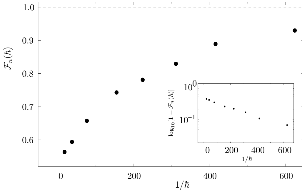
Figura 3.12: Fidelidade \mathcal{F}_n(\hbar) da aproximação semiclassical como função de 1/\hbar , no instante n = 3 . O gráfico menor, numa escala Linear-Log, mostra \log_{10}[1 - \mathcal{F}_n(\hbar)] vs 1/\hbar . Portanto, na medida em que \hbar \rightarrow 0 , a fidelidade tende exponencialmente ao seu valor máximo.
