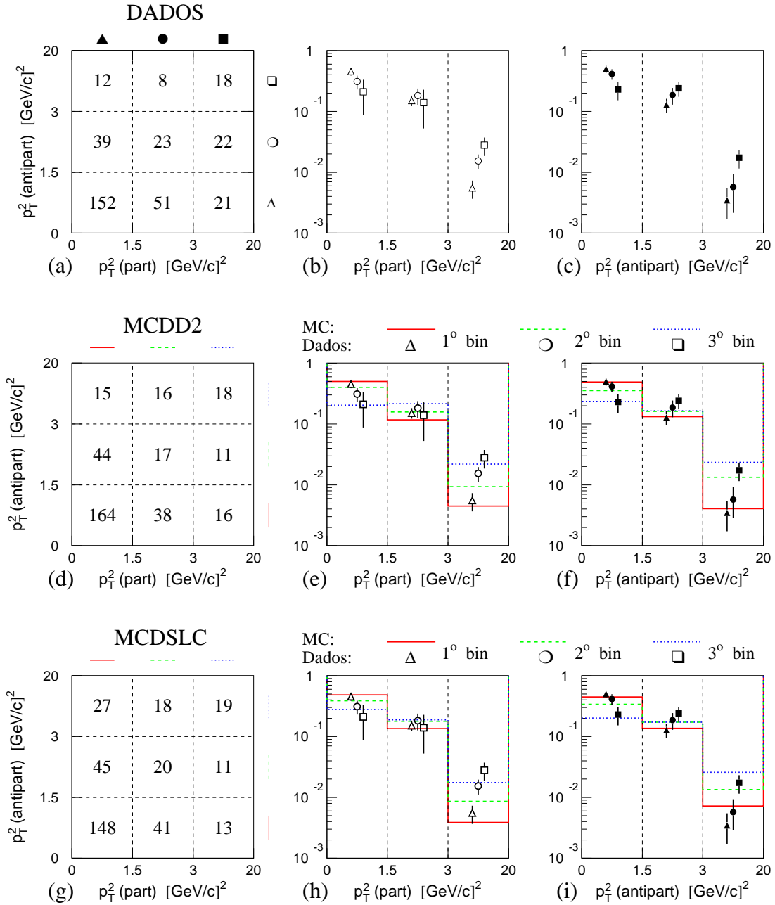
Figura 6.19: Número dN_s de eventos ( D\Lambda_c^- + \Lambda_c^+ \bar{D} ), para os dados (a), e para as amostras de Monte Carlo MCDD2 (d) e MCDSL C (g), distribuídos em nove bins ( p_{T(part)}^2, p_{T(antipart)}^2 ), onde as distribuições de MC estão normalizados com o número de eventos dos dados. (b), (e) e (h) Distribuições normalizadas de p_{T(part)}^2 , 1/N_i[dN_s/dp_{T(part)}^2] , para cada bin de p_{T(antipart)}^2 , correspondentes aos dados e às amostras de MC. As distribuições de MC comparados com os dados. (c), (f) e (i) Similar a (b), (e) e (h) para as distribuições de p_{T(antipart)}^2 .
