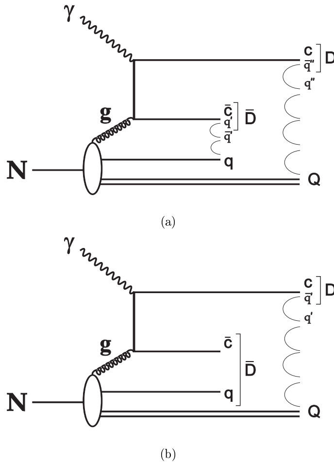
Figura 6.23: Produção dos pares D\bar{D} : (a) a energias típicas dos experimentos de alvo fixo, (b) a baixas energias, por associação direta de um antiquark \bar{c} e o "quark solteiro" q do núcleo. Em ambos casos se espera que a produção seja simétrica.
