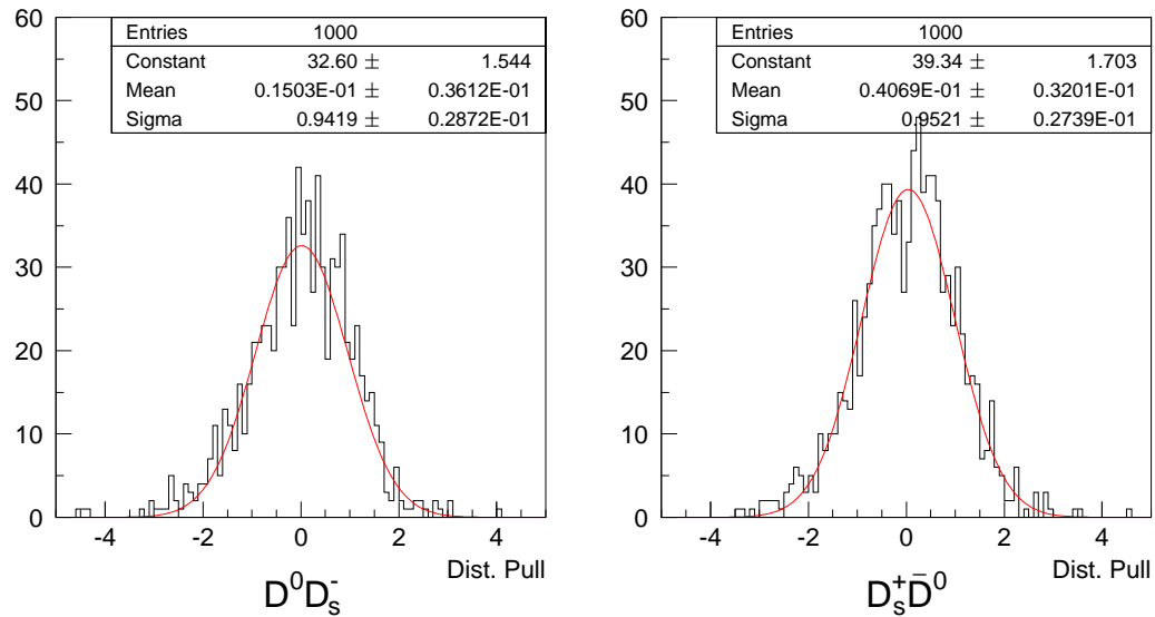
Figura 6.28: Distribuições pull das amostras de pares D^0 D_s^- e D_s^+ \bar{D}^0 .
