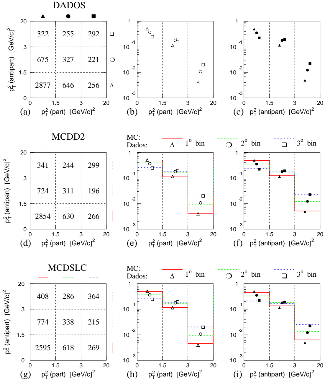
Figura 6.17: Número dN_s de eventos D\bar{D} , para os dados (a), e para as amostras de Monte Carlo MCDD2 (d) e MCDSL C (g), distribuídos em nove bins ( p_{T(part)}^2, p_{T(antipart)}^2 ), onde as distribuições de MC estão normalizadas com o número de eventos dos dados. (b), (e) e (h) Distribuições normalizadas de p_{T(part)}^2 , 1/N_i [dN_s/dp_{T(part)}^2] , para cada bin de p_{T(antipart)}^2 , correspondentes aos dados e às amostras de MC. As distribuições de MC comparados com os dados. (c), (f) e (i) Similar a (b), (e) e (h) para as distribuições de p_{T(antipart)}^2 .
