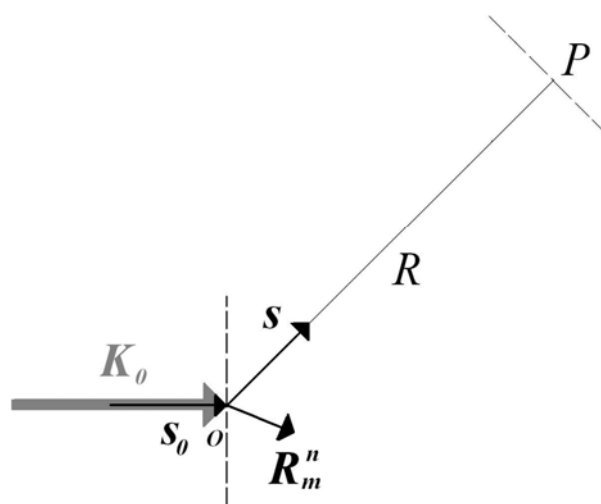
Figura 2.5. Difração de uma onda de vetor de onda K_0 por um pequeno cristal cuja distância ao ponto P é R .
