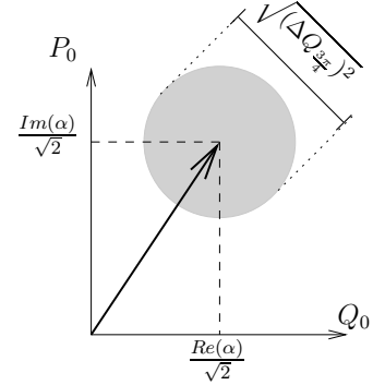
Figura 1.2: Estado coerente
