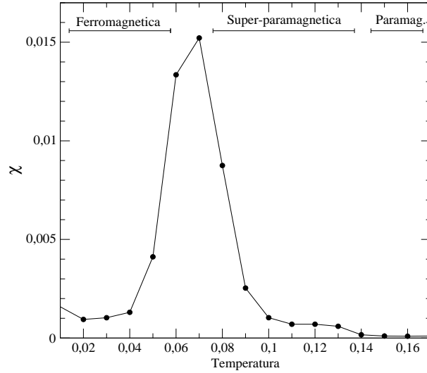
Figura 3.1: Susceptibilidade em função da temperatura do sistema. O pico caracteriza a transição entre o estado ordenado para o estado super-paramagnético. O patamar na susceptibilidade caracteriza os grupos de spins que se fragmentam a altas temperaturas.
