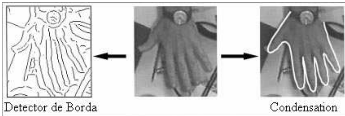
Figura 2.6 – Rastreamento usando o algoritmo Condensation . Trabalho de Isard e Blake [6]
