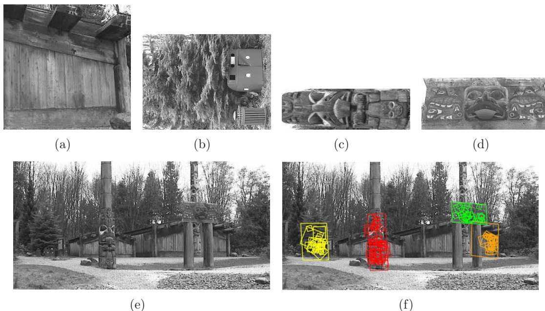
Figura 2.3 – Algoritmo SIFT [3]. As Figuras (a), (b), (c) e (d) são as imagens de treinamento, a Figura (e) é a imagem para o teste. A Figura (f) mostra as regiões reconhecidas, com os pontos chave representados como pequenos retângulos.
