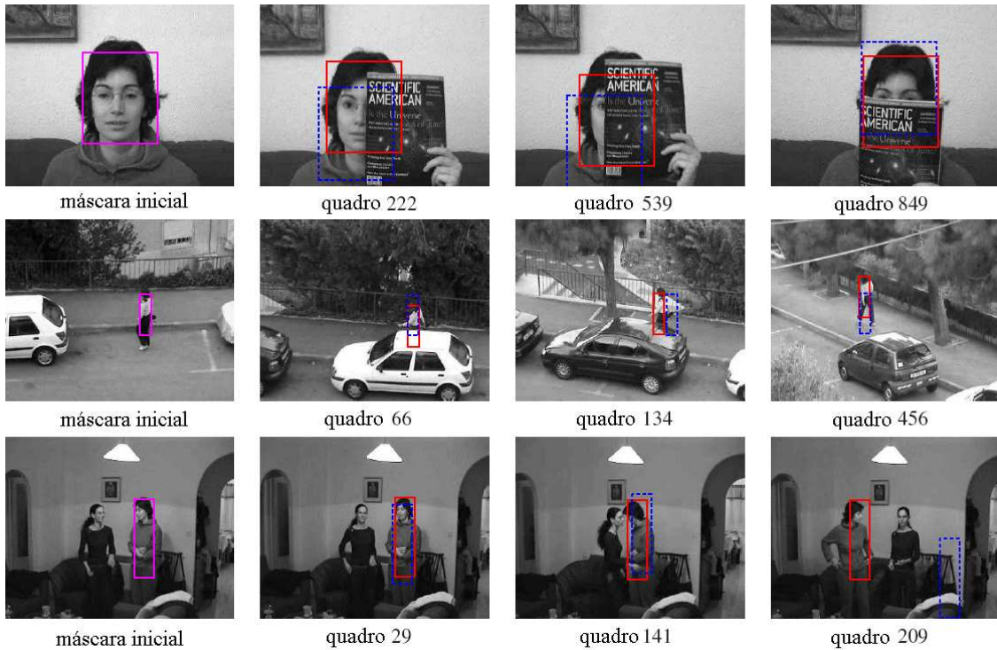
Figura 2.5 – Resultados do algoritmo FragTrack [5] (retângulos em vermelho), comparados com o rastreamento obtido pela técnica Meanshift [4] (representado pelos retângulos pontilhados em azul).
