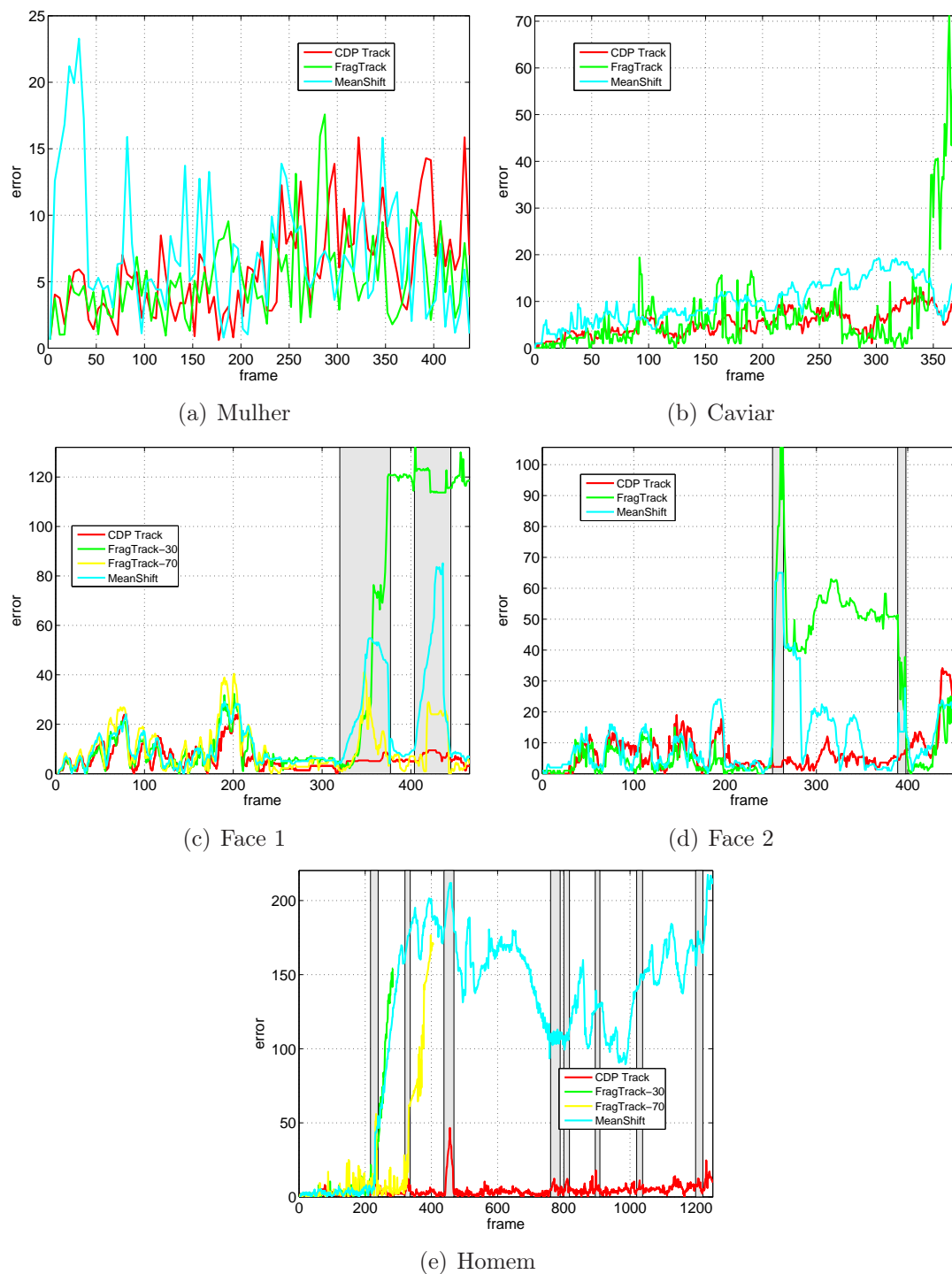
Figura 4.1 – Erro de Rastreamento das técnicas analisadas ( Meanshift , FragTrack e CPD ) para as cinco seqüências de vídeo. Os retângulos cinzas indicam os trechos das seqüências onde ocorre a oclusão total dos alvos.
