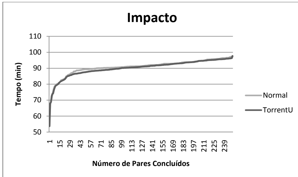
Figura 6.4: Impacto do Monitor no Enxame
