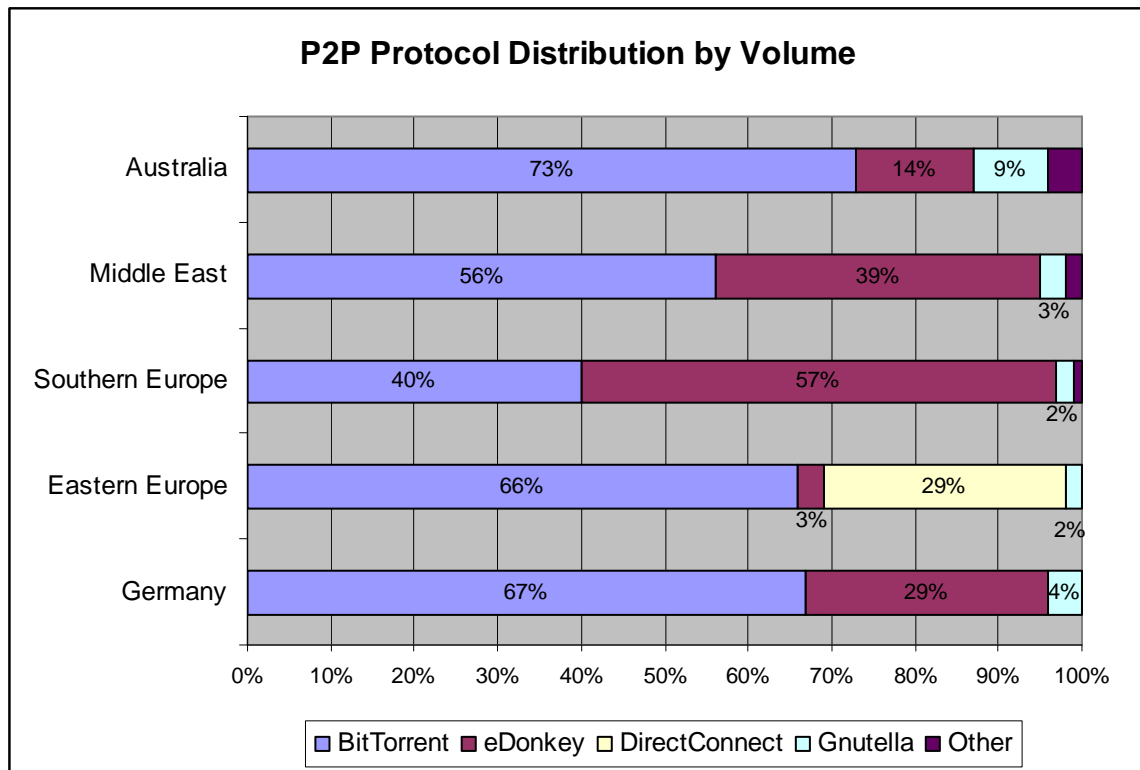
Figura 1.2: Participação de cada protocolo
