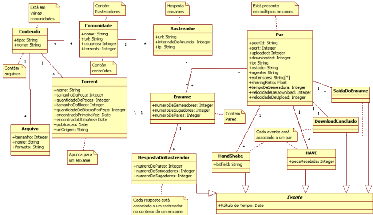
Figura 4.2: Modelo de Dados
