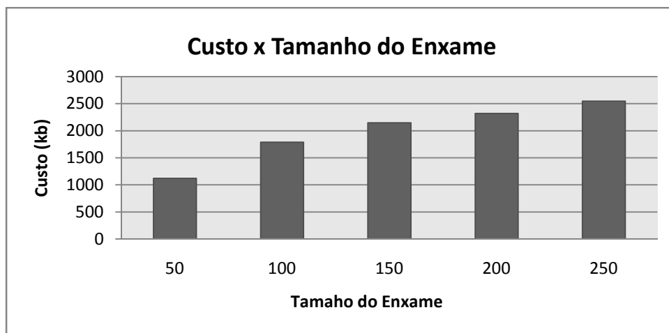
Figura 6.2: Custo do Monitor com Peça de 1MB
