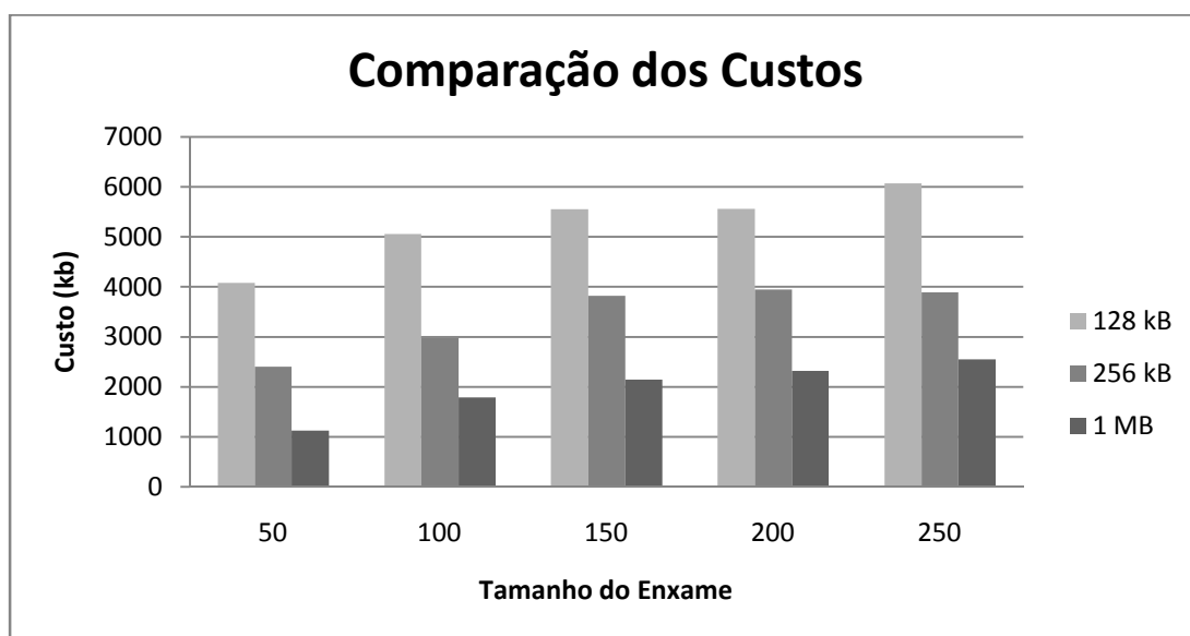
Figura 6.3: Comparação de Custos
