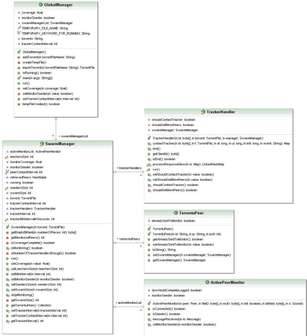
Figura 5.5: UML das Classes
