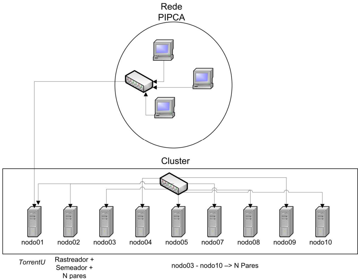
Figura 6.1: Ambiente de Testes
