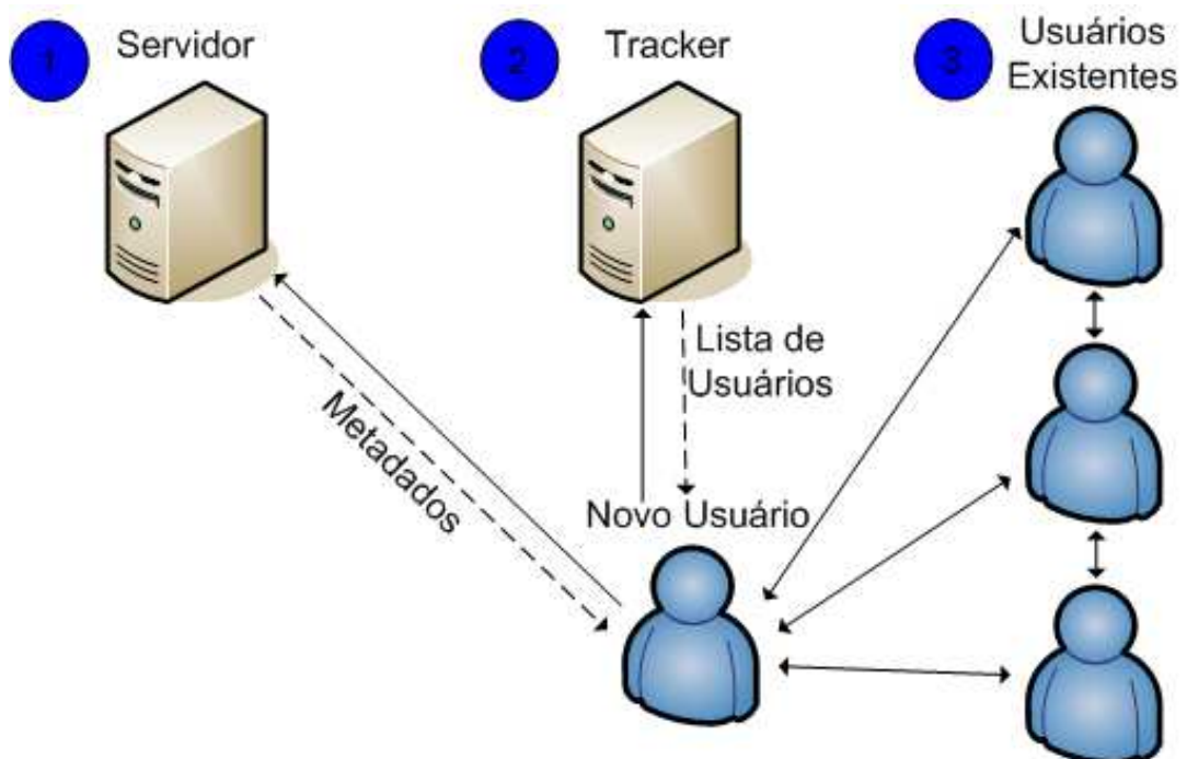
Figura 2.1: Fases do Protocolo BitTorrent
