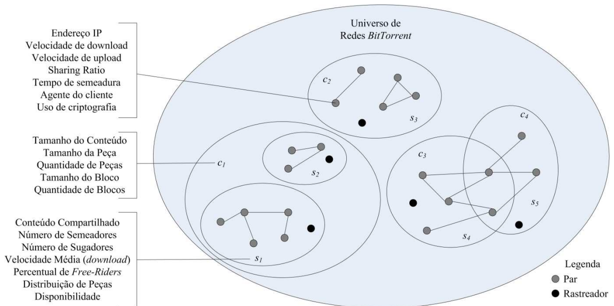
Figura 2.2: Universo Torrent
