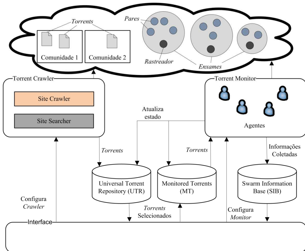
Figura 4.1: Arquitetura TorrentU
